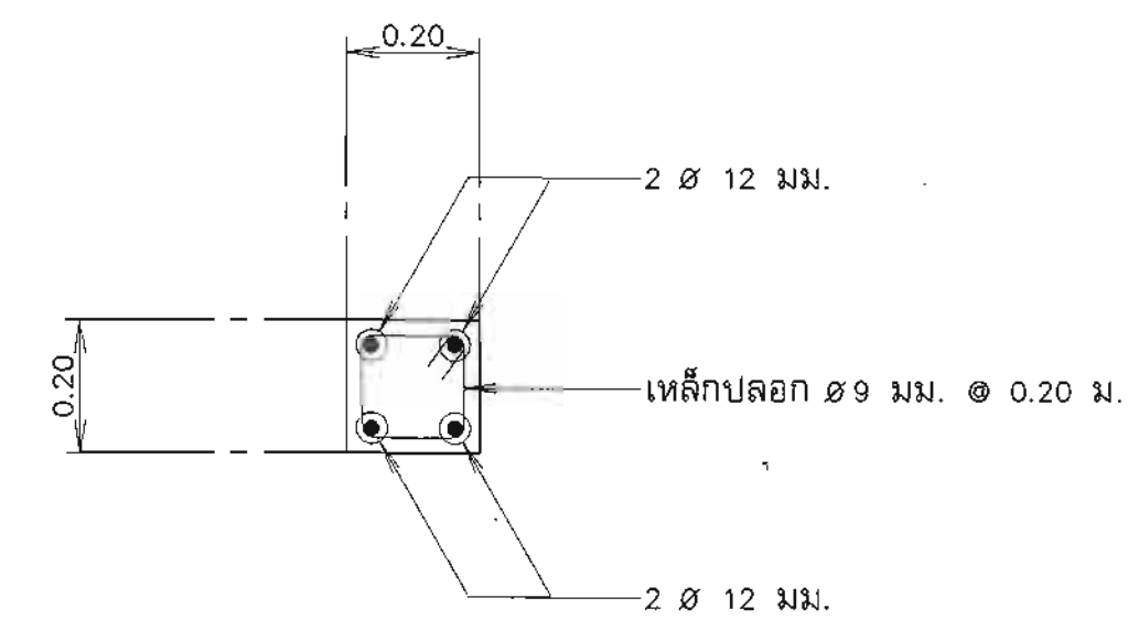
รูปตัด ค - ค มาตราส่วน 1:12.5
