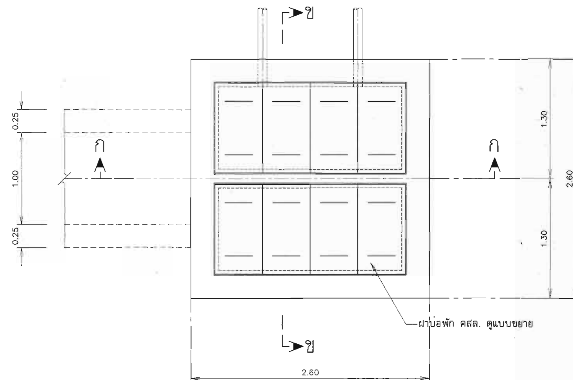
แปลนอาคารบ่อน้ำ มาตราส่วน 1:25
