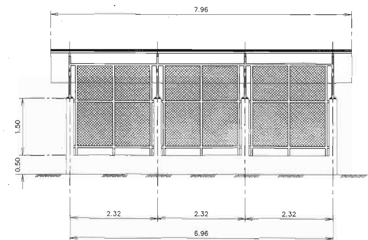
รูปด้านหลังอาคารโรงสูบน้ำ
