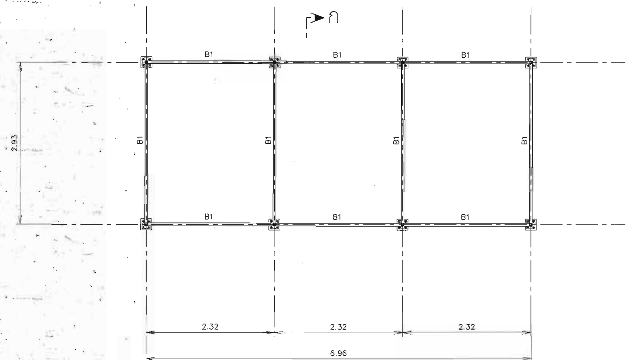
รายละเอียด โครงหลักรับแผงเซลล์แสงอาทิตย์
