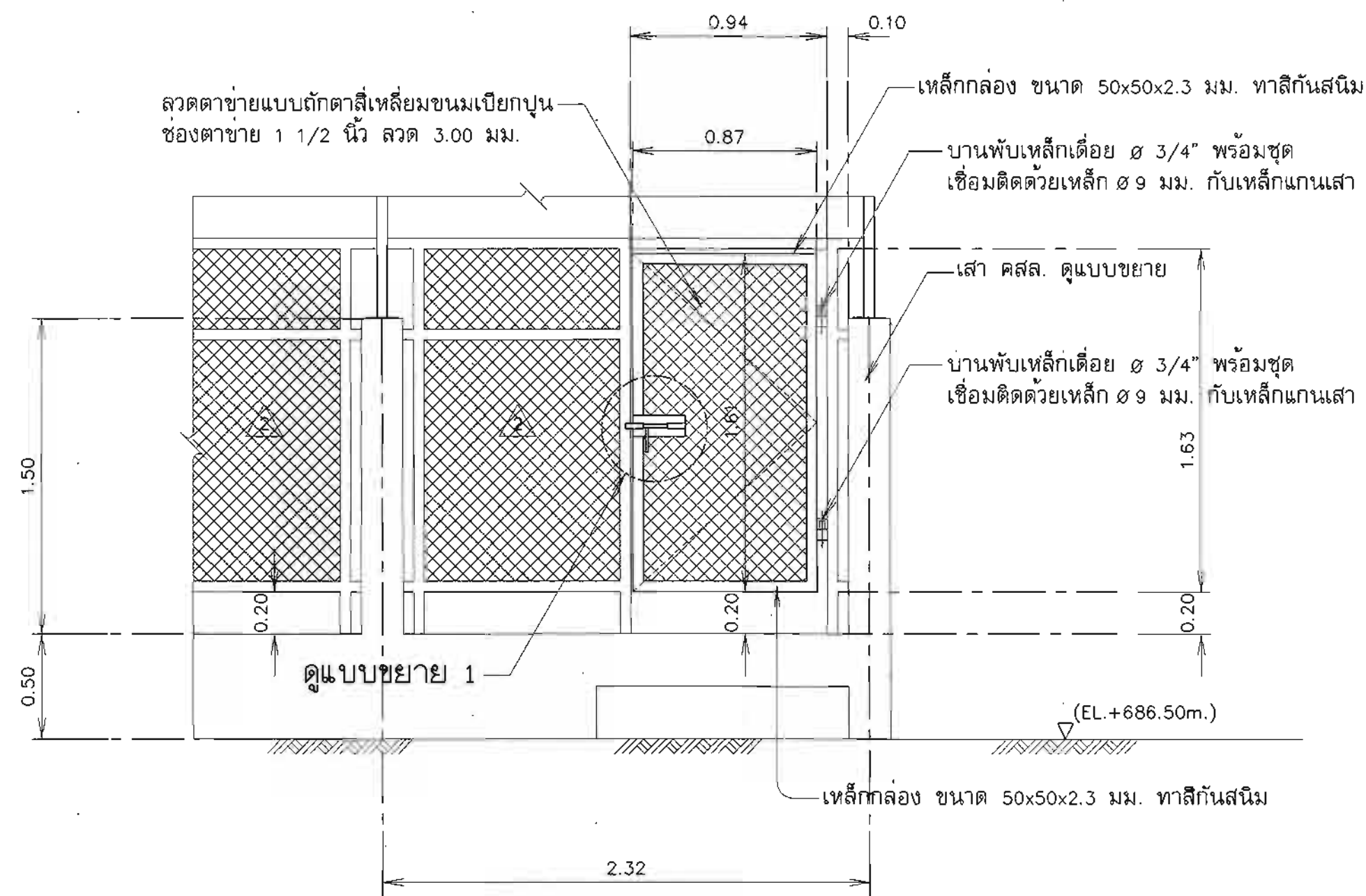
ขยายประตู มาตราส่วน 1:25
