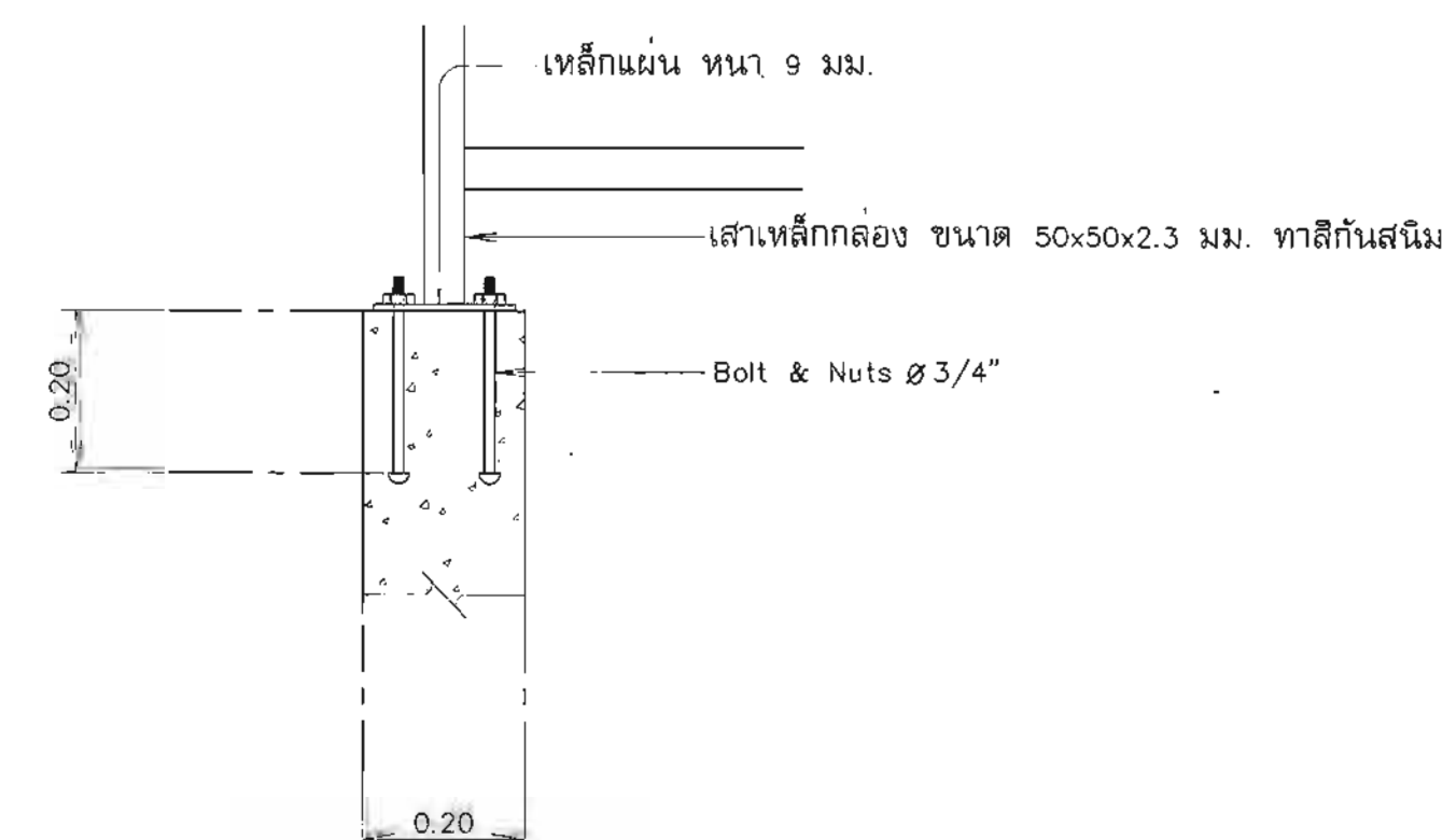
รูปขยาย 1
