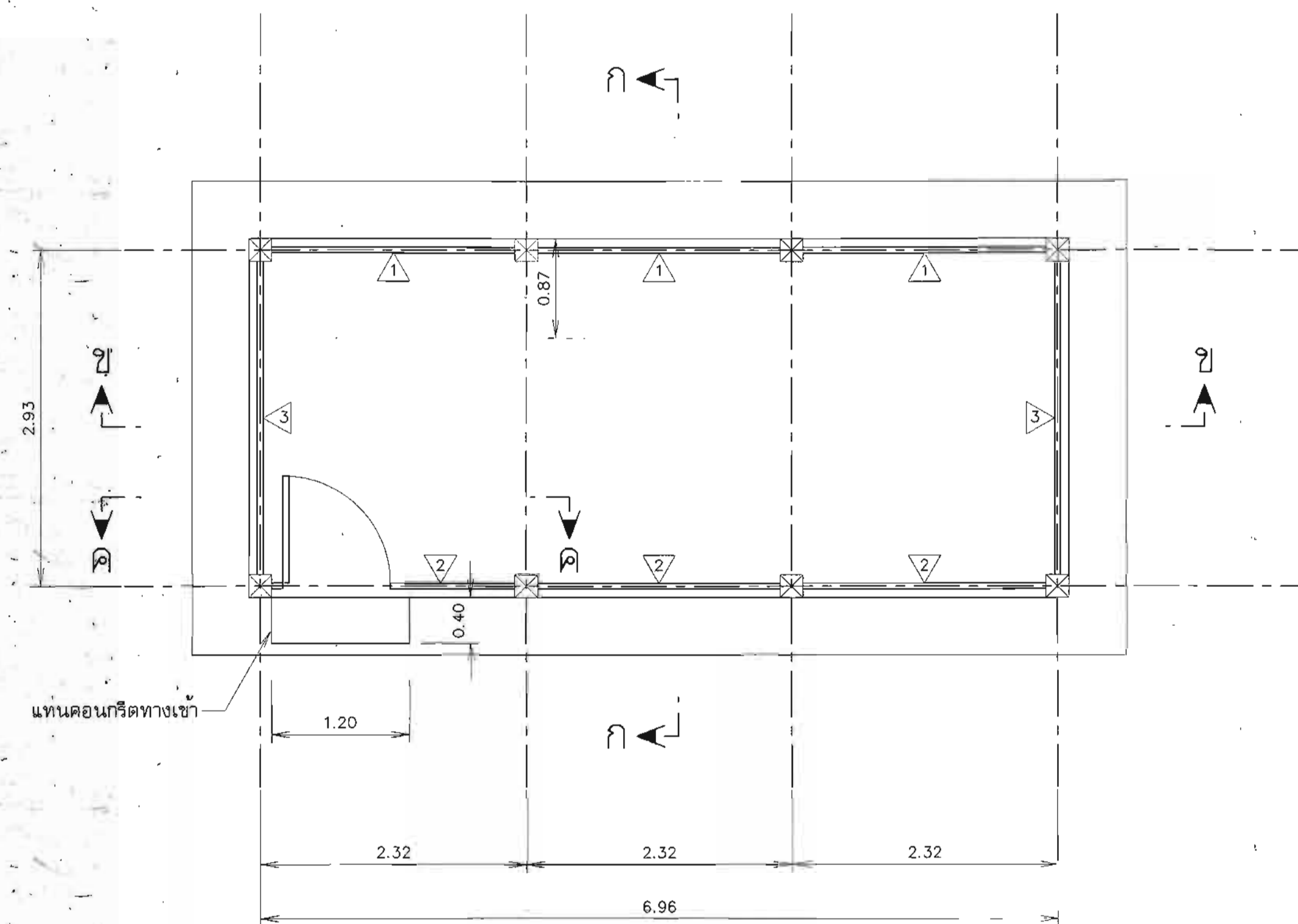
แปลนอาคารโรงสูบน้ำ
