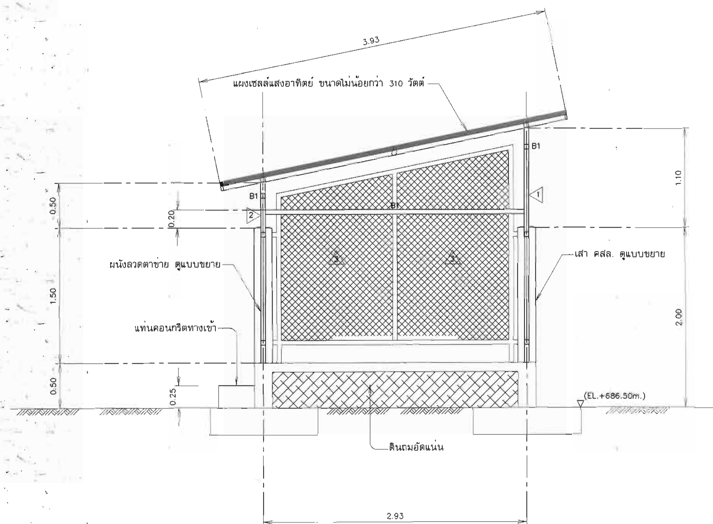
รูปตัด ข - ข
