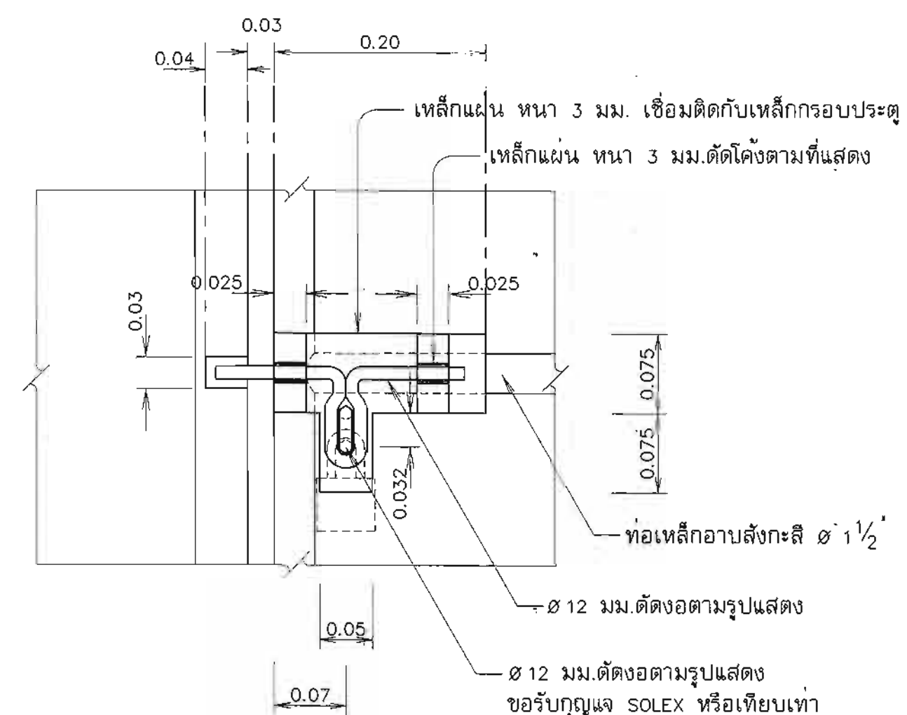
อธิบาย 1 มาตราส่วน 1:5
