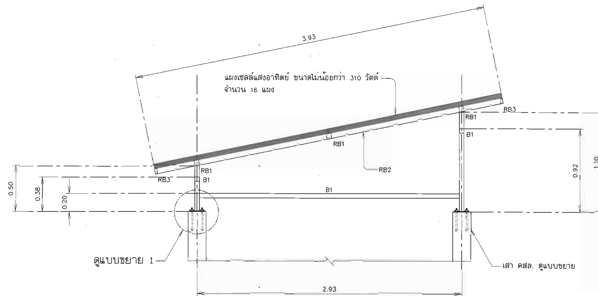
รายละเอียด โครงหลักรับแผงเซลล์แสงอาทิตย์
