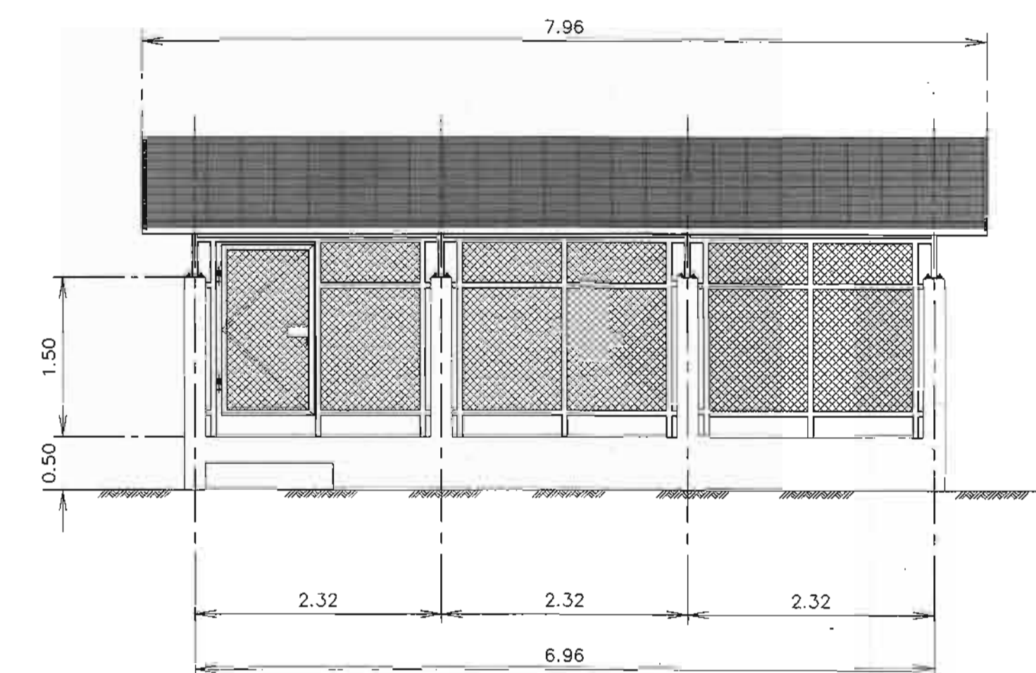
รูปด้านหน้าอาคารโรงสูบน้ำ
