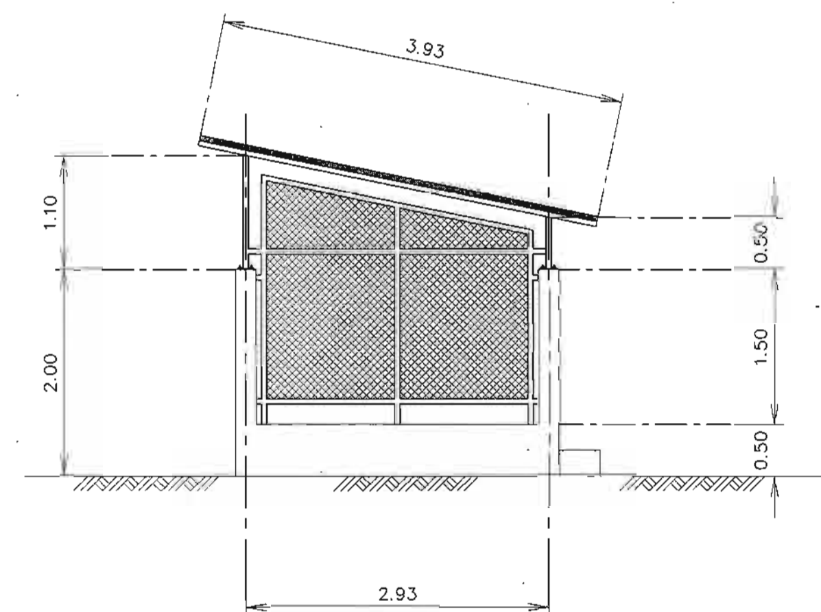
รูปด้านข้างอาคารโรงสูบน้ำ
