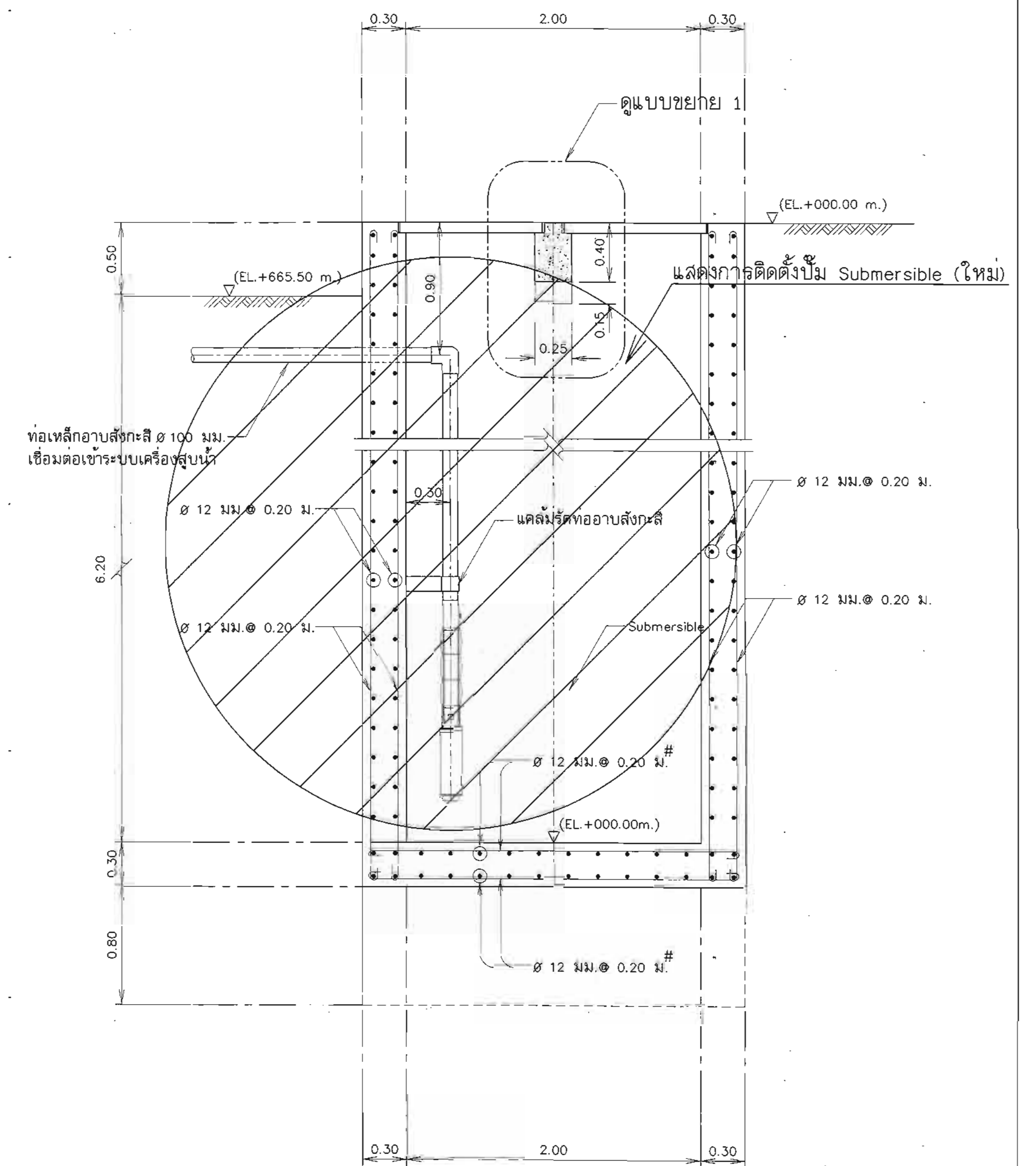
รูปตัด ข - ข อาคารบ่อน้ำ มาตราส่วน 1:25
