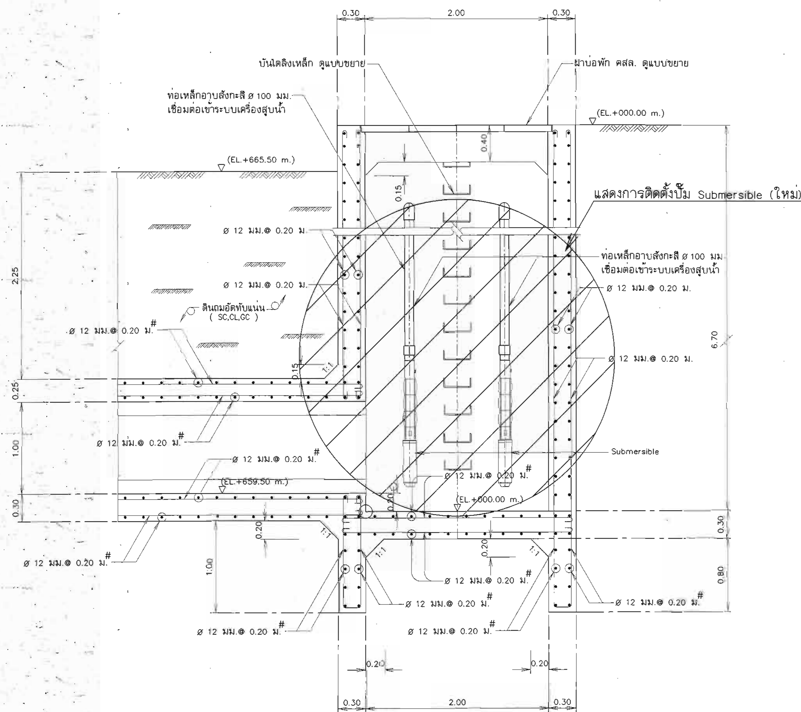
รูปตัด ก - ก อาคารบ่อน้ำ มาตราส่วน 1:25
