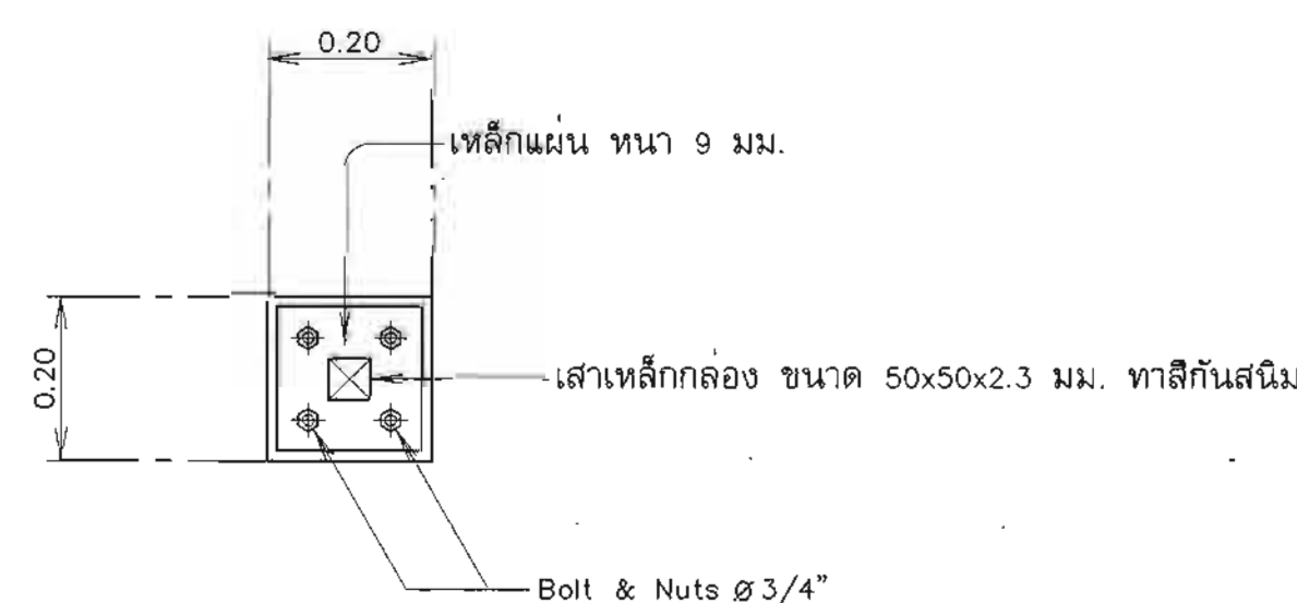
ขยายรอยต่อเสา คสล.-เสาเหล็ก
