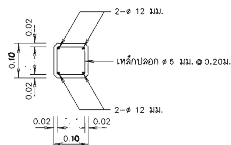
รูปตัด 2 - 2 มาตรฐาน 1:10
