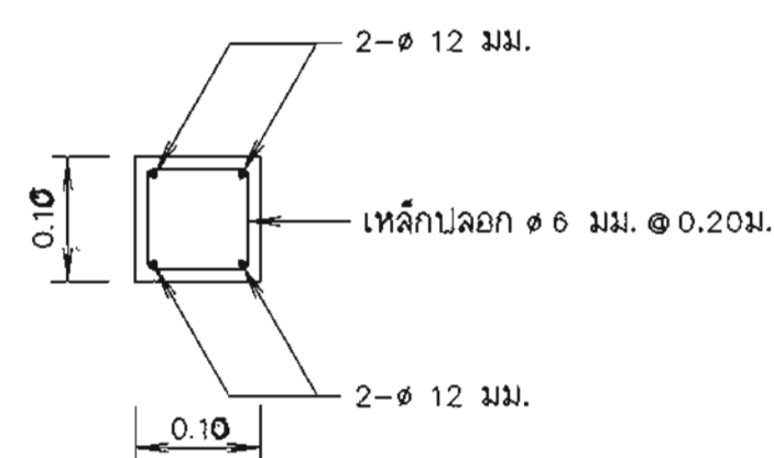
รูปตัด 1 - 1 มาตรฐาน 1:10
