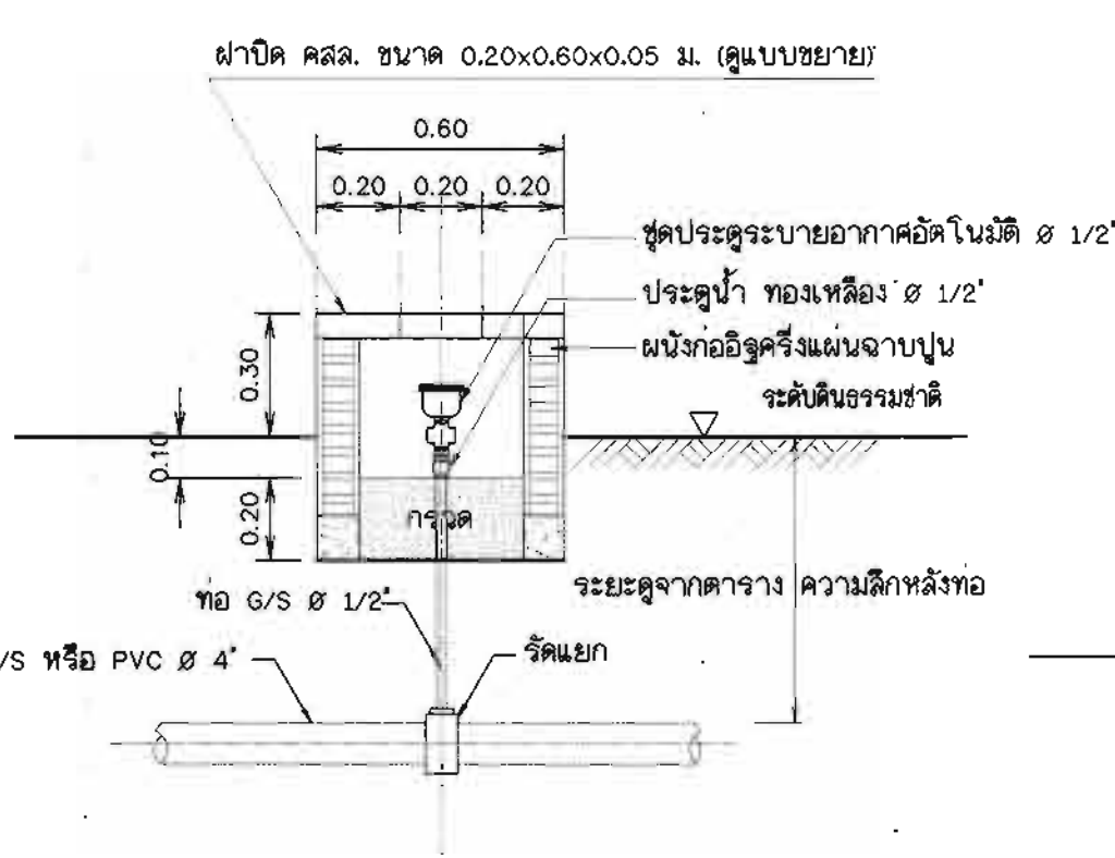
การติดตั้งประตูปะบายอากาศอัตโนมัติ มาตราส่วน 1:20
