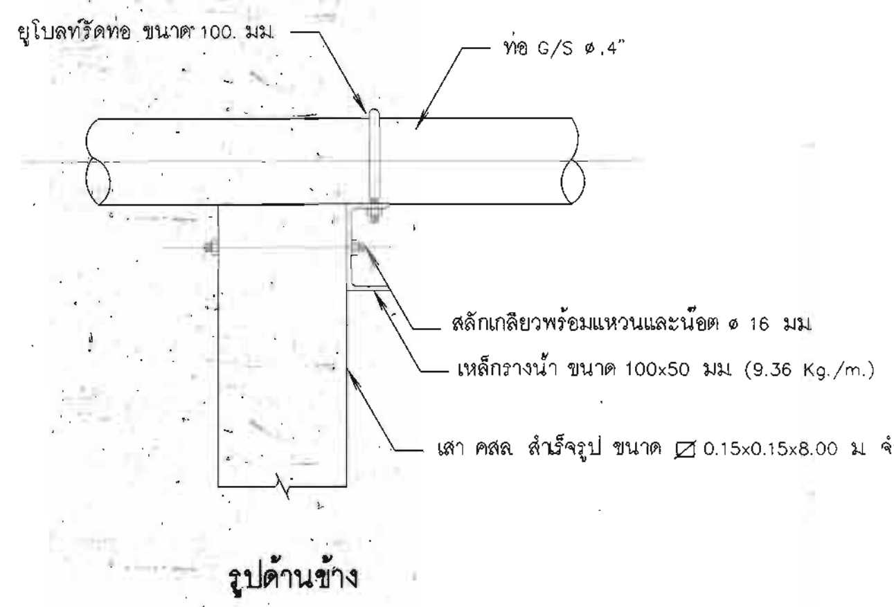
15. การต่อท่อเครื่องสูบน้ำ ไม่แสดงมาตราส่วน
