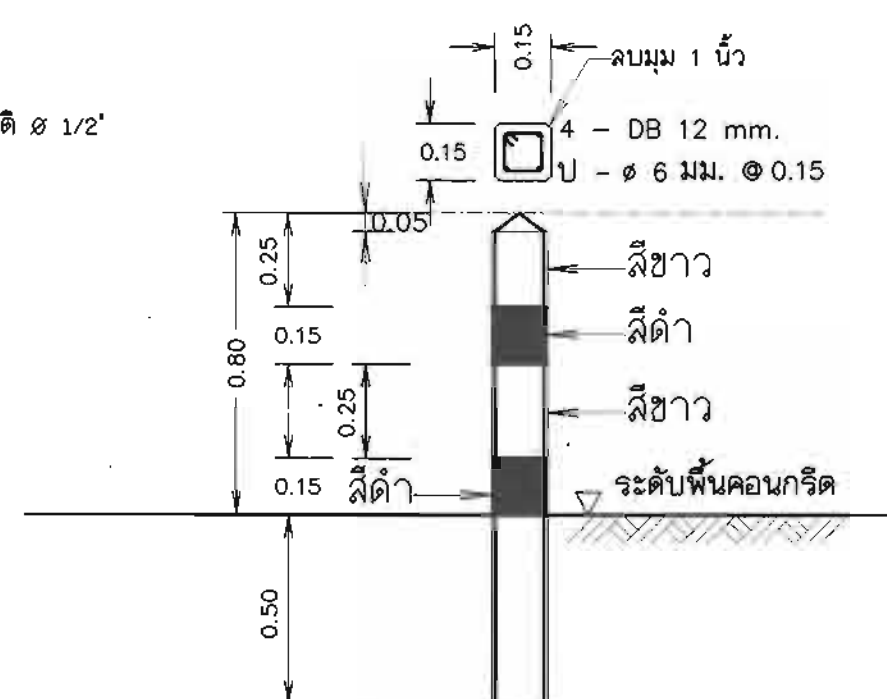
แบบขยาย หลักรัง คสล. มาตราส่วน 1:20
