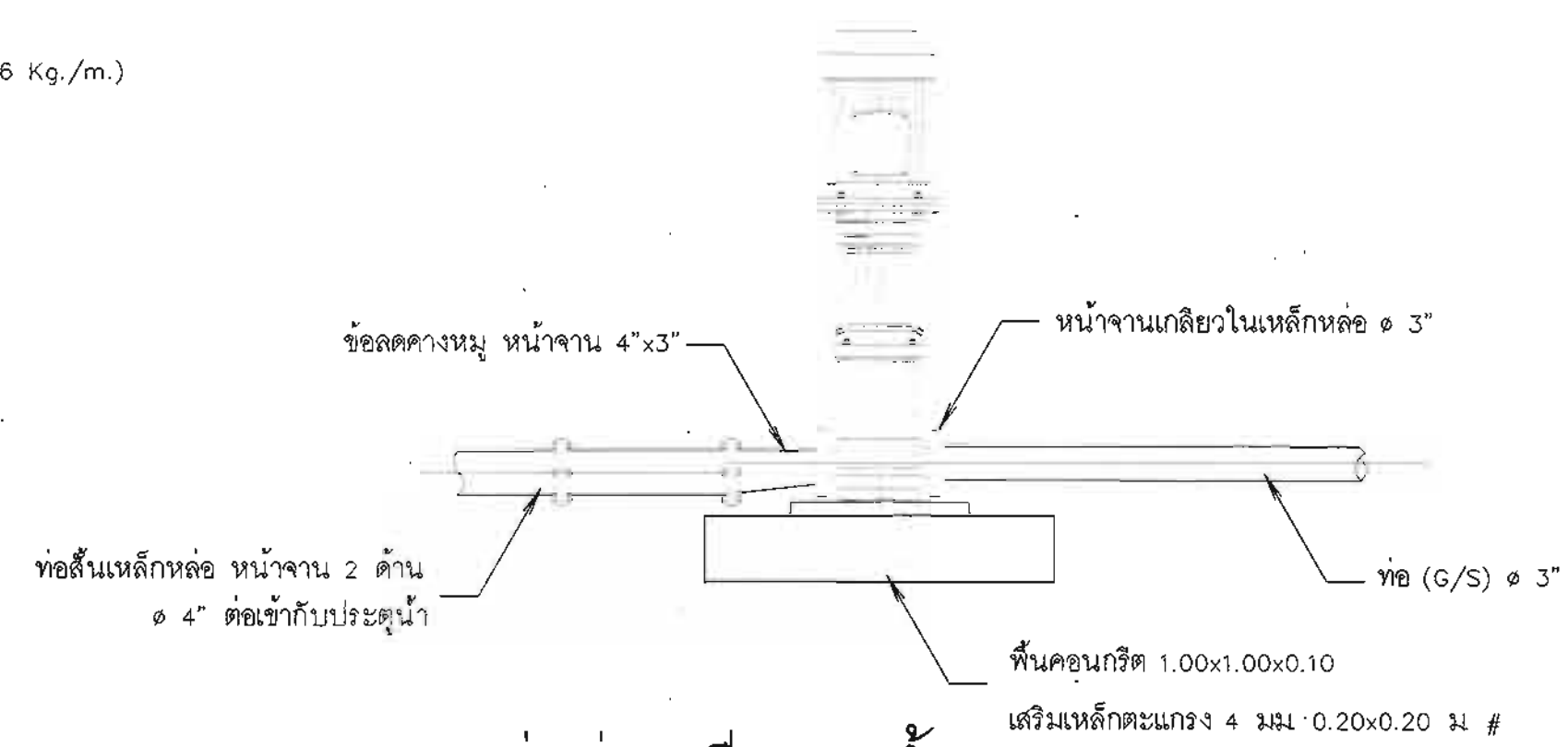
16. การติดตั้งประตูปะบายอากาศอัตโนมัติ ไม่แสดงมาตราส่วน
