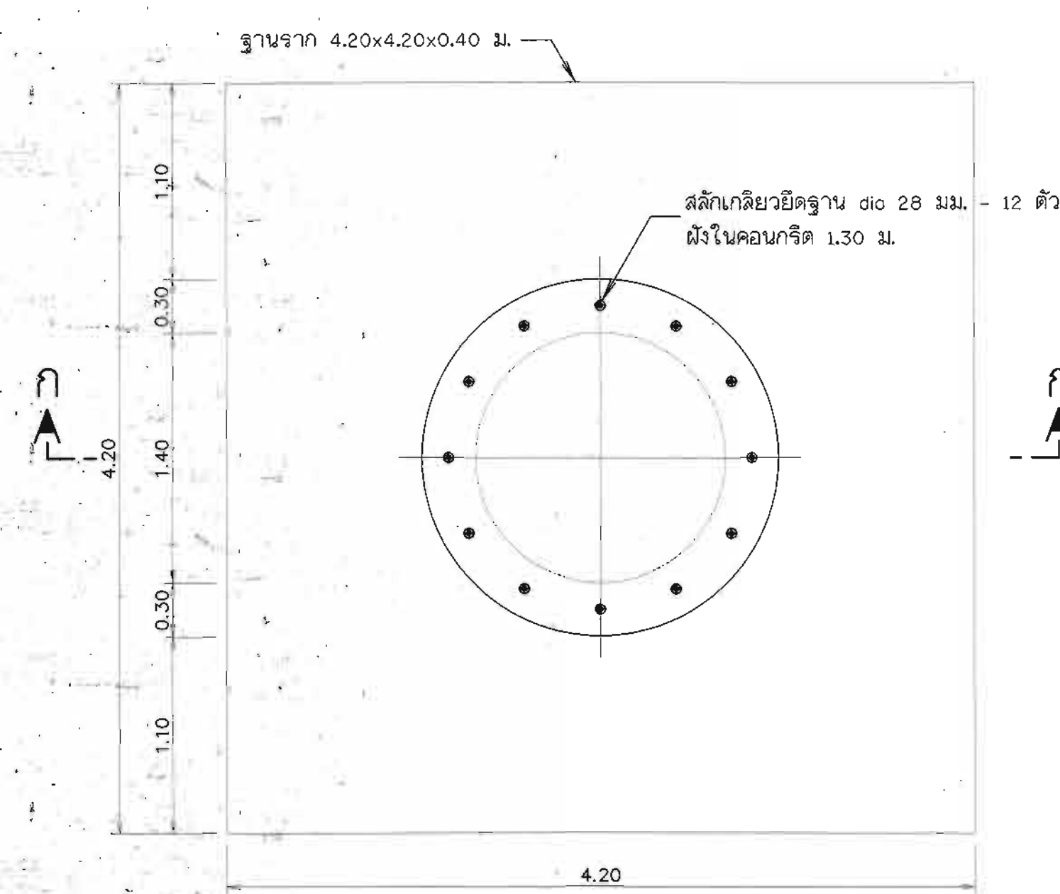
แปลน ฐานรากหอดึงสูง (แบบฐานแฉก)
