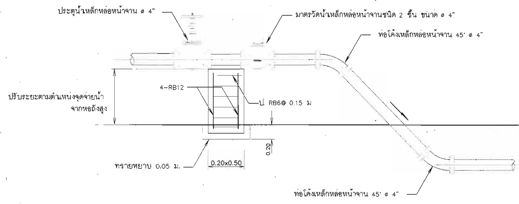
13. เสาคอมม่อนรับท่อชุด และแบบขยายอุปกรณ์รัดท่อ ไม่แสดงมาตราส่วน
