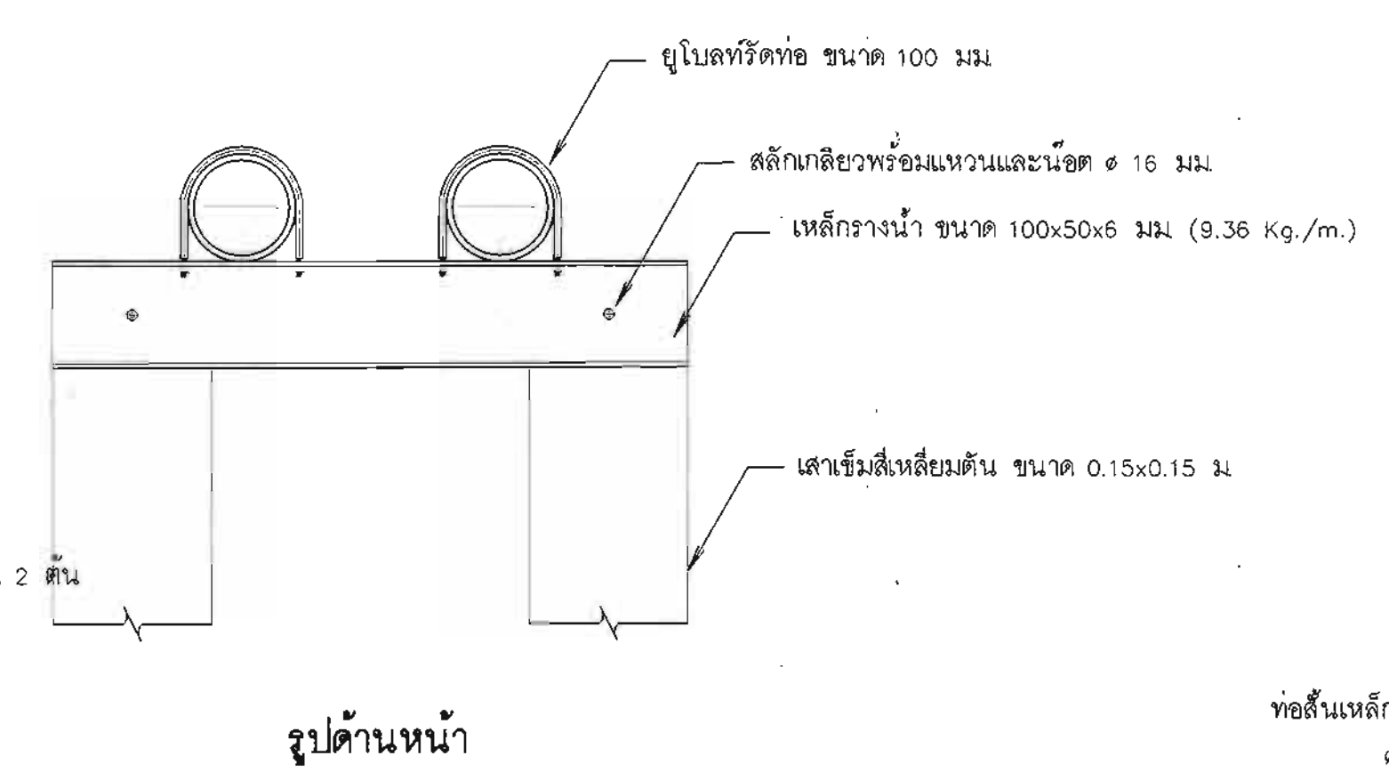
15. การต่อท่อเครื่องสูบน้ำ ไม่แสดงมาตราส่วน
