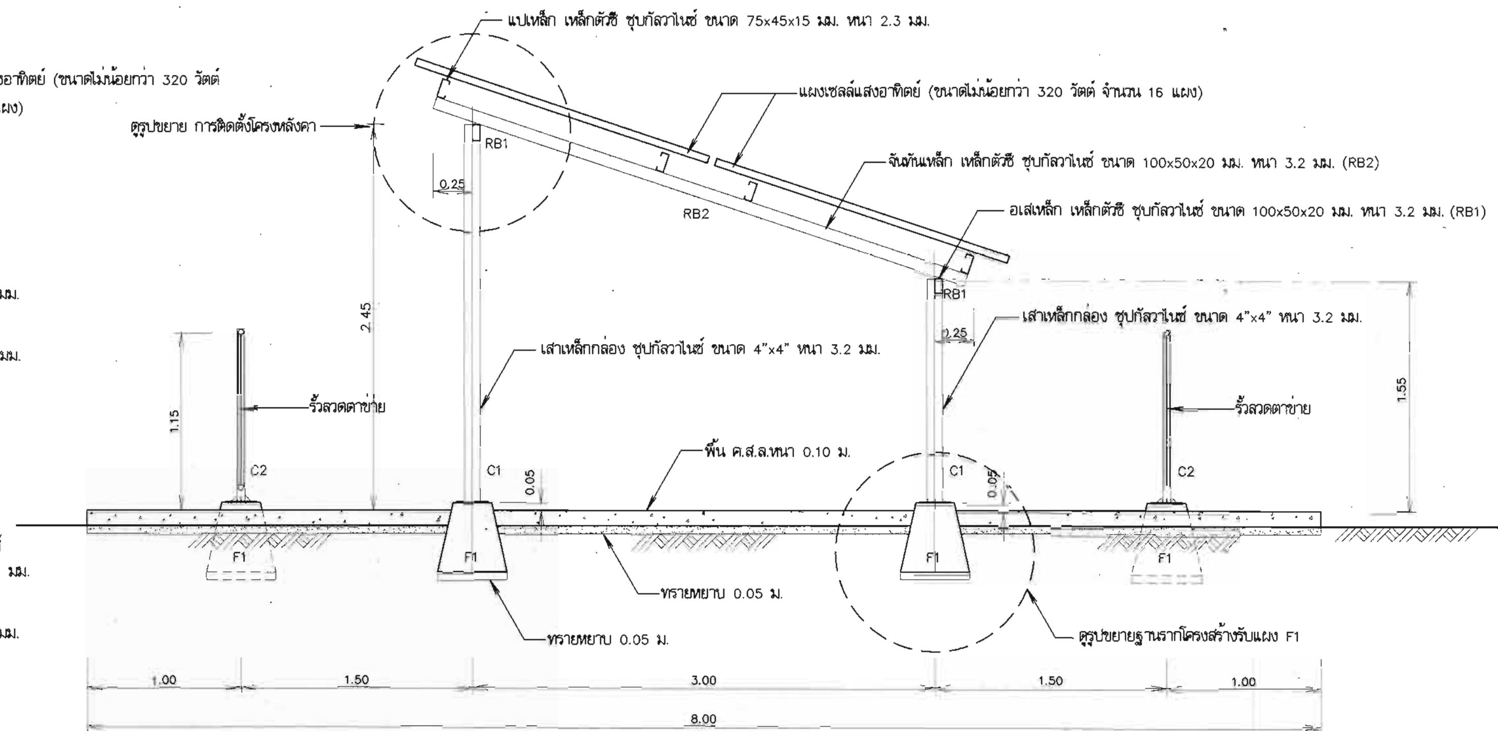
รูปด้านข้าง ไม่แสดงขนาดบางส่วน
