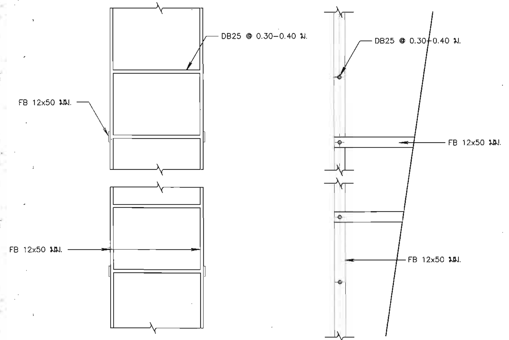
แบบขยายบันได ภายในทองถึงสูง ไม่แสดงมาตราส่วน
