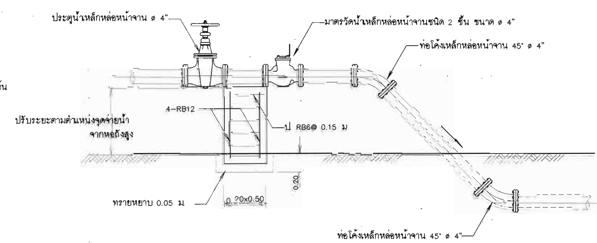
14. การติดตั้งมาตรวัดน้ำบนพื้นดิน ๑ 4" ไม่แสดงขนาดสาย
