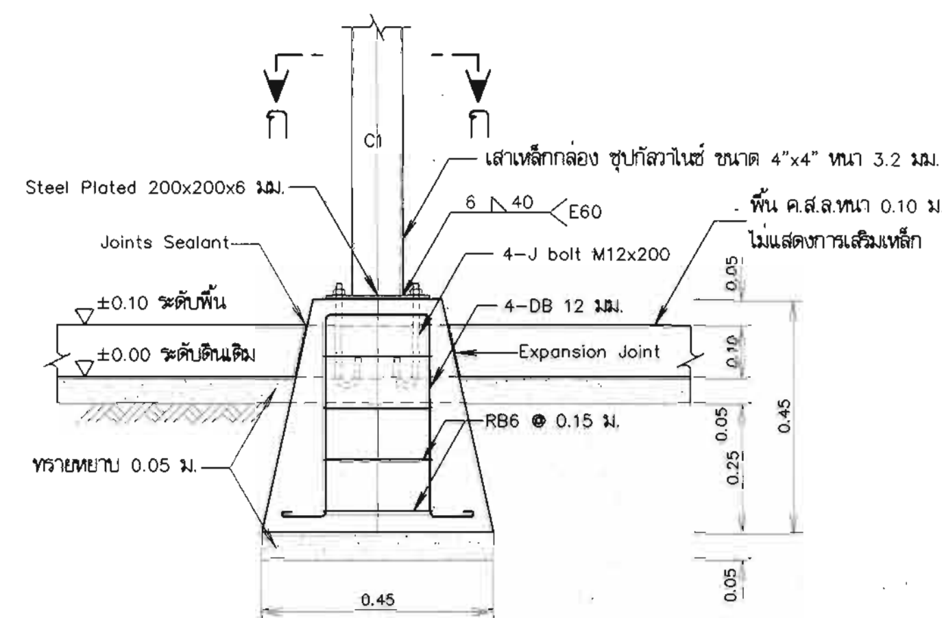
รูปขยายฐานรากโครงสร้างรับแผง F1 (คานา คสล. ท่อลึงาโครงสร้างรับแผง) ไม่แสดงขนาดบางส่วน
