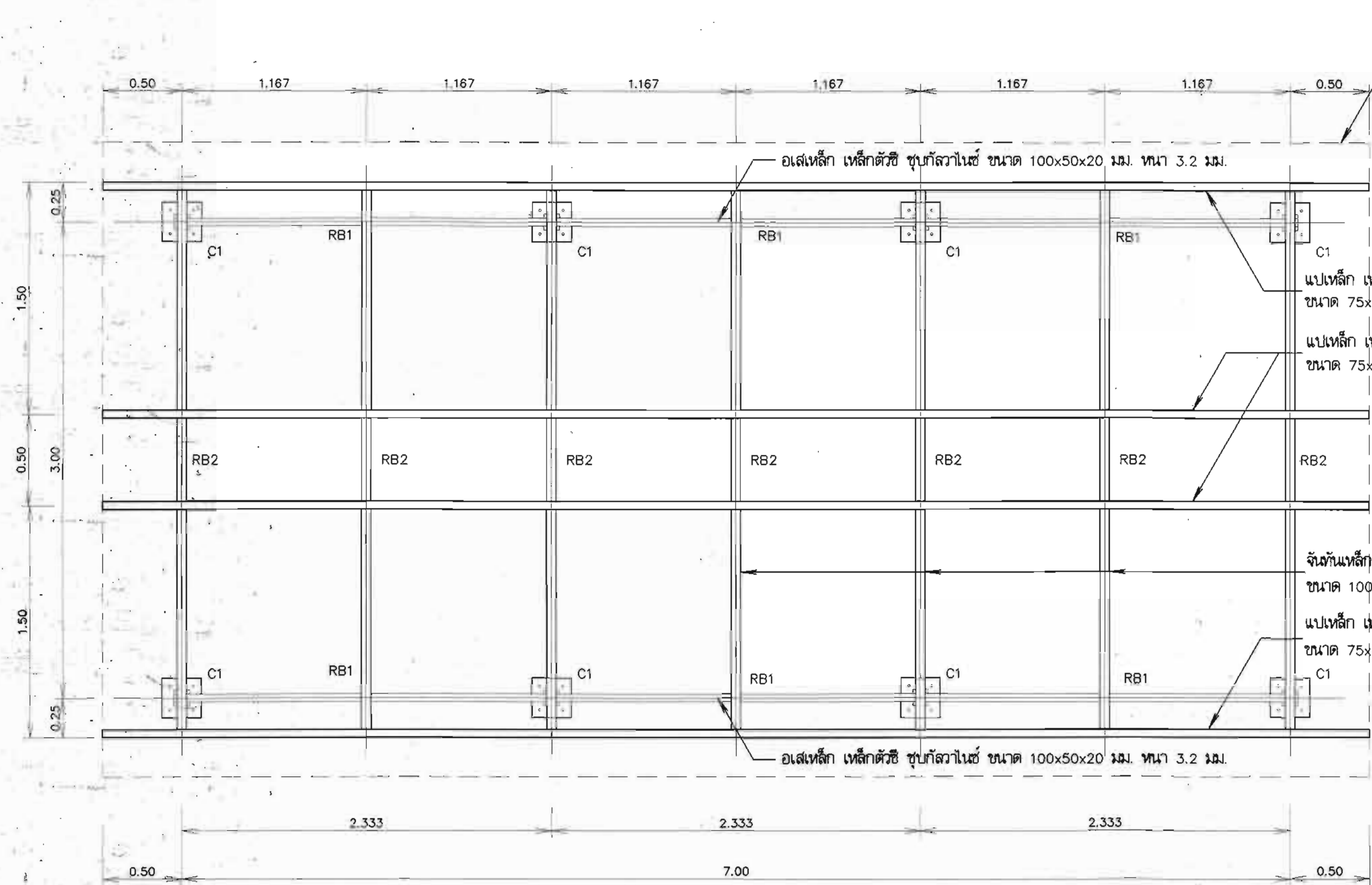
แปลนฐานรากและโครงหลังคา ไม่แสดงขนาดบางส่วน
