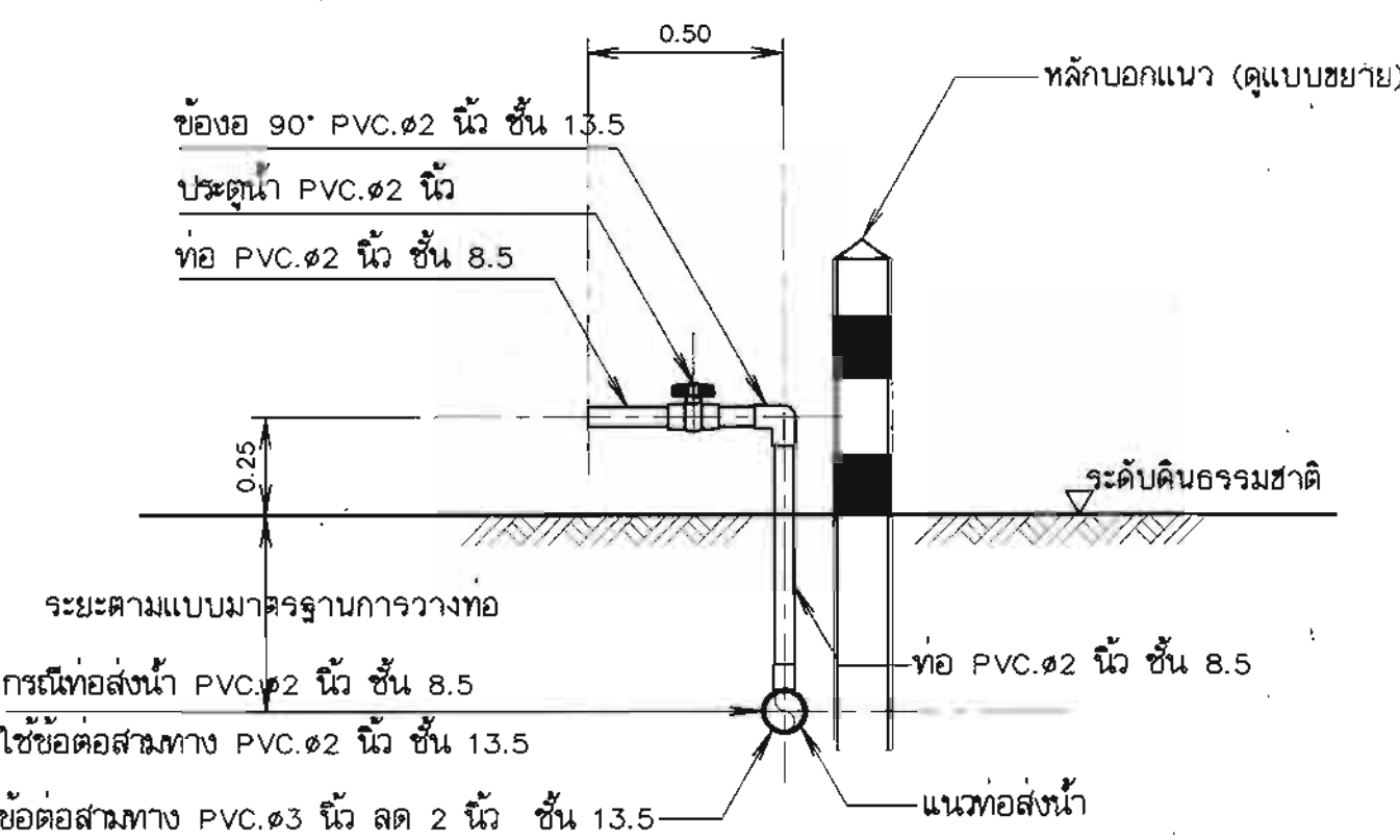
รูปตัด ก - ก แสดงการติดตั้งอาคารจุดปล่อยน้ำ มาตราส่วน 1 : 20
