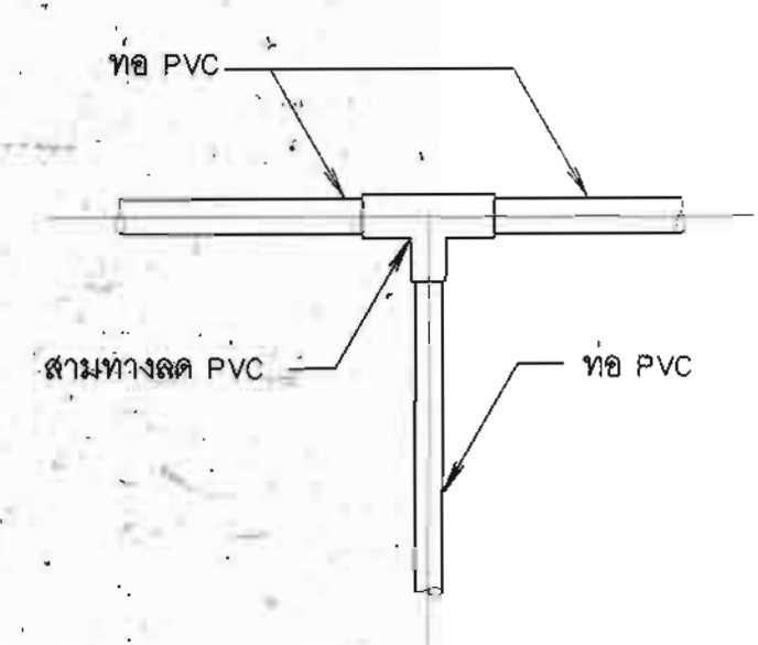
9. แบบการต่อสามทางลด PVC ไม่แสดงขนาดสาย
