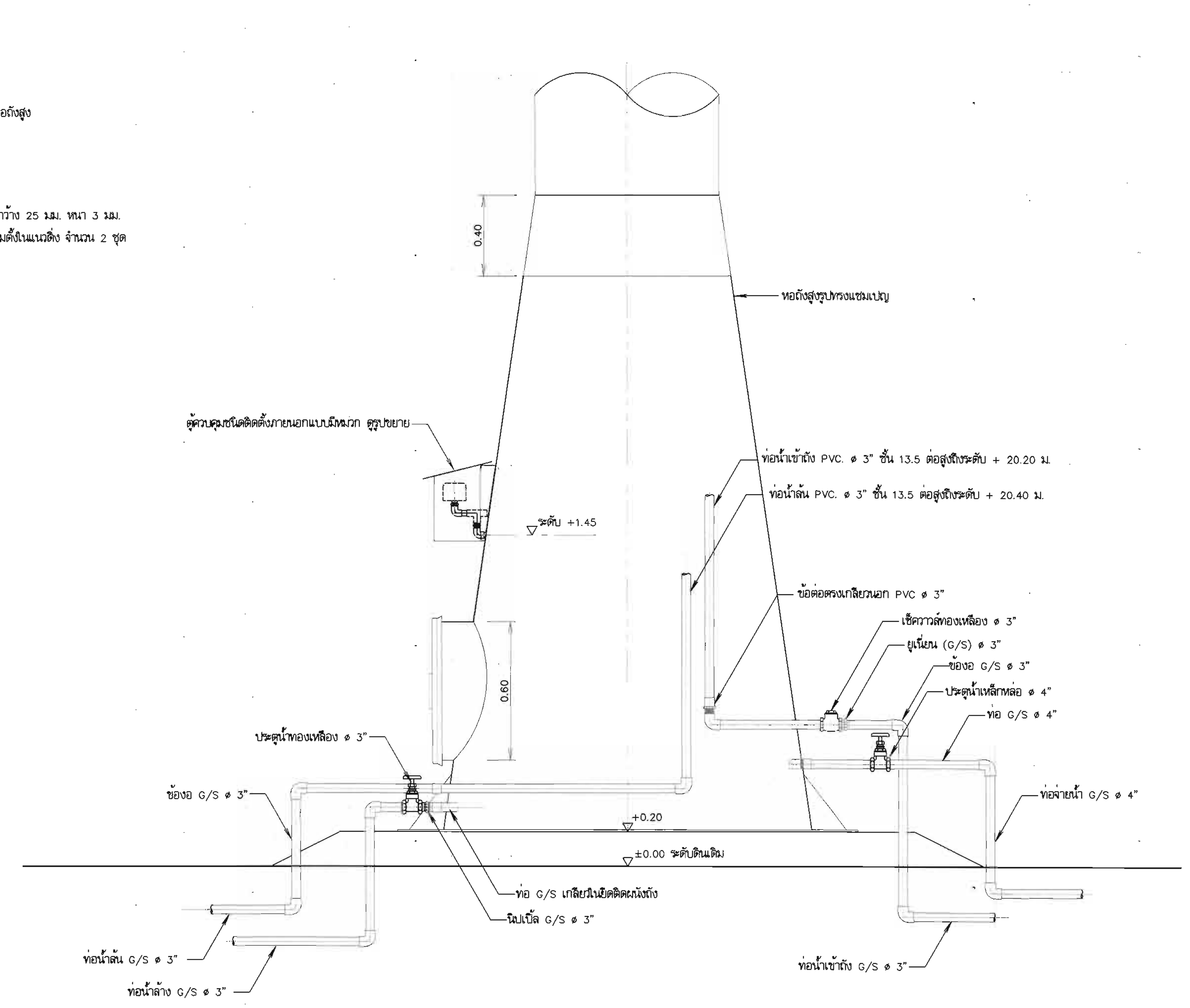
แบบแสดงการเดินท่อน้ำทองถึงสูง ไม่แสดงมาตราส่วน
