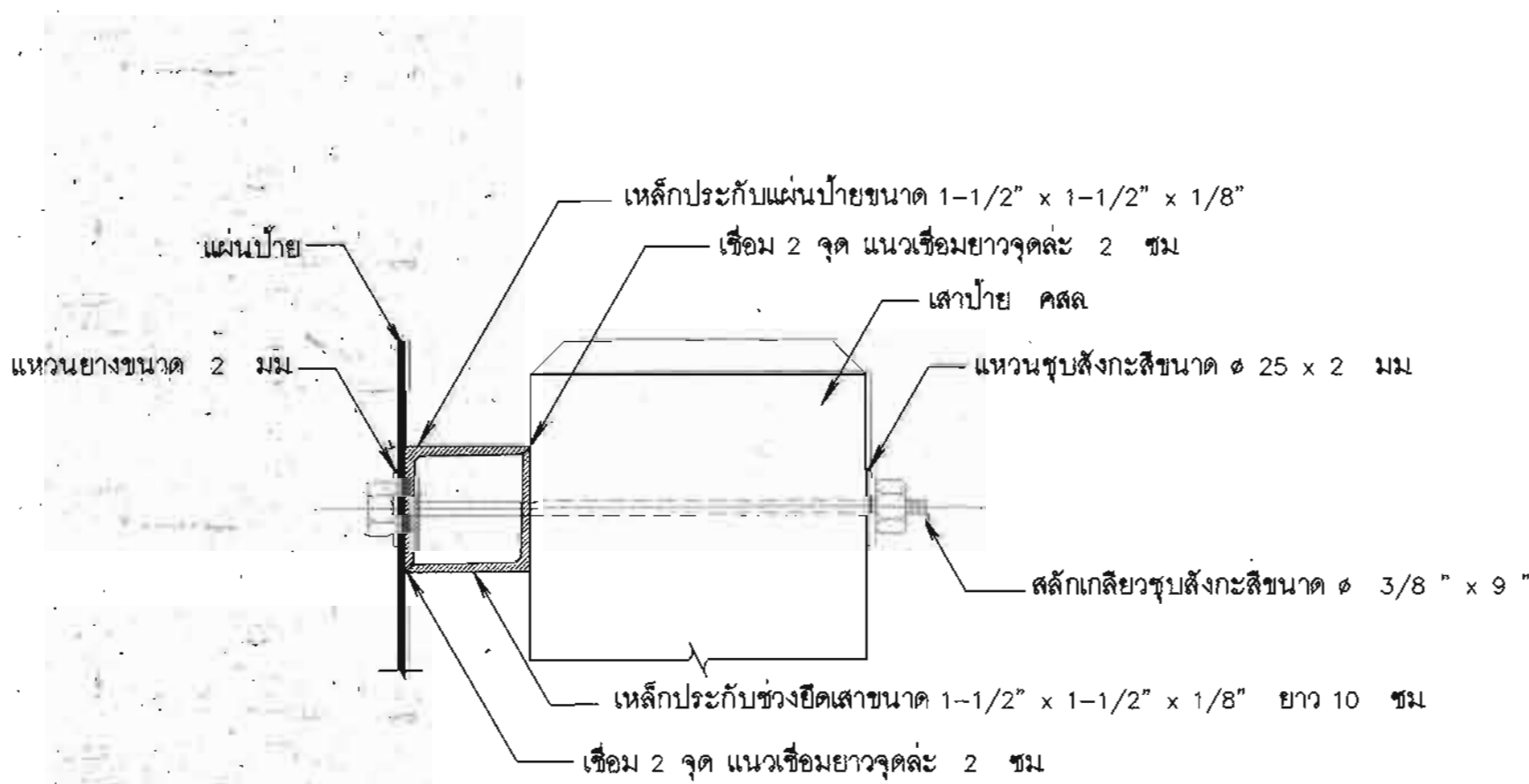
รูปตัดขยายการยึดแผ่นป้ายและเสา ไม่แสดงมาตราส่วน
