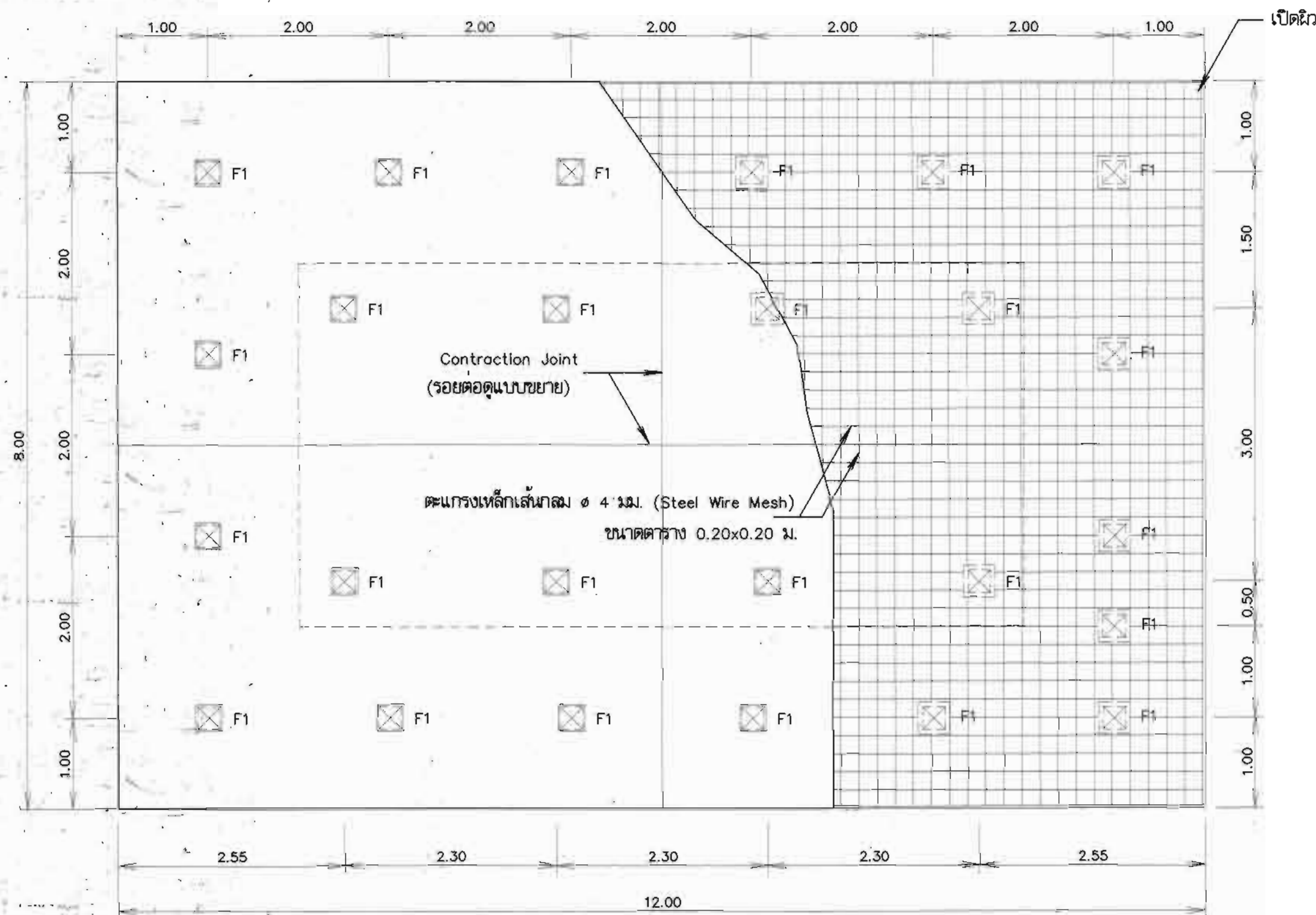
รูปขยายพื้นคอนกรีต ไม่แสดงขนาดบางส่วน
