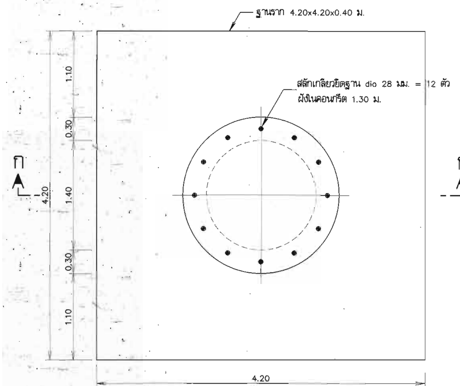
แปลน ฐานรากหอดึงสูง (แบบฐานแผ่)
