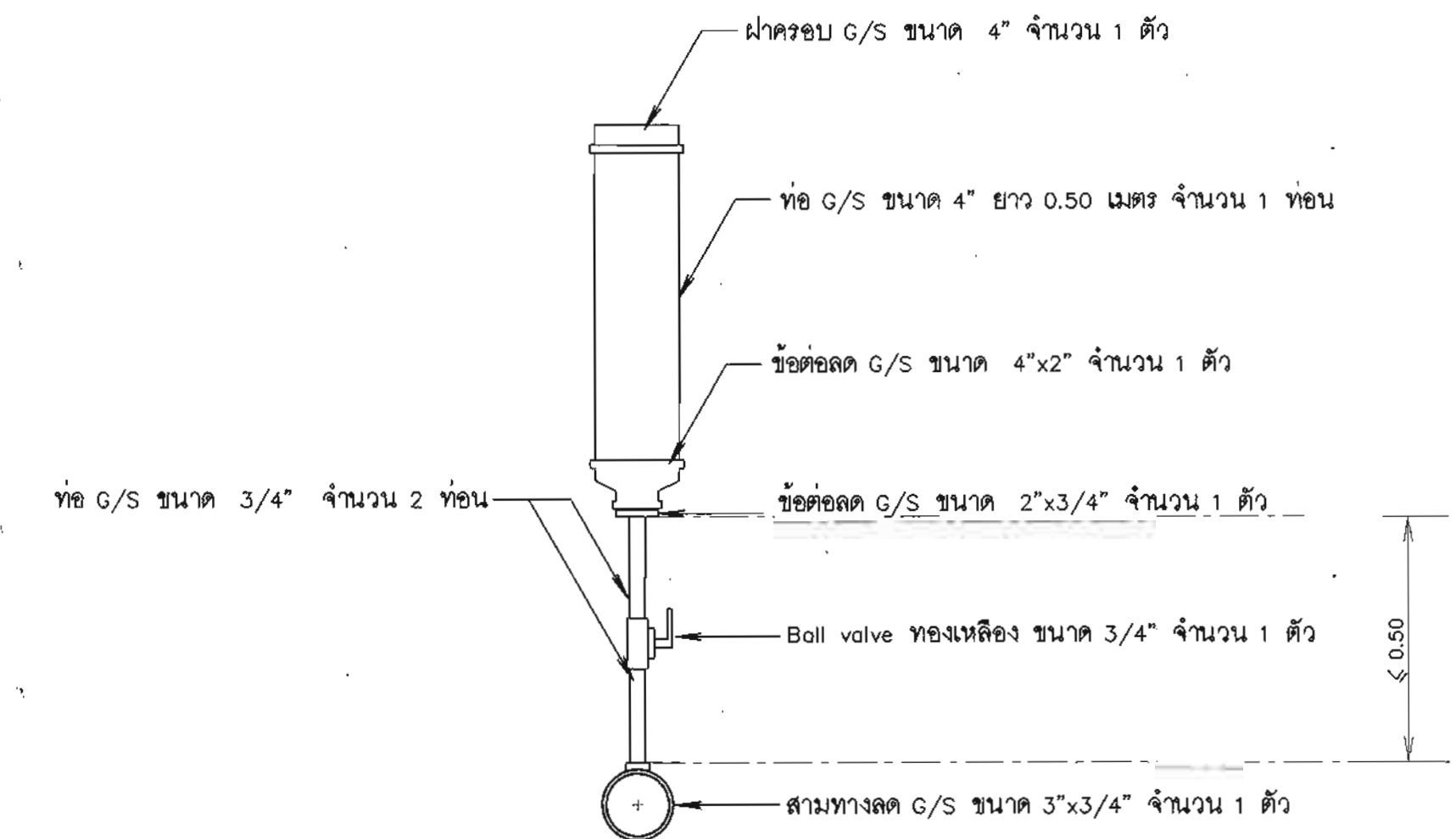
11. ช้องเต็มน้ำ ไม่แสดงขนาดสาย
