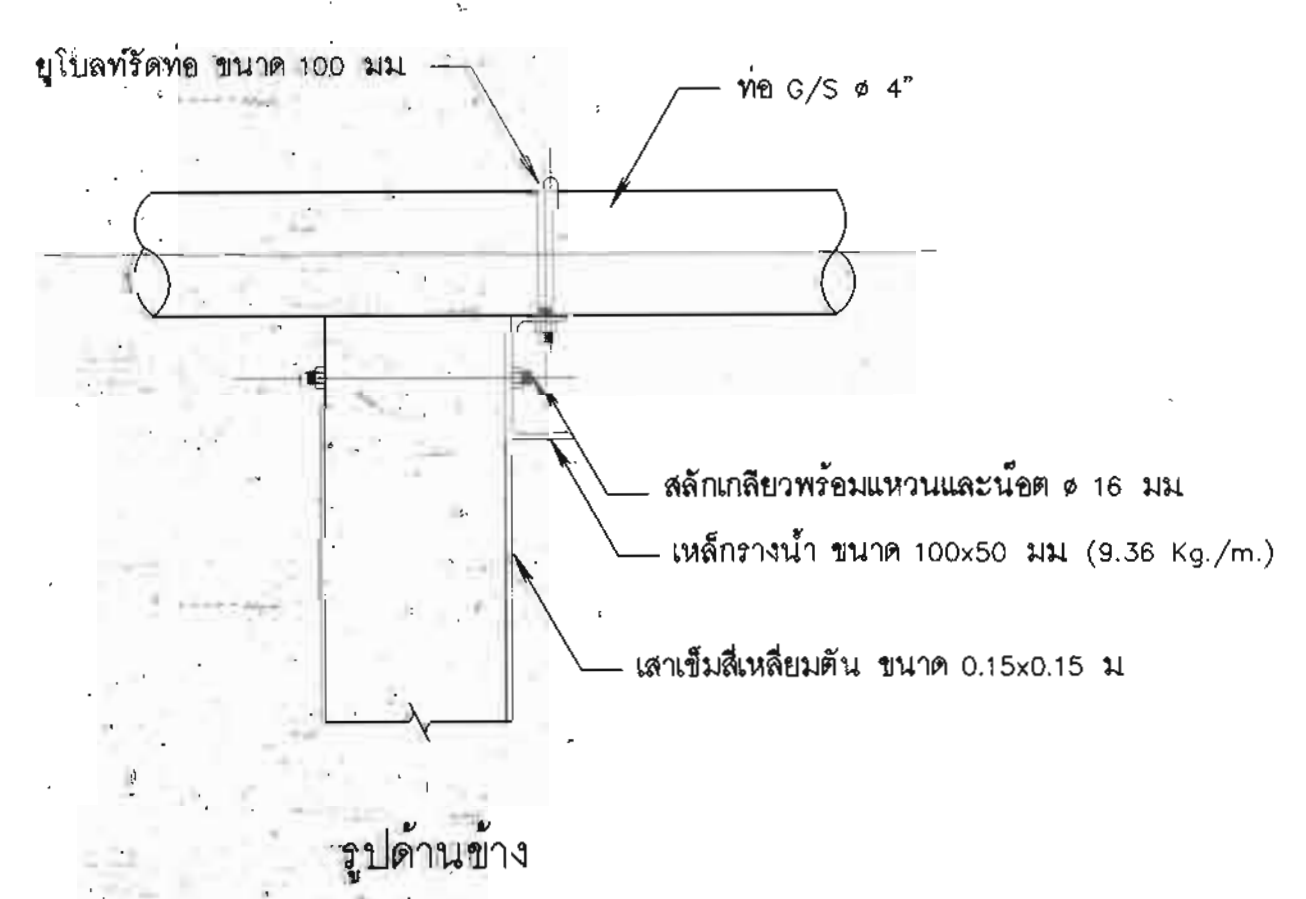
13. เสาต่อมอรับท่อชุด และแบบขยายอุปกรณ์รัดท่อ ไม่แสดงขนาดสาย
