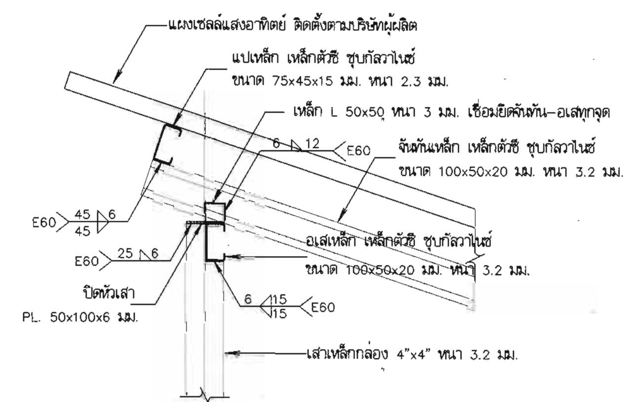
รูปขยาย การติดตั้งโครงหลังคา ไม่แสดงขนาดบางส่วน
