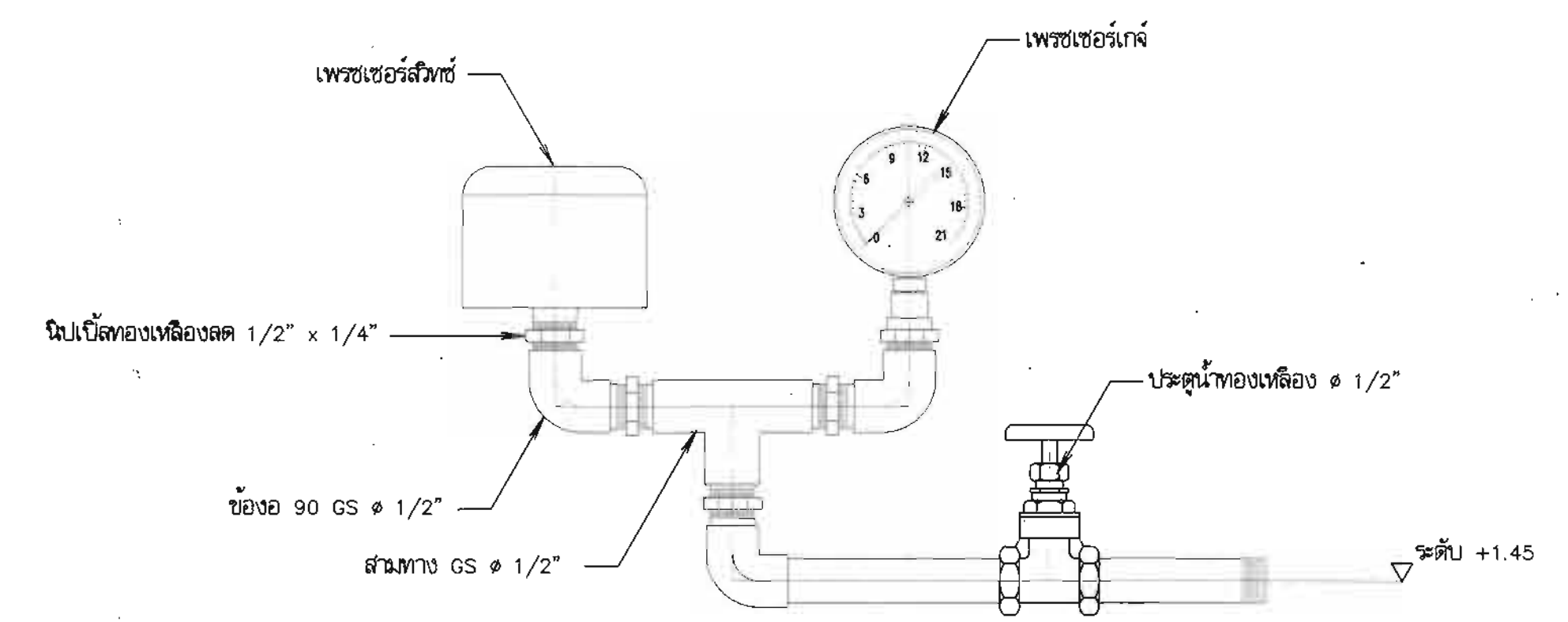
แบบขยายลิฟท์ควบคุมและเก้วัดความดัน ไม่แสดงมาตราส่วน
