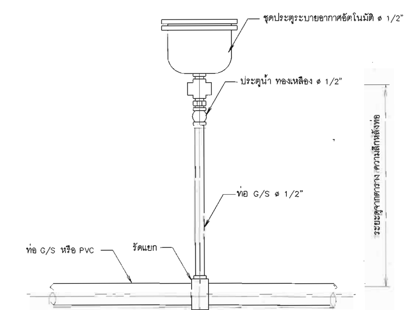
12. การติดตั้งประตูปะบายอากาศอัตโนมัติ ไม่แสดงขนาดสาย
