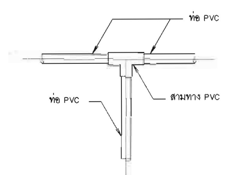
10. แบบการต่อสามทาง PVC ไม่แสดงขนาดสาย
