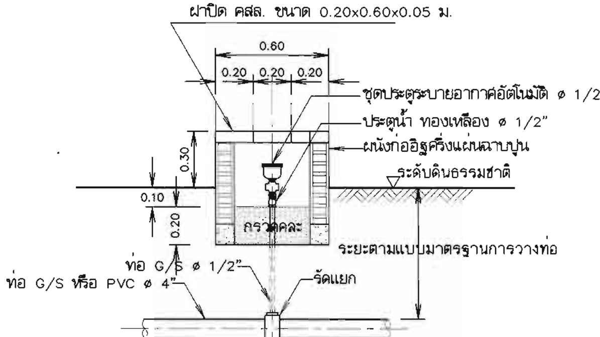
แบบขยายการติดตั้งประตุน้ำอากาศอัตโนมัติ มาตราส่วน 1 : 20
