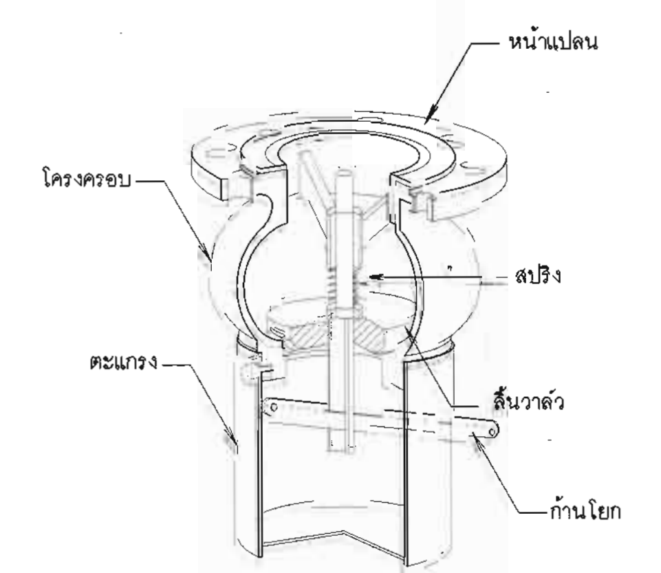
ฟุตวาล์ว แบบก้านโยก ไม่แสดงขนาดสาย
