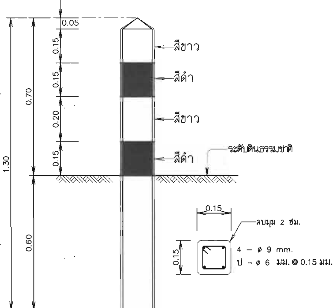
แบบขยายหลักบ่อแก้ว มาตราส่วน 1 : 10
