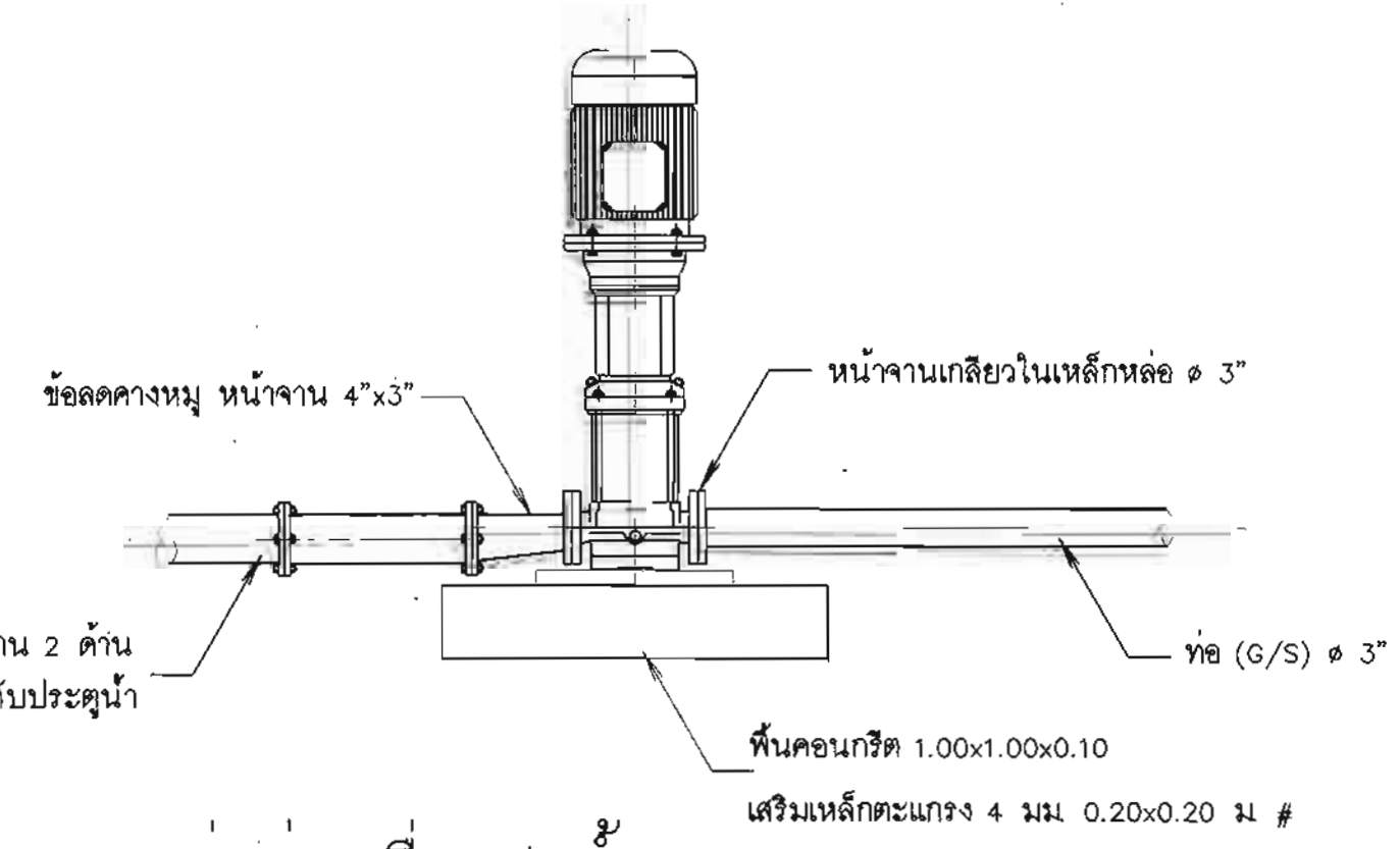
15. การต่อท่อเครื่องสูบน้ำ ไม่แสดงขนาดสาย
