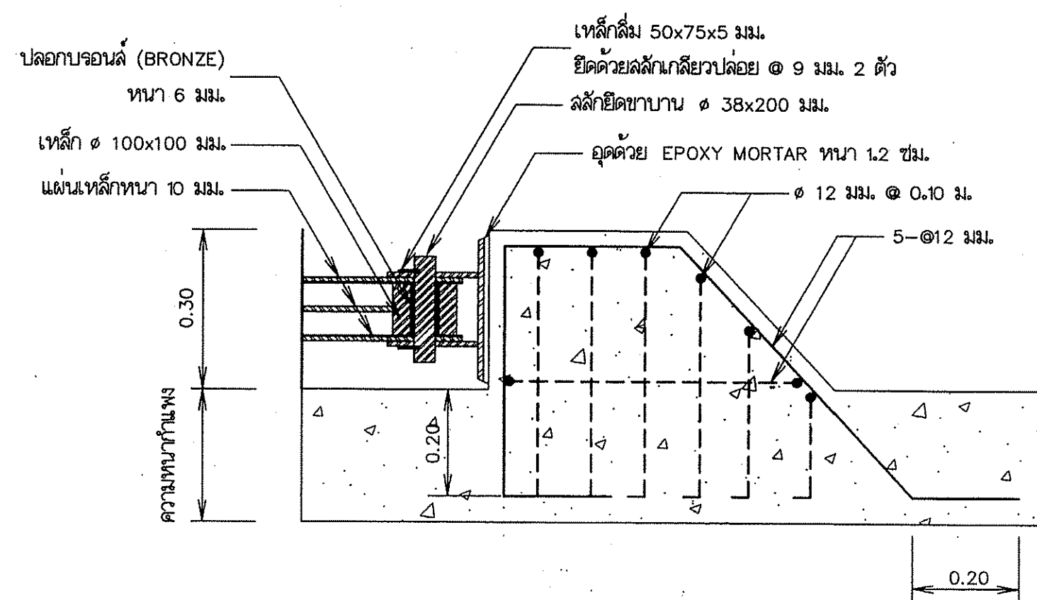
รูปตัดแสดงการเสริมเหล็กและงานยึดบานประตู มาตราส่วน 1:10
