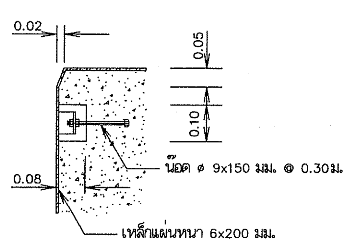
รูปตัดขยาย ข - ข มาตราส่วน 1:10
