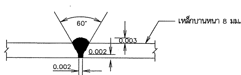
แบบขยายการต่อเชื่อมแผ่นเหล็กบาน มาตราส่วน 1:1
