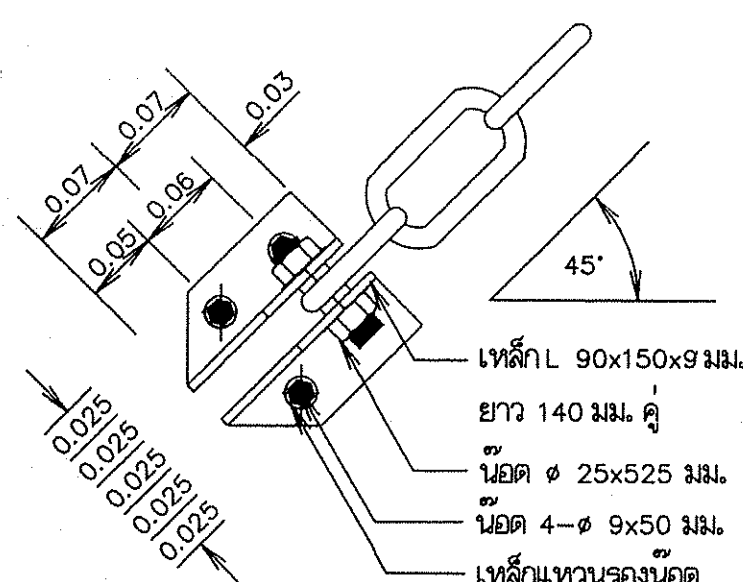
รูปด้านแสดงการยึดขันติดบาน
