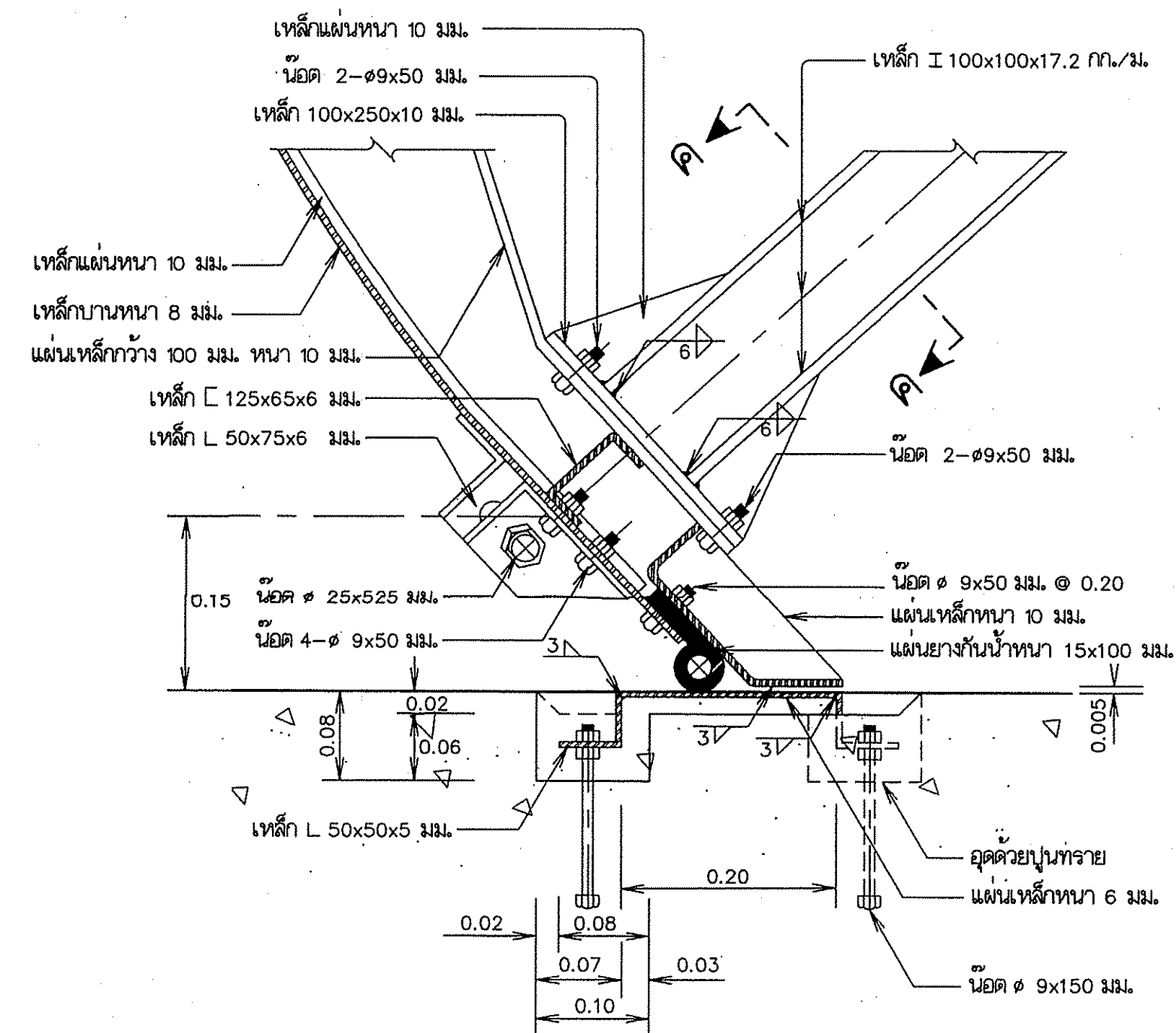
รูปขยาย 3
