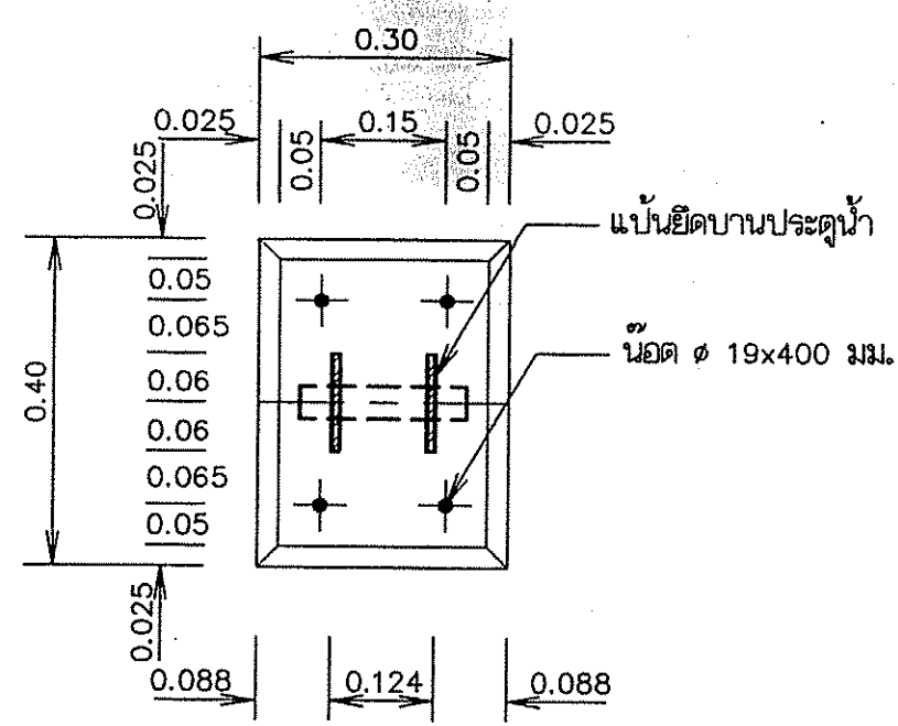
รูปขยายบานยึดบานประตู มาตราส่วน 1:10
