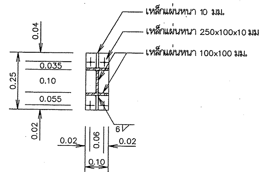
รูปตัดขยาย ค - ค มาตราส่วน 1:10
