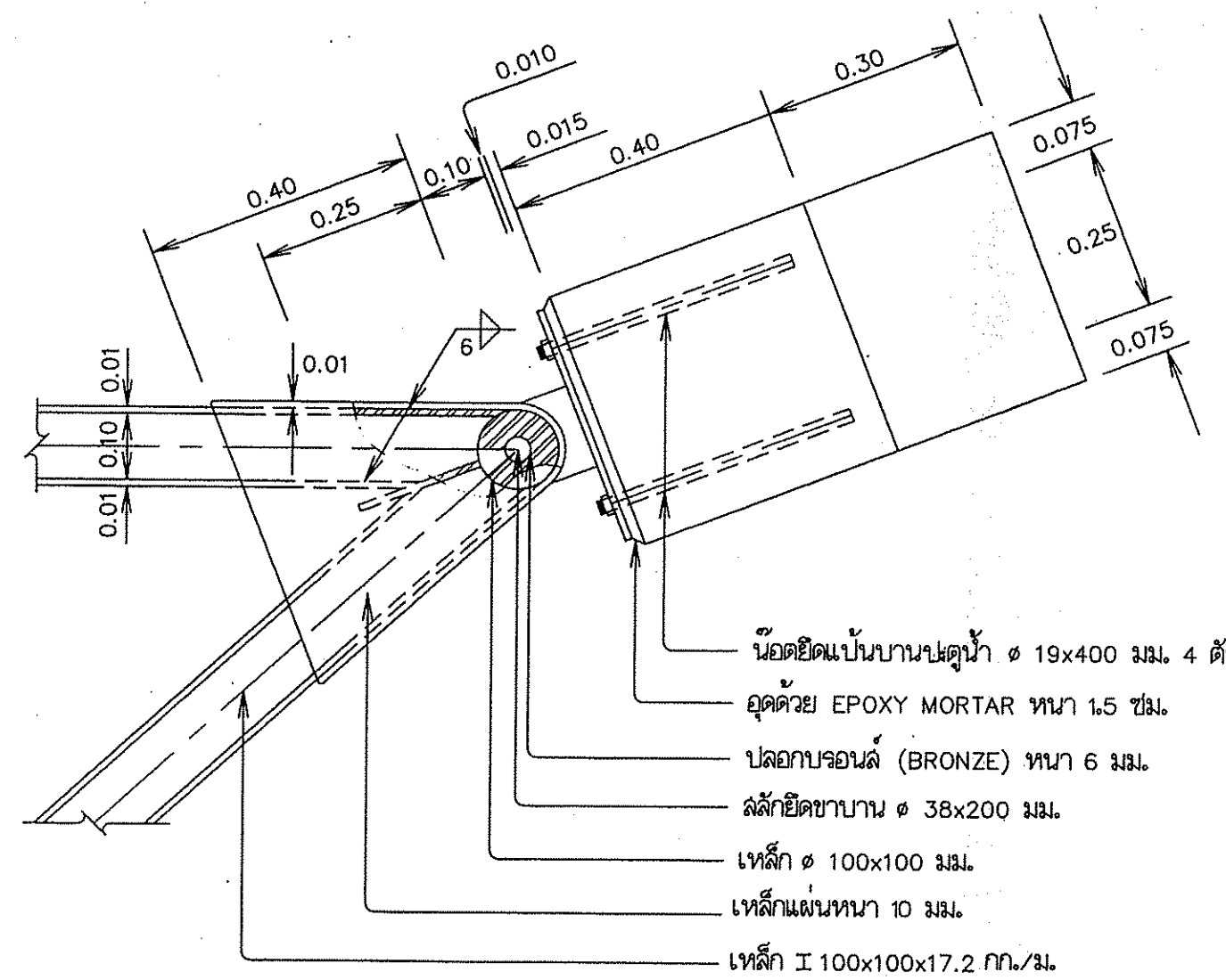
รูปขยาย 4 มาตราส่วน 1:10
