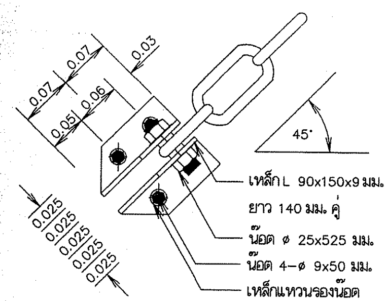
รูปด้านแสดงการยึดปิดบาน มาตราส่วน 1:5
