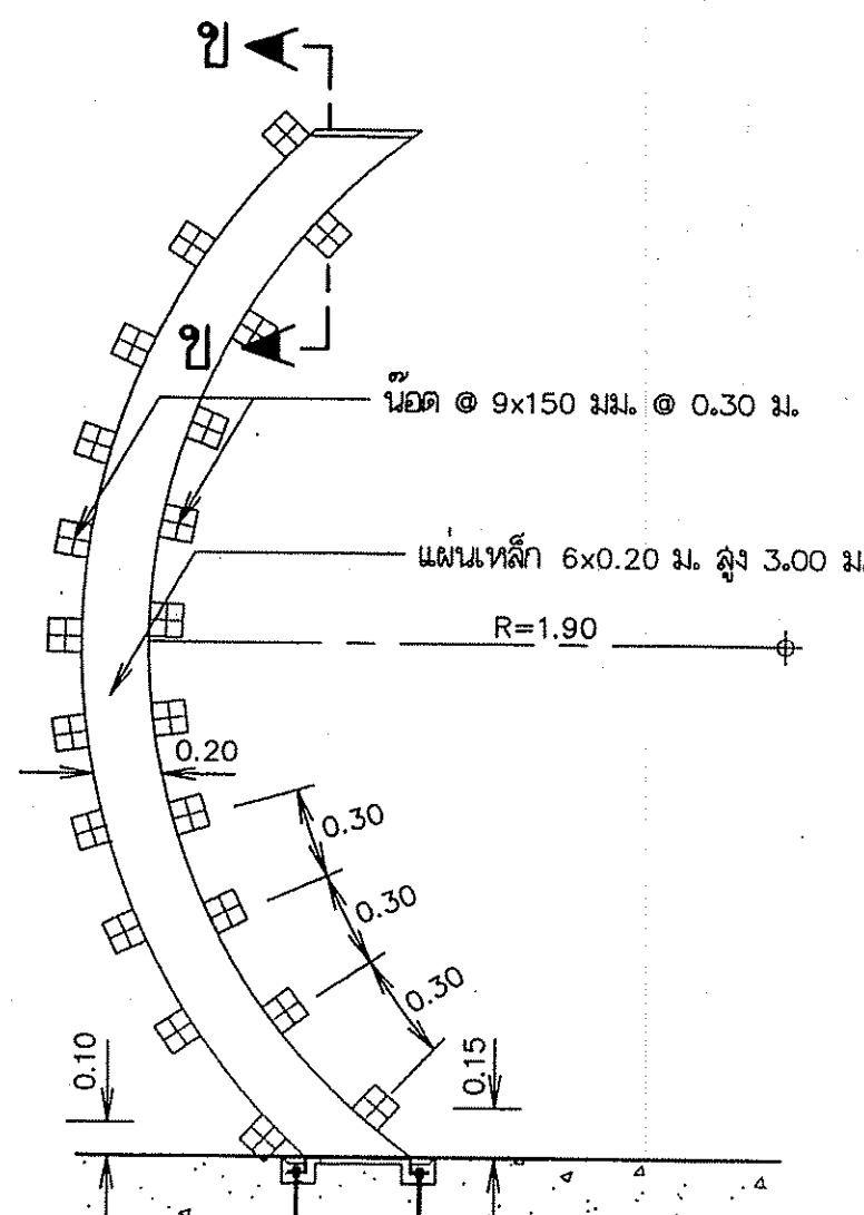
แปลนรองยางกันน้ำด้านพื้นล่าง มาตราส่วน 1:25
