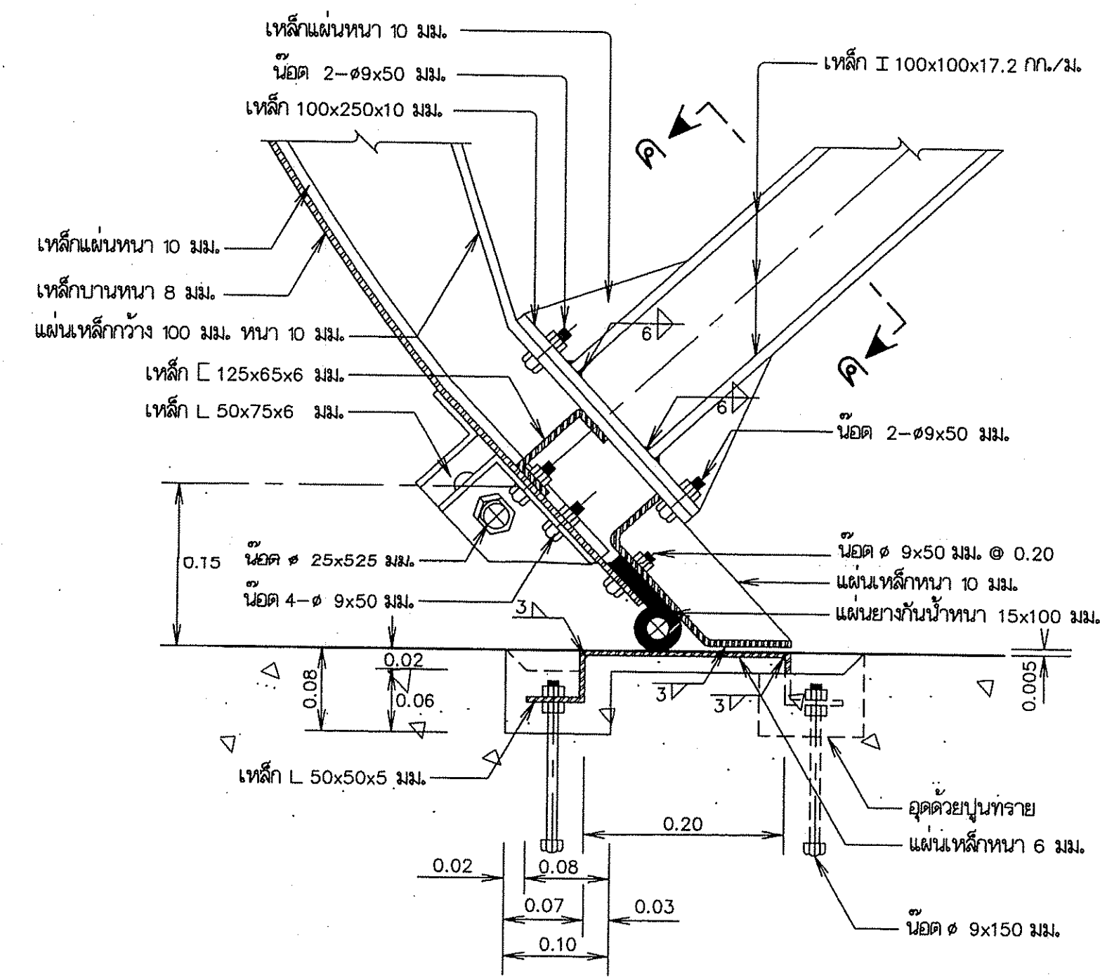
รูปขยาย 3 มาตราส่วน 1:5
