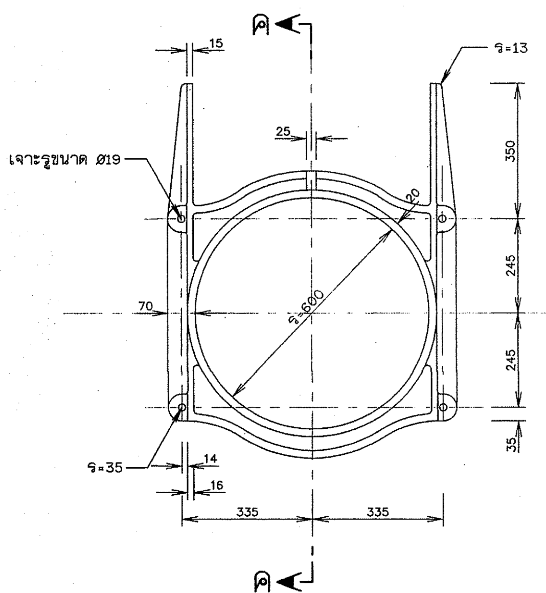
กรอบบาน(เหล็กหล่อ) มาตราส่วน 1:10
