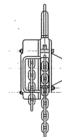
รอกใช้มือสว่านขนาด 3 ตัน ระยะยก 3.00 เมตร
