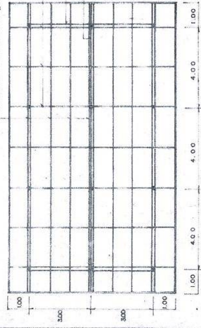
แปลนโครงสร้างหลังคา 18100
