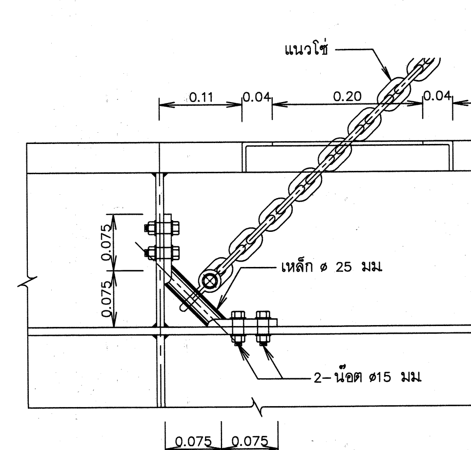
รูปขยาย ตำแหน่งจุดยึดรอกใช้กับบานระบาย
