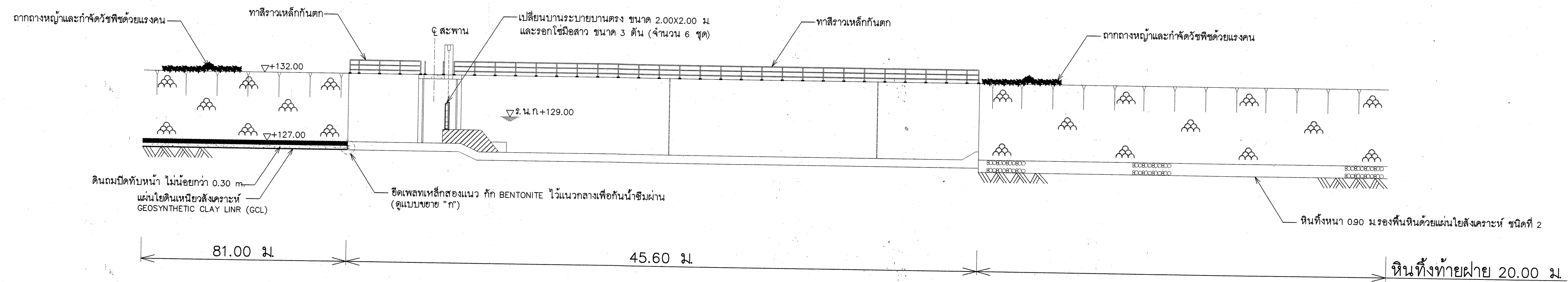
รูปตัด ก-ก มาตราส่วน 1:100
