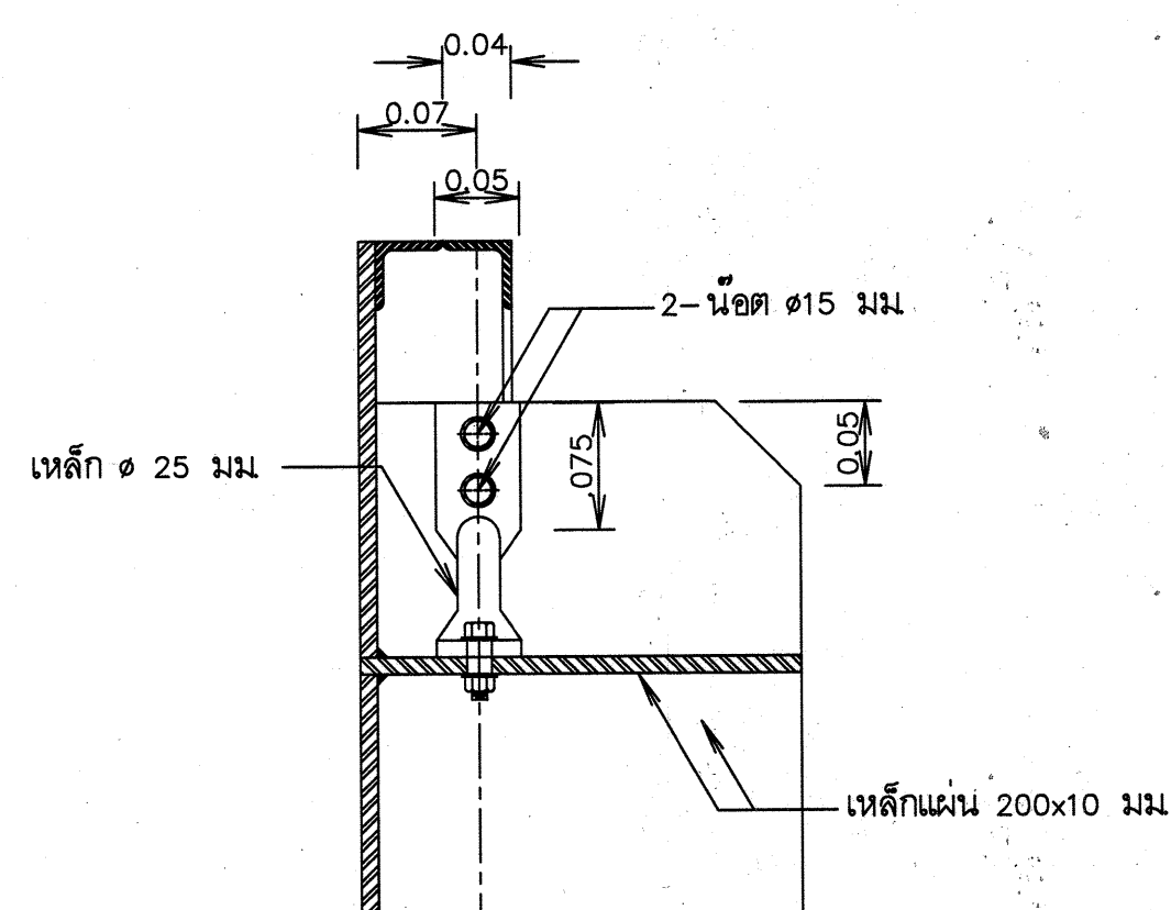
รูปขยาย ตำแหน่งจุดยึดรอกใช้กับบานระบาย
