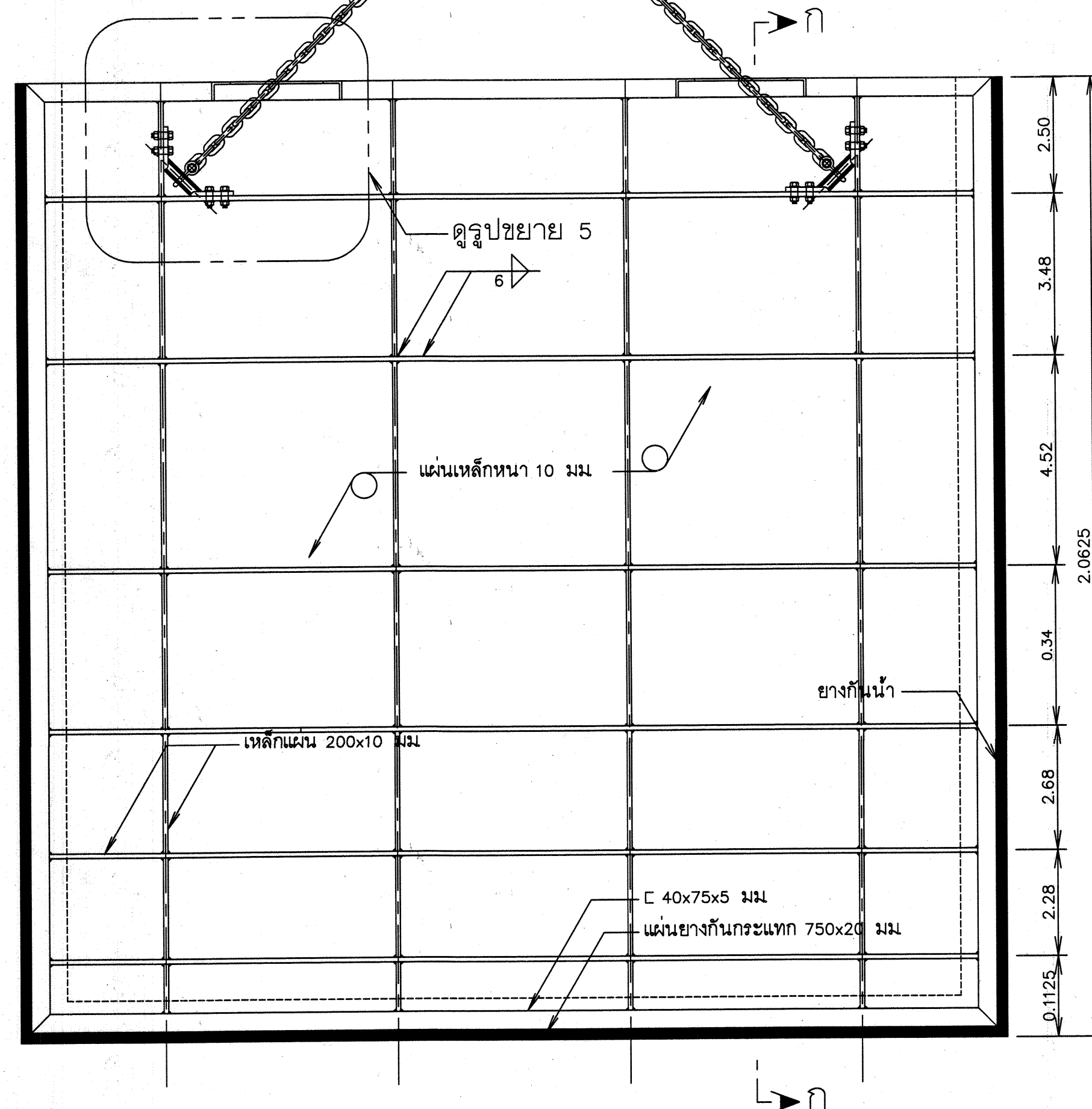
รูปด้านหลังบานประตูระบายทราย
