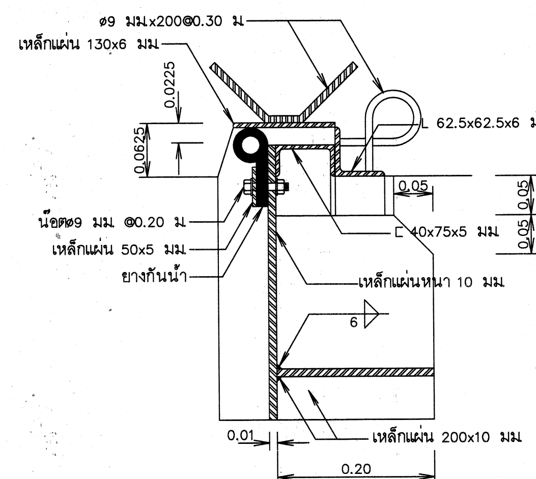
รูปขยายบานระบายด้านติดกำแพง
