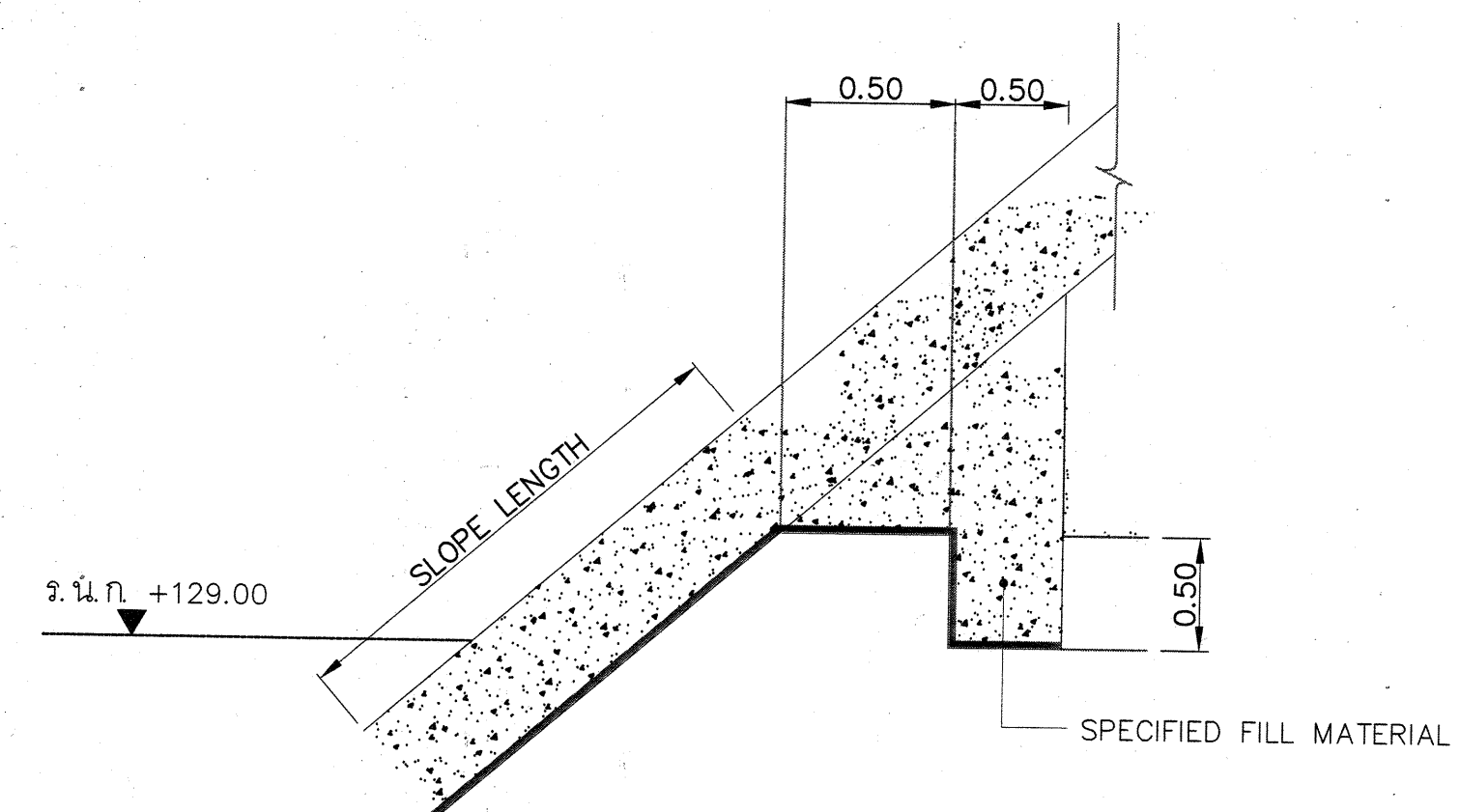
แบบขยาย "ข" ANCHOR TRENCH ไม่แสดงมาตราส่วน
