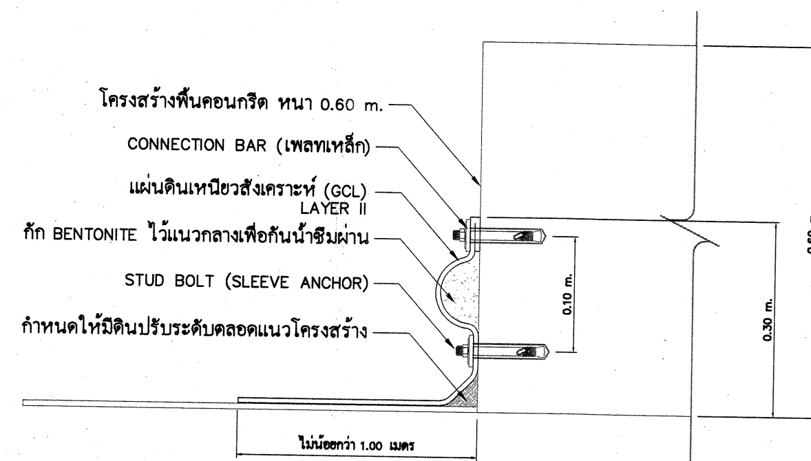
แบบขยาย "ก" การเชื่อมเหล็ก ไม่แสดงมาตราส่วน
