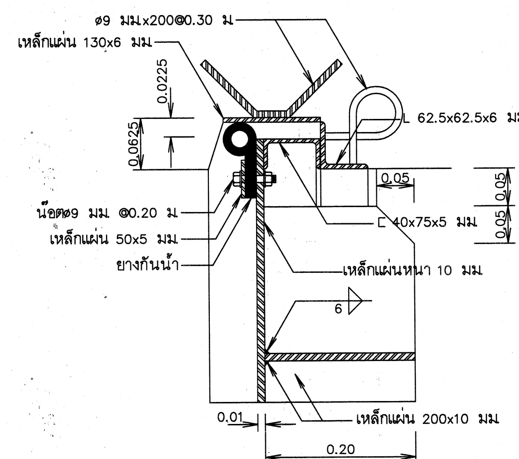
รูปขยายบานระบายด้านติดกำแพง มาตราส่วน 1:5
