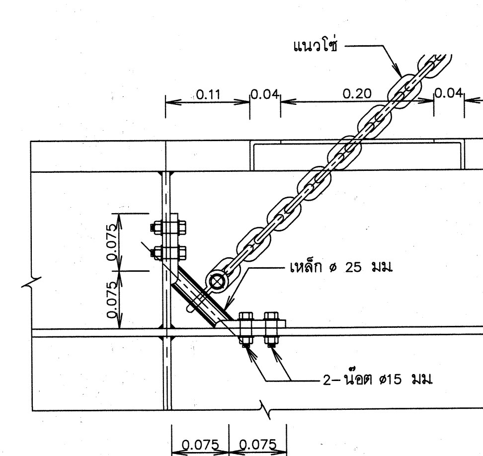
รอกโซ่มือสาวขนาด 3 ตัน ระยะยก 3.00 เมตร มาตราส่วน 1:10
