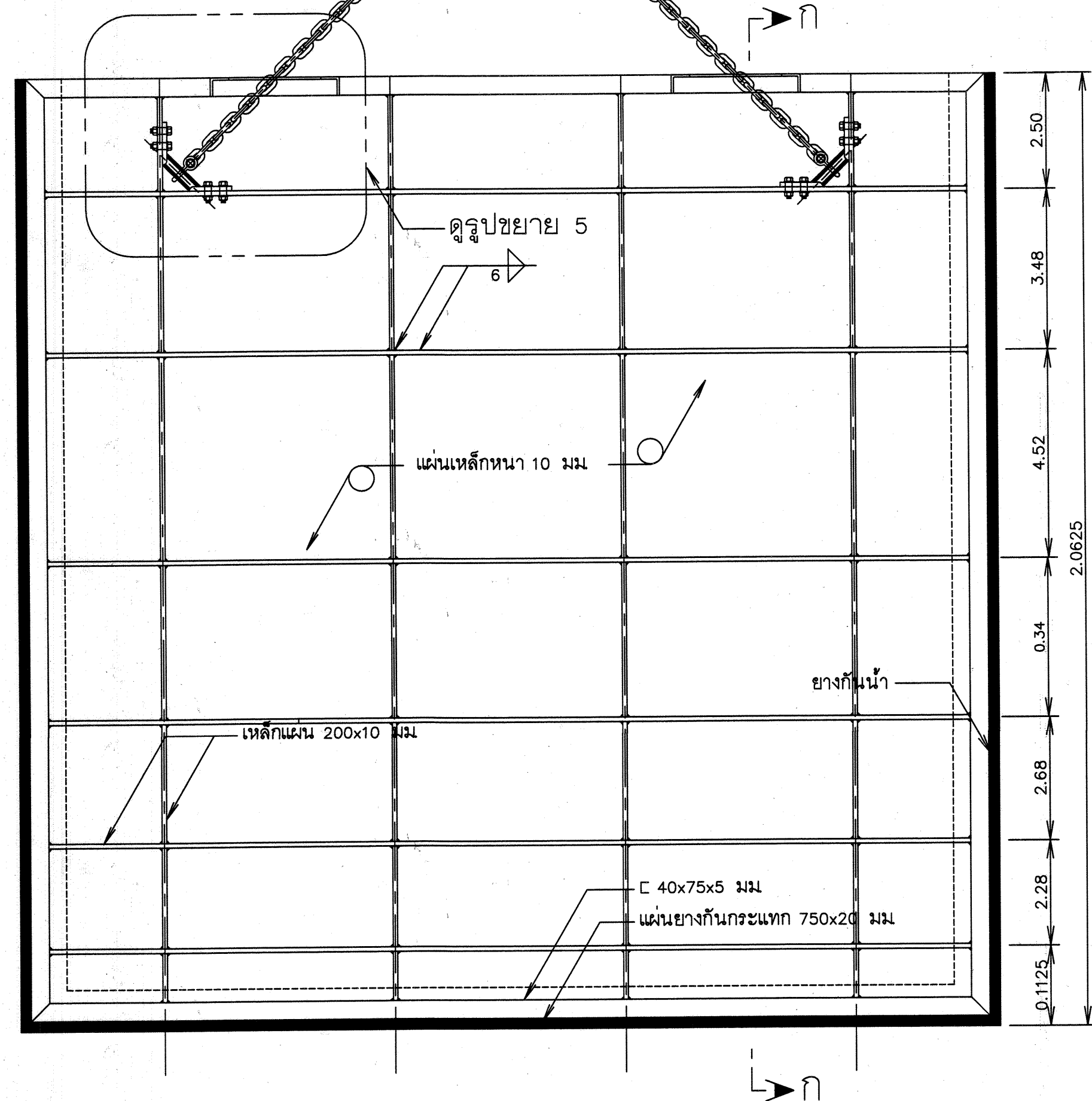
รูปด้านหลังบานประตูระบายทราย มาตราส่วน 1:10
