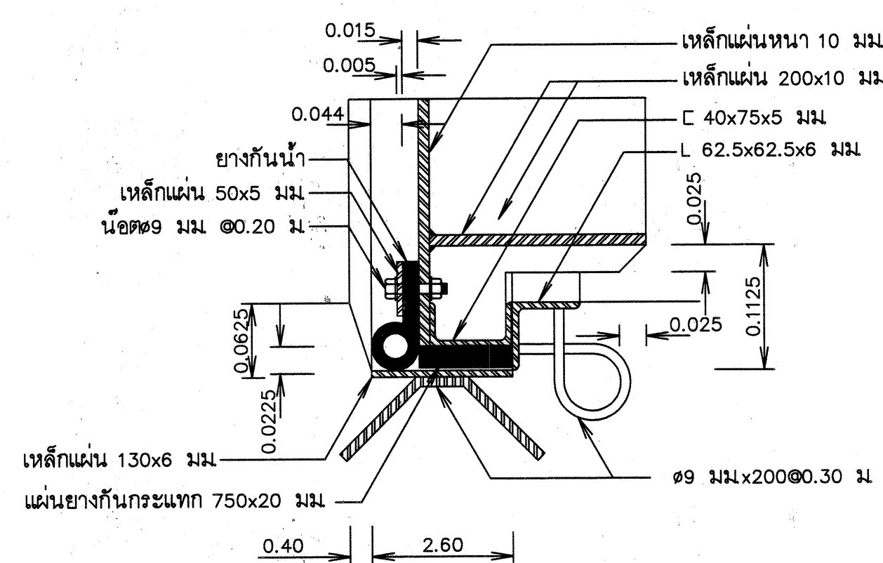
รูปขยายบานระบายด้านติดพื้น มาตราส่วน 1:5
