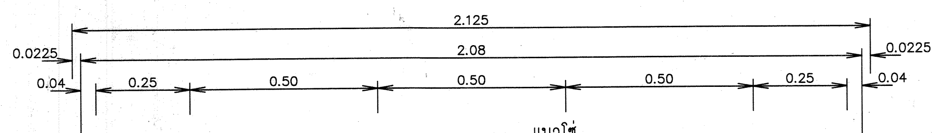
แปลนประตูระบายทราย มาตราส่วน 1:10
