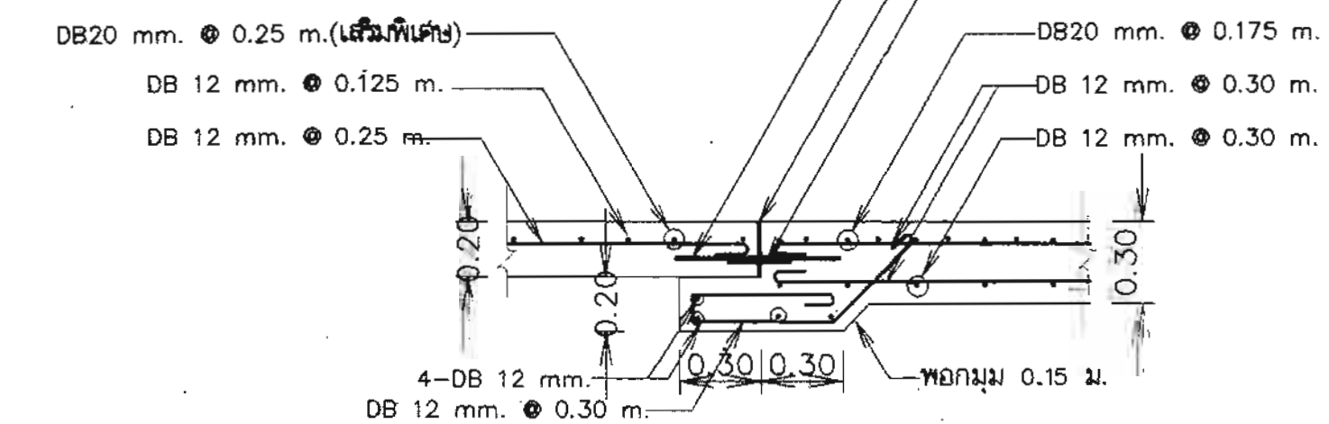
แบบขยาย A-3 มาตรฐาน 1:25
