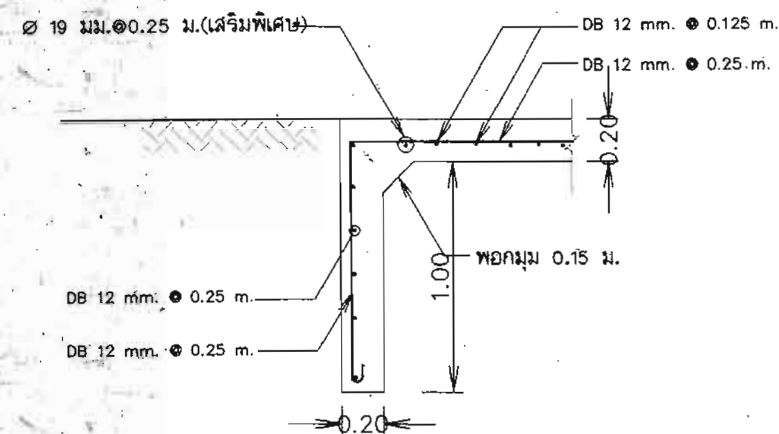
แบบขยาย A-1 มาตรฐาน 1:25
