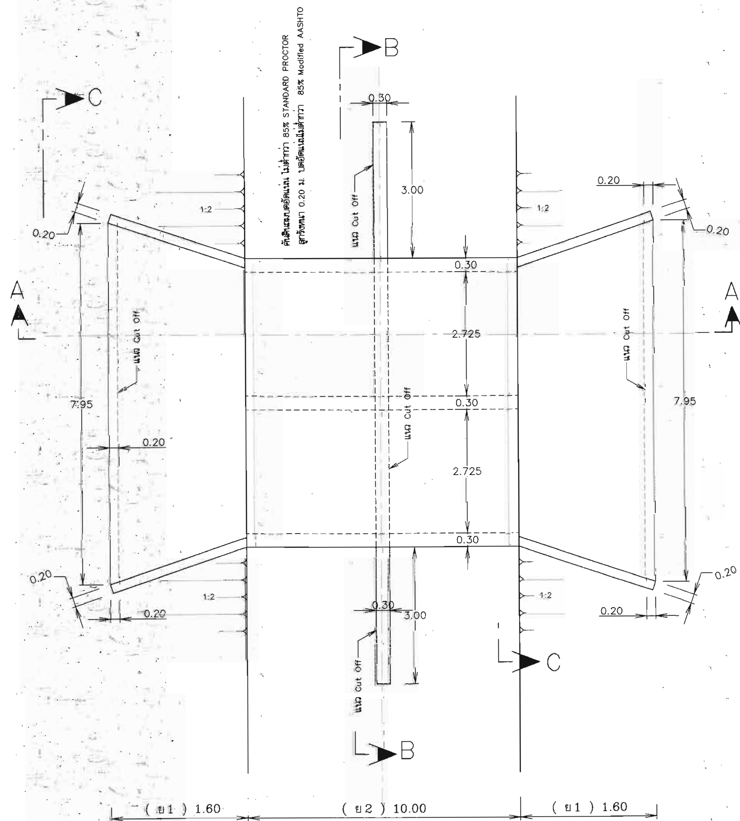
แปลนอาคารระบายนํ้า มาตรฐาน 1:50
