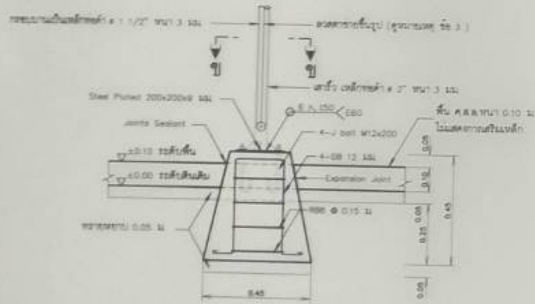
รูปขยายฐานรากโครงสร้างรับแรง F1
