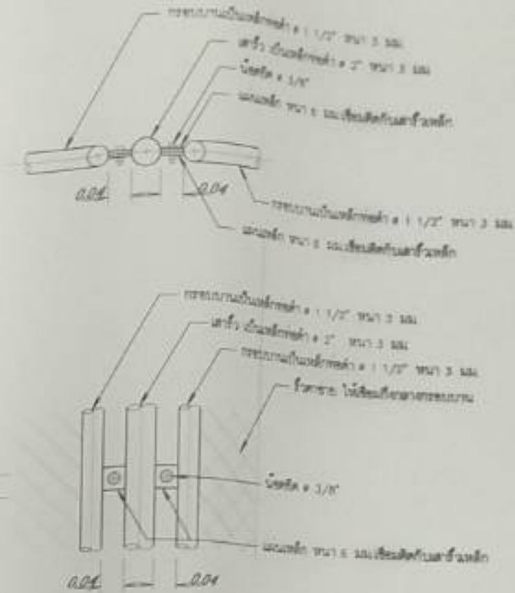
แบบขยายรายละเอียดแสดงการยึดระหว่างตัวบานกับเสา
