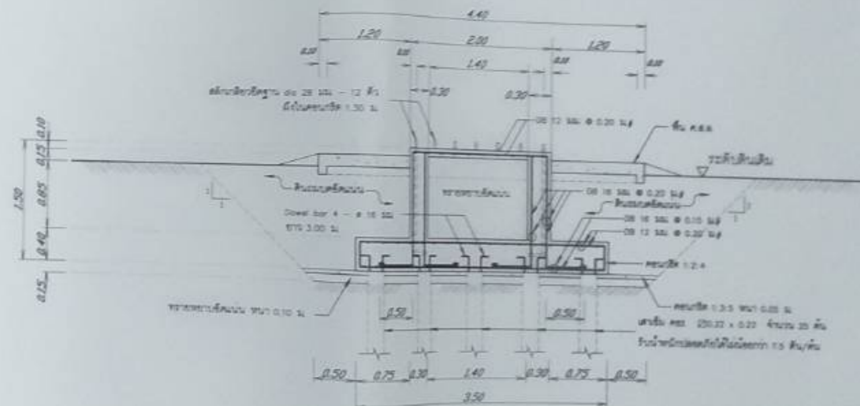
รูปตัด ข-ข
