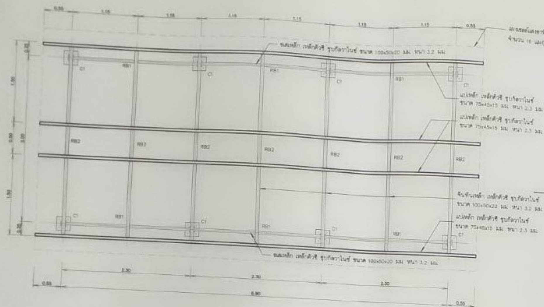
แปลนฐานรากและโครงหลังคา ไม่แสดงเสาเข็ม
