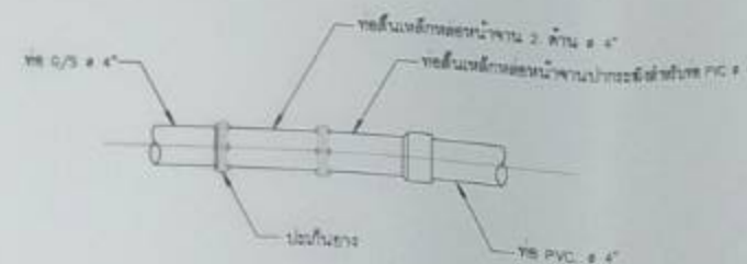
8. การบรรจบท่อเหล็กกับท่อ G/S กับท่อ PVC. ไม่แสดงมาตรฐาน
