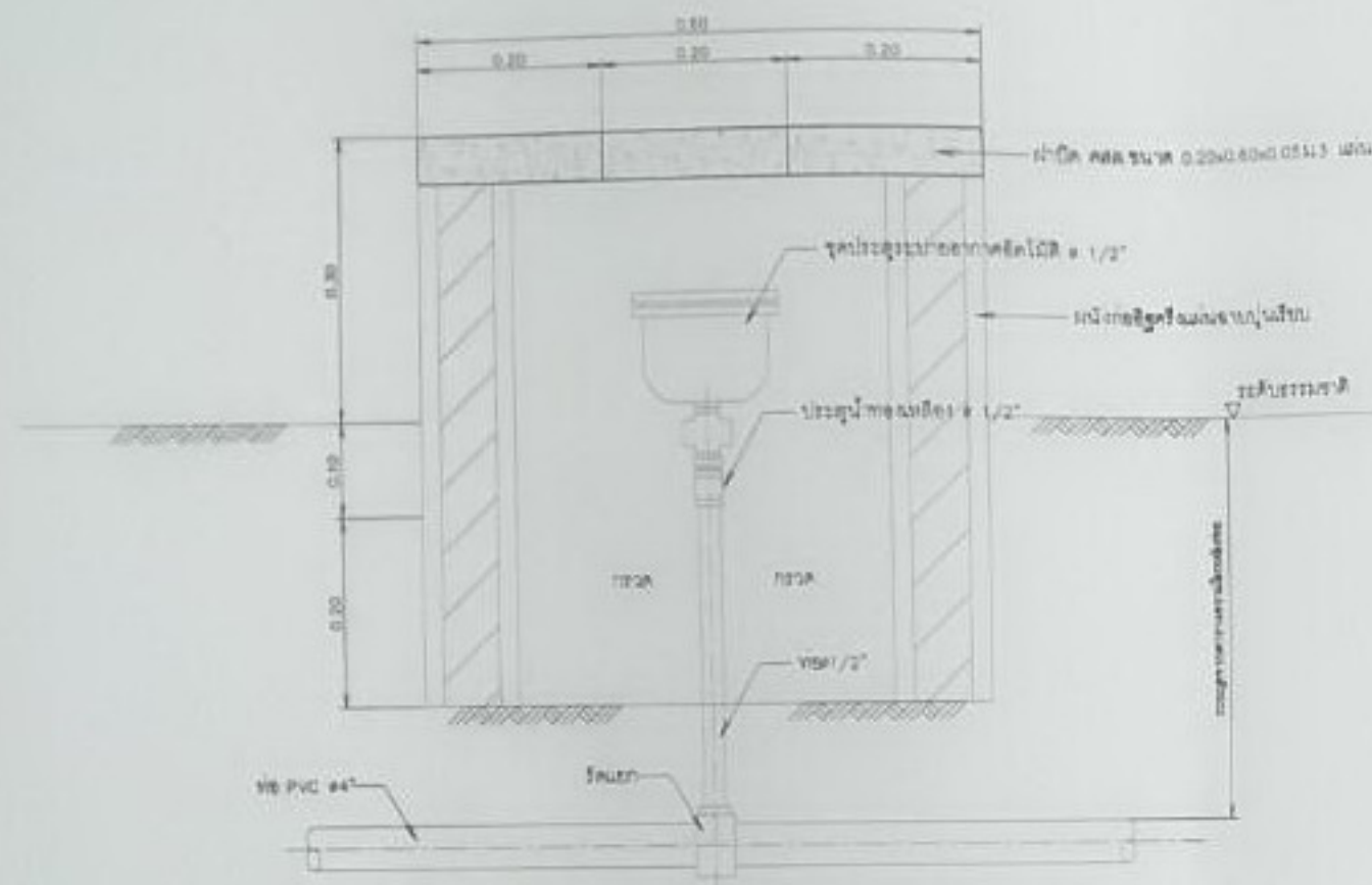
12 การติดตั้งประตูป้ายอากาศอัตโนมัติ มาตราส่วน 1:5
