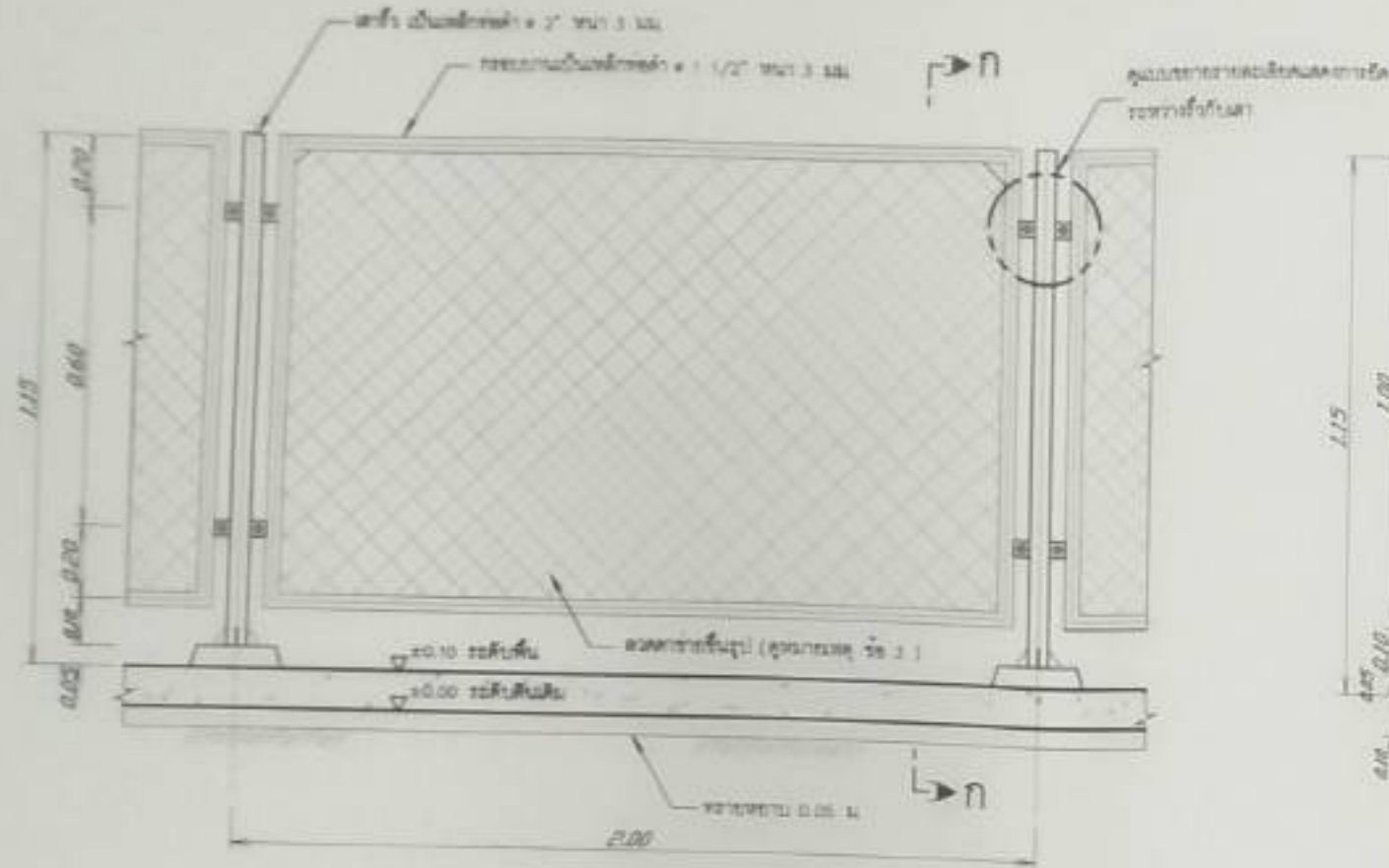
แบบขยายรายละเอียดการยึดระหว่างตัวบานกับเสา
