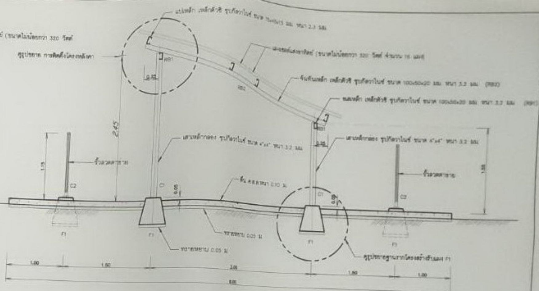
รูปด้านข้าง ไม่แสดงเสาเข็ม
