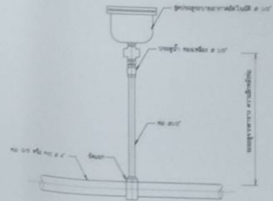
12. การติดตั้งประตูระบายน้ำจากคอกสัตว์ในมด
