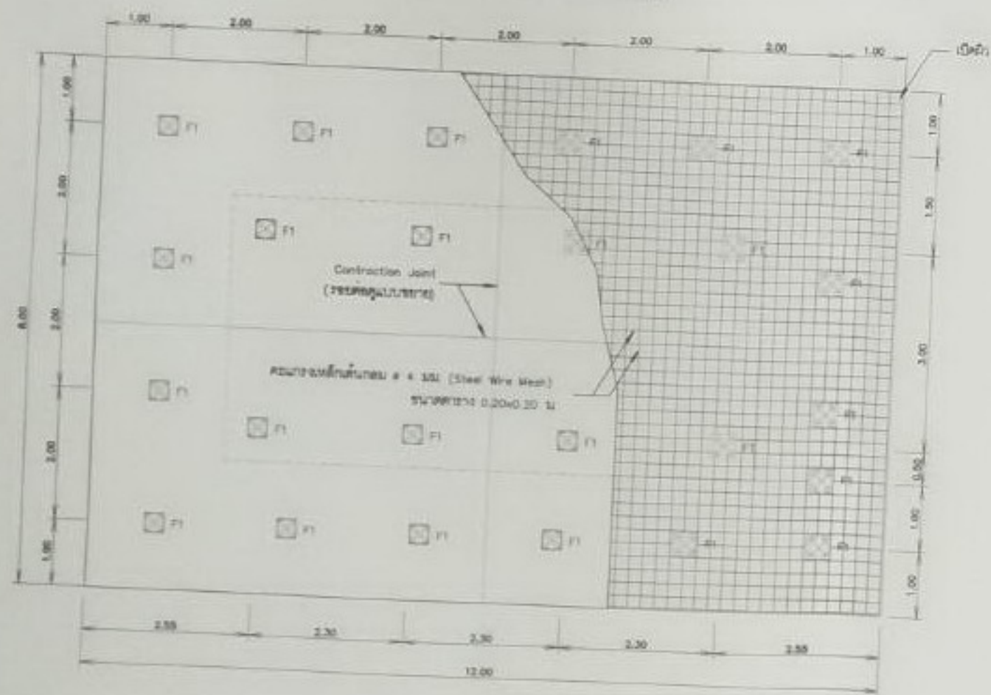
รูปขยายพื้นคอนกรีต ไม่แสดงเสาเข็ม
