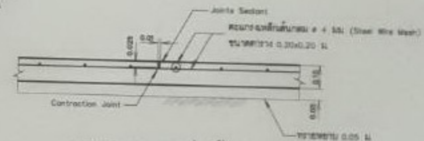
แบบขยายรอยต่อพื้น (Contraction Joint) ไม่แสดงเสาเข็ม
