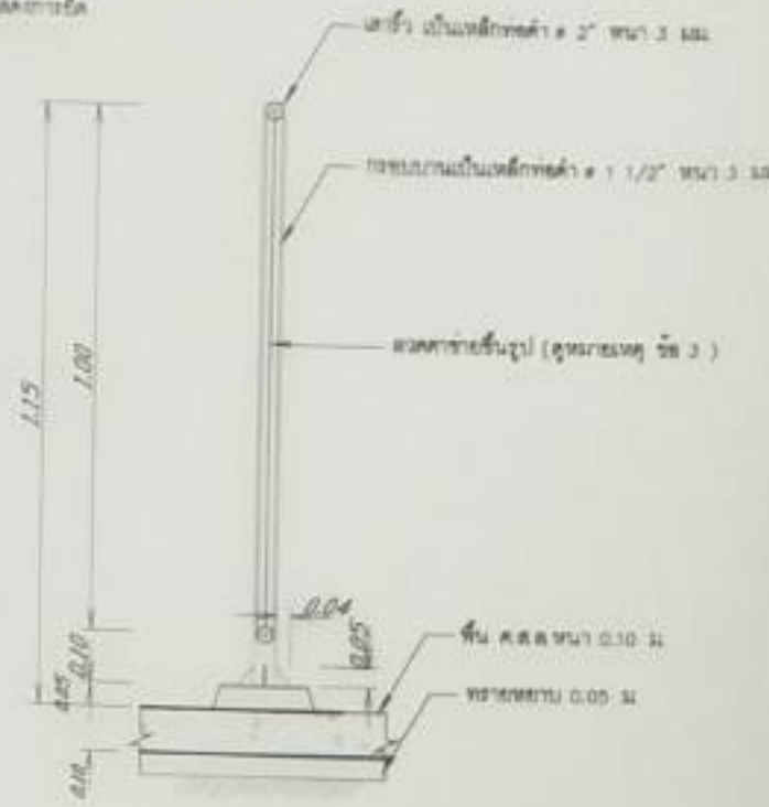
รูปตัด ก-ก
