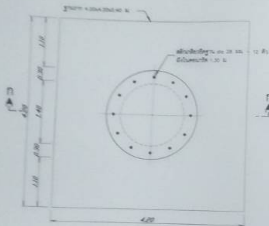
แปลนฐานรากหอดึงสูง (แบบฐานแฉ่ง)
