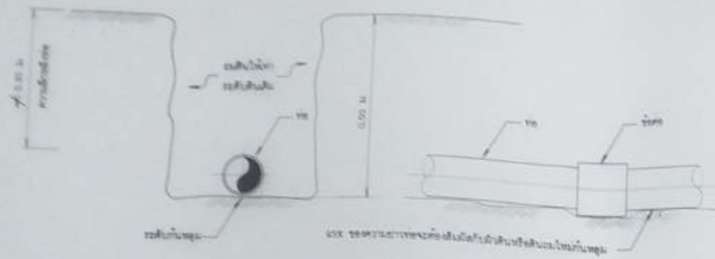
1. แบบการวางท่อทั่วไป ไม่แสดงมาตรฐาน
