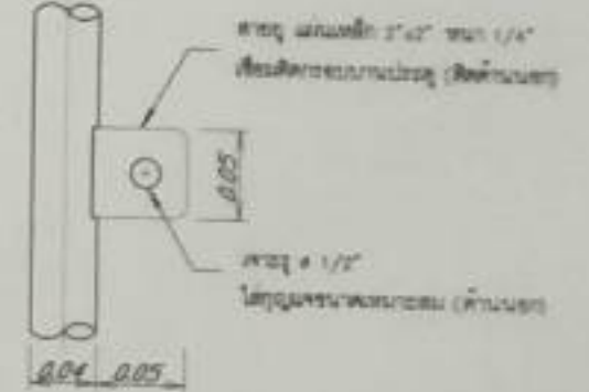
แบบขยายสายยู
