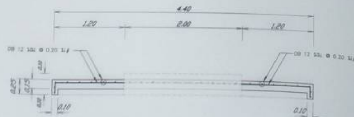
รูปตัด ค-ค
