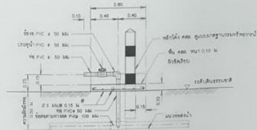
รูปตัด ก - ก แสดงการติดตั้งประตูปปล่อยน้ำ มาตราส่วน 1:20
