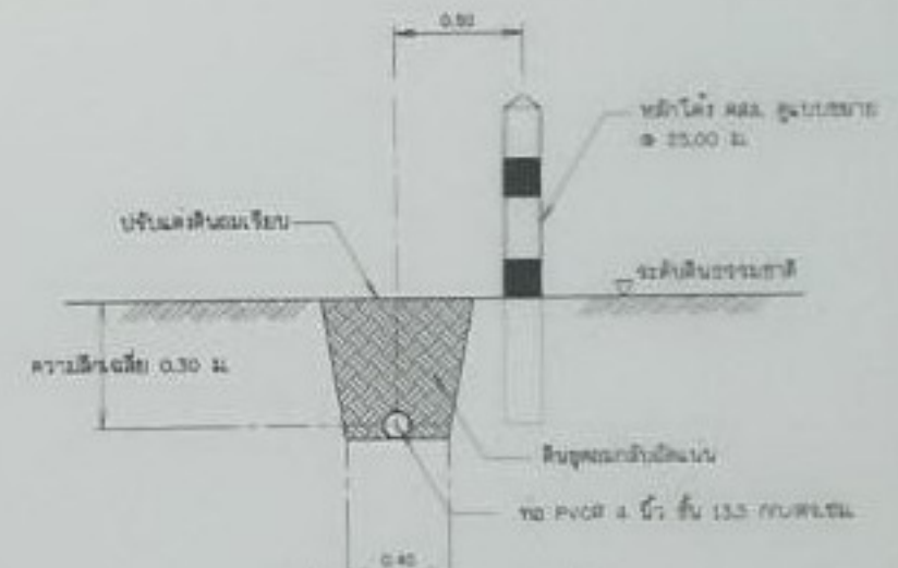
รูปตัดการจุดวางท่อ มาตราส่วน 1:20
