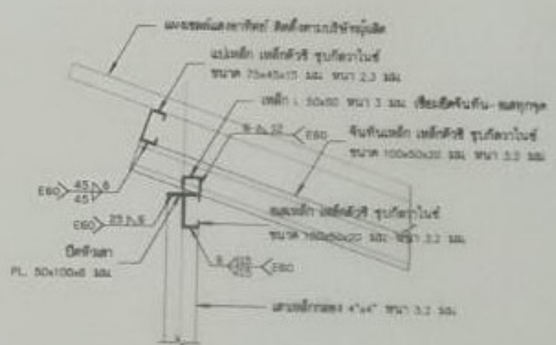
รูปขยาย การติดตั้งโครงหลังคา ไม่แสดงเสาเข็ม
