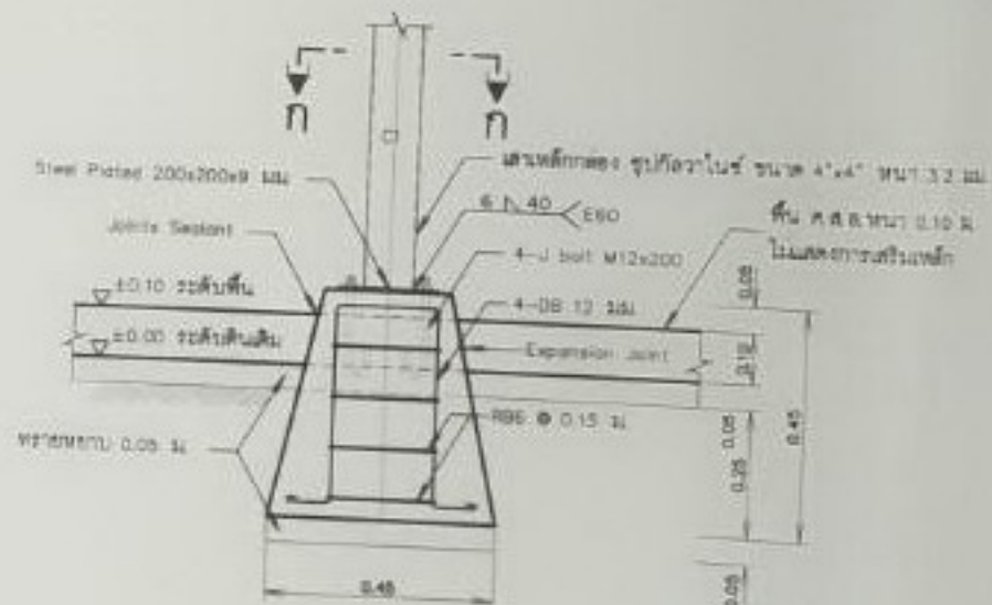
รูปขยายฐานรากโครงสร้างรับแรง F1 (กรณี คสล. ท่อส่งน้ำรูปวงรีชนิด 1) ไม่แสดงเสาเข็ม
