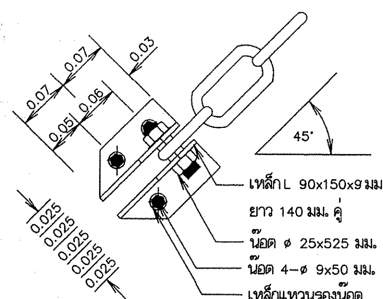
รูปด้านแสดงการยึดติดบ้าน
