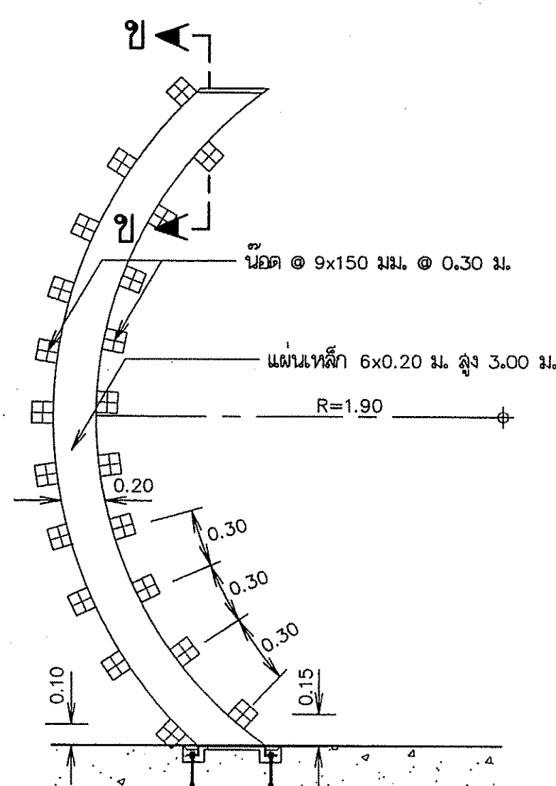
แผนรียงยักน้ำด้านพื้นล่าง มาตราส่วน 1:25
