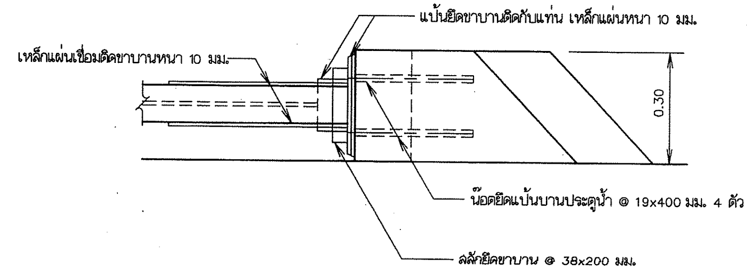
รูปขยาย 2 มาตราส่วน 1:10
