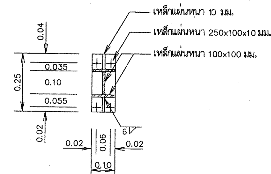
รูปตัดขยาย ค - ค มาตราส่วน 1:10
