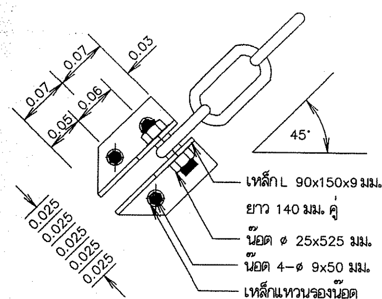
รูปด้านแสดงการยึดขัดบ้าน มาตราส่วน 1:5
