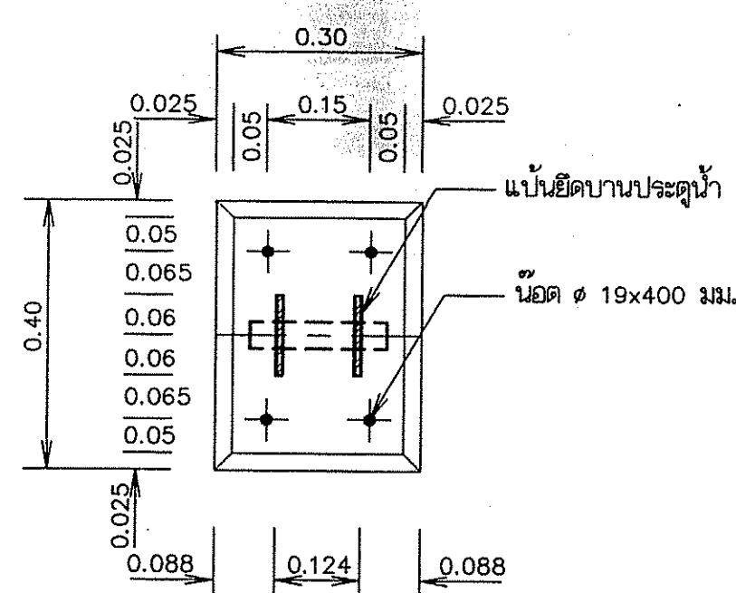
รูปขยายบันไดบ้านประตู มาตราส่วน 1:10
