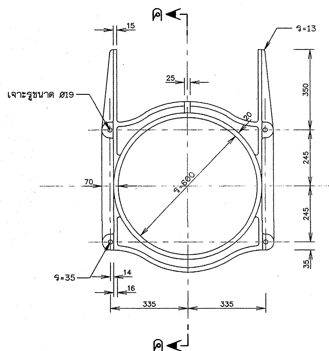
กรอบบาน(เหล็กหล่อ) มาตราส่วน 1:10
