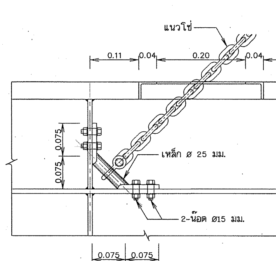
รูปขยาย ตำแหน่งจุดยึดรอกโซ่กับบานระบาย
