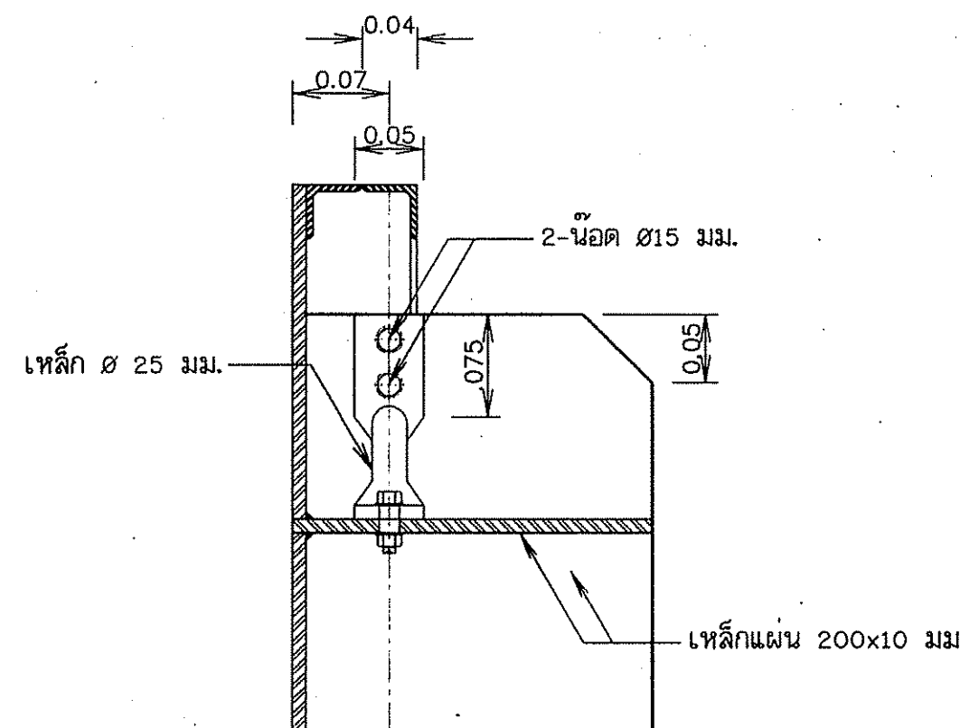
รูปขยาย ตำแหน่งจุดยึดรอกโซ่กับบานระบาย
