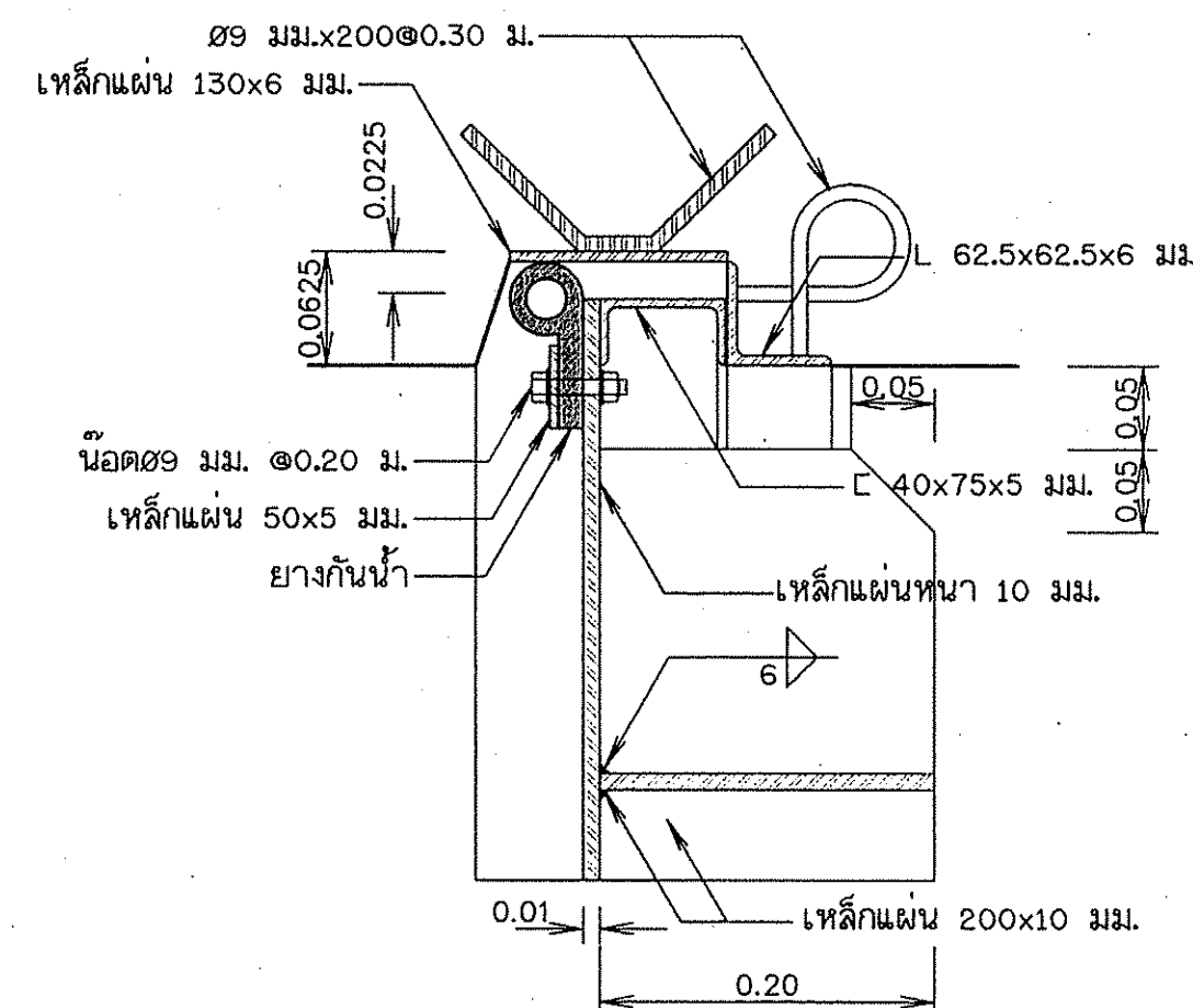
รูปขยายบานระบายด้านติดกำแพง
