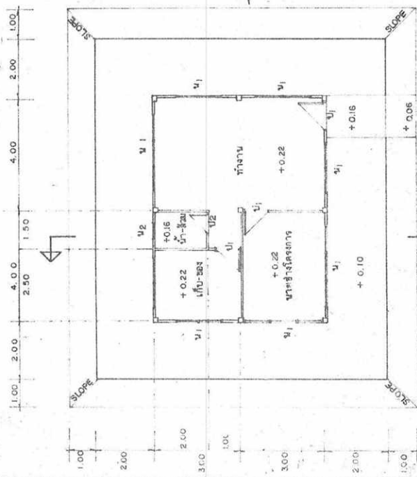
แบบผัง 18100
