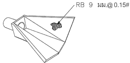
แบบขยายการก่อสร้างอาคารปากท่อ ไม่แสดงมาตราส่วน
