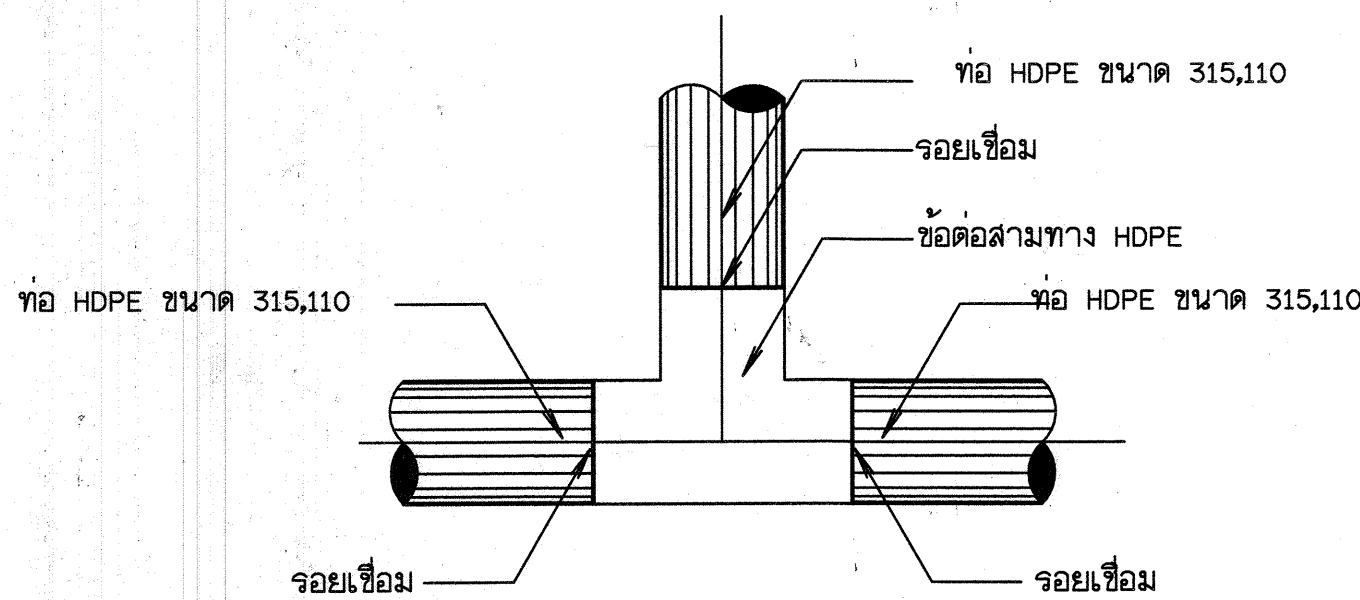
ขยายจุดที่ 1 การบรรจุท่อสามทาง HDPE กับท่อ HDPE
