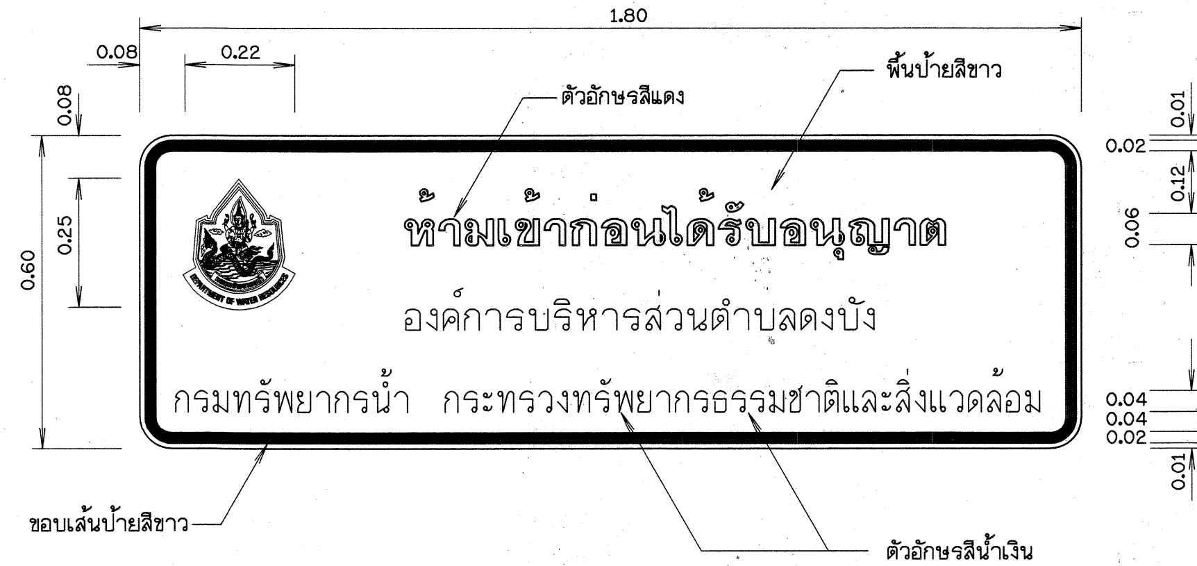
ป้ายแจ้งเตือน มาตรฐาน 1:10
