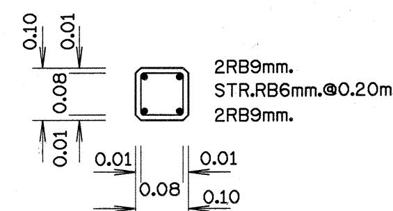
รูปตัด ข - ข มาตรฐาน 1:10
