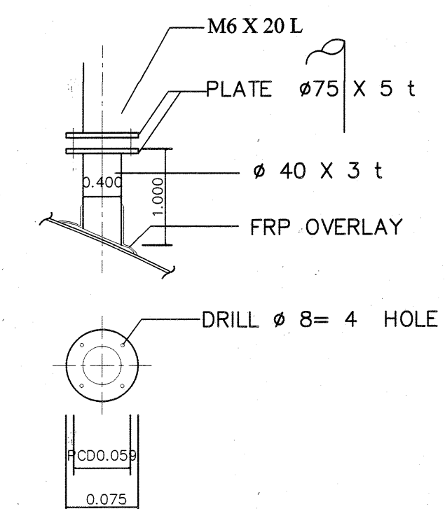
DETAIL B (ขายีครวักนตค)
