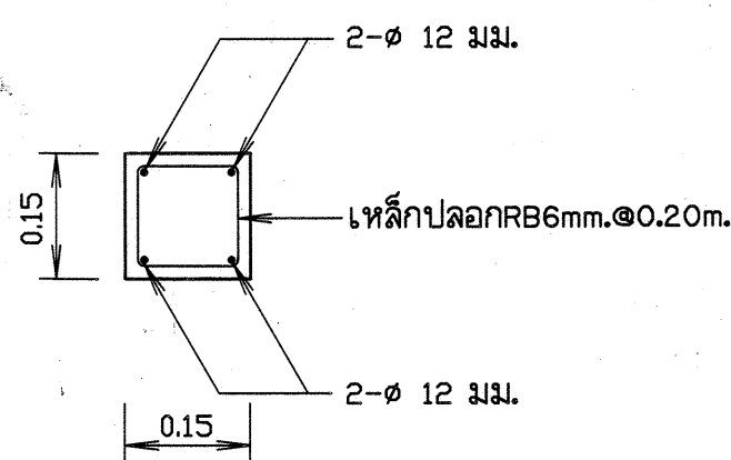
รูปตัด ก - ก มาตรฐาน 1:10
