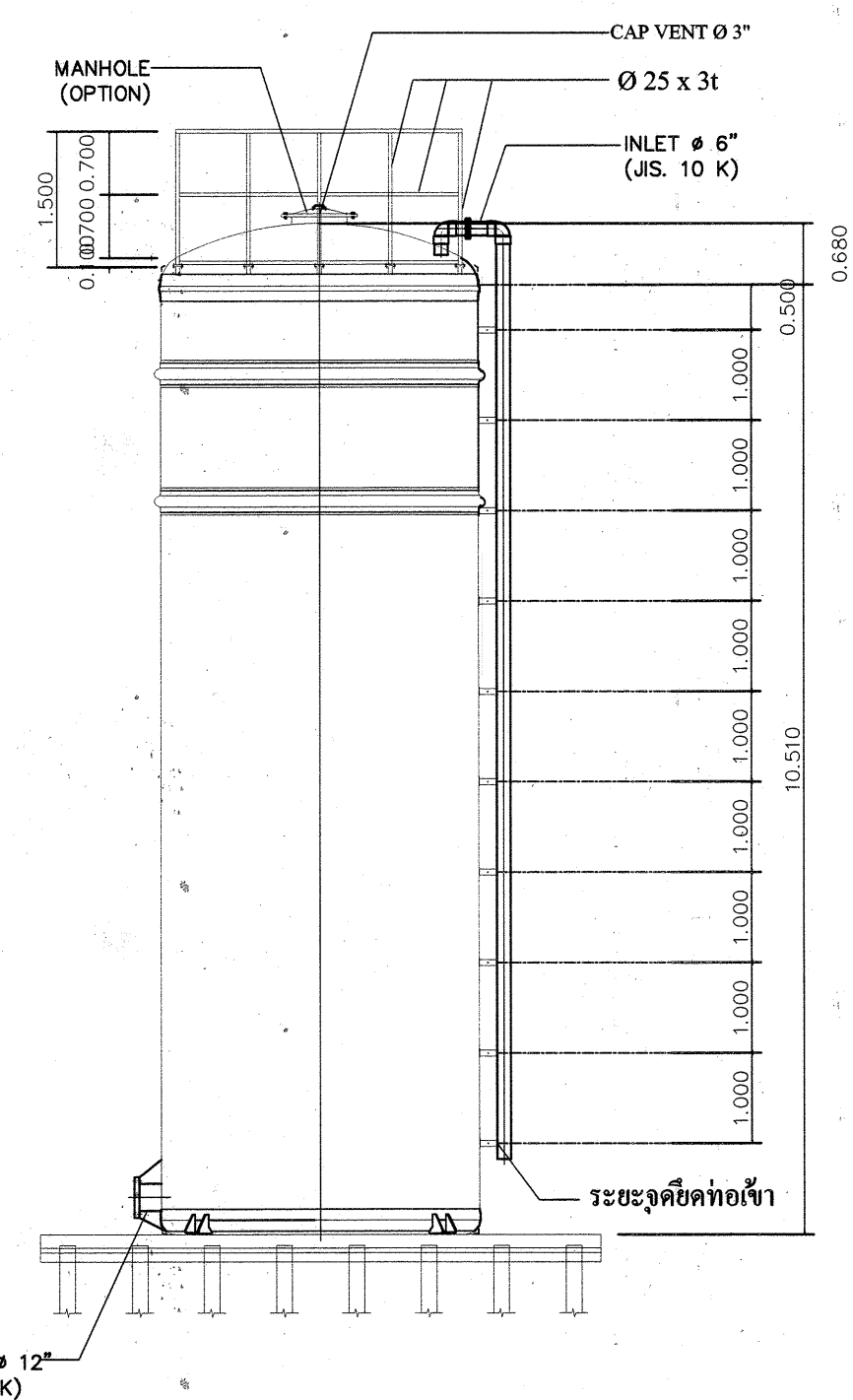
SECTION SCALE : 1:100
