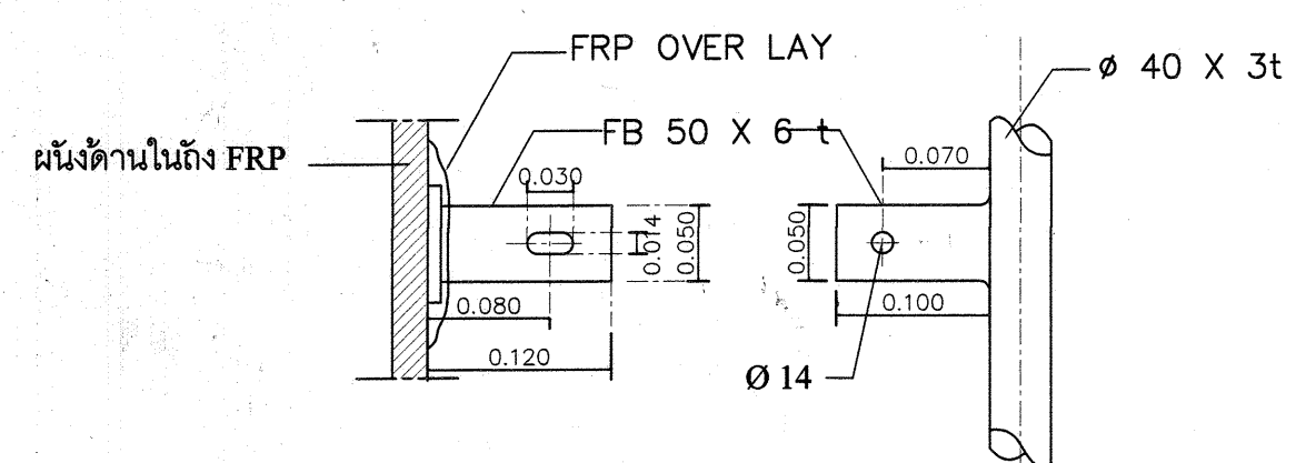
DETAIL A (ขายคัปปันไค)
