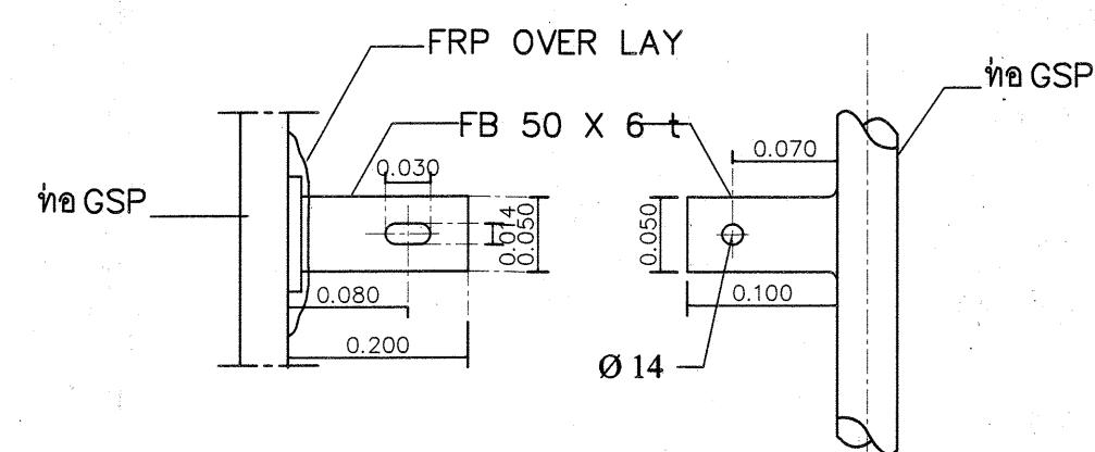
DETAIL C (ข้ายึดท่อ)
