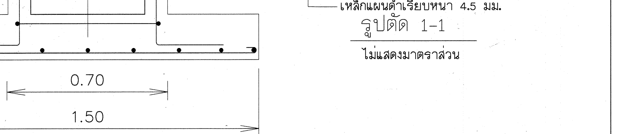
รูปตัด 2-2
