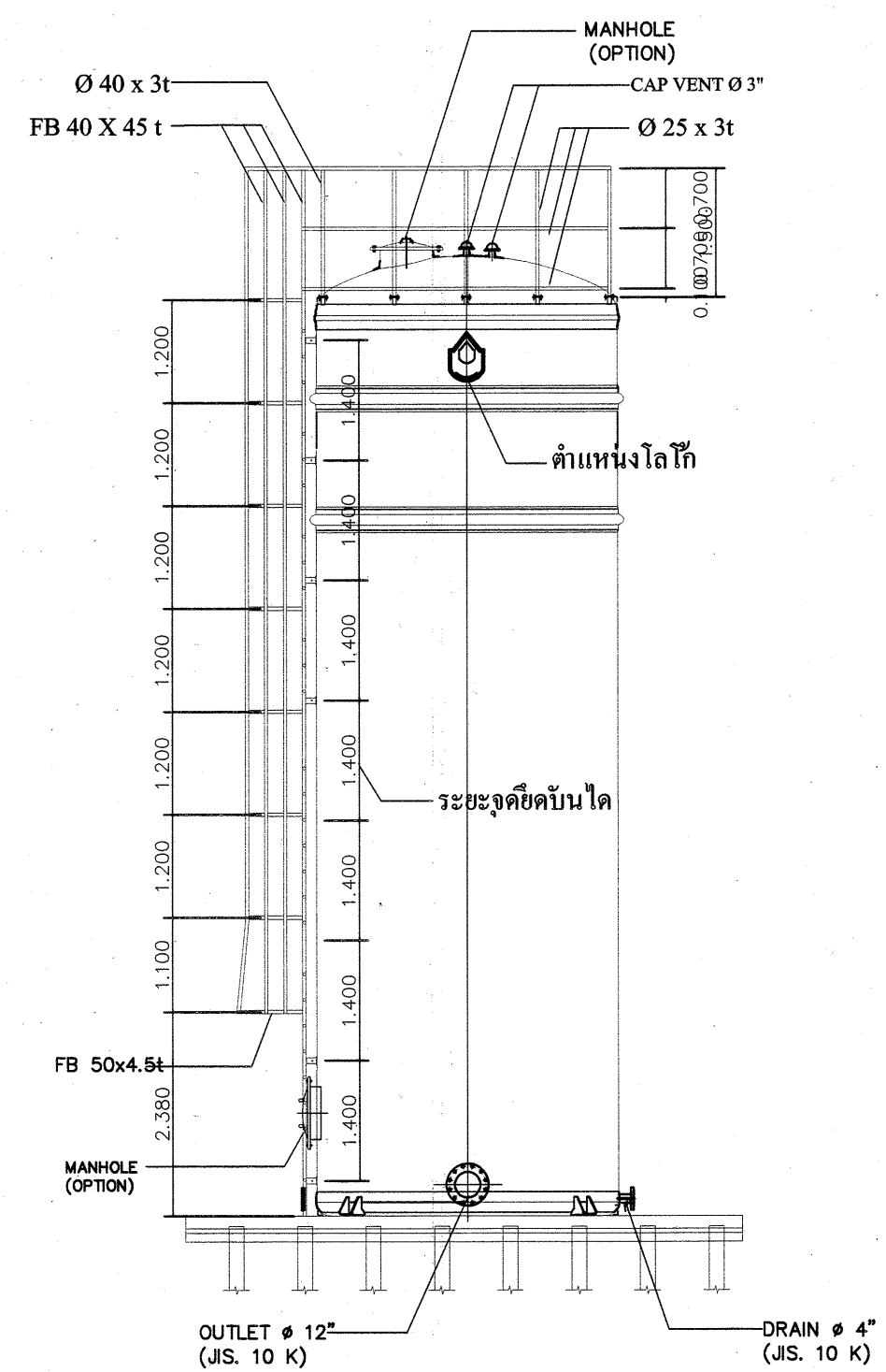
SECTION SCALE : 1:100
