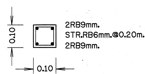
รูปตัด ก - ก มาตรฐาน 1:10
