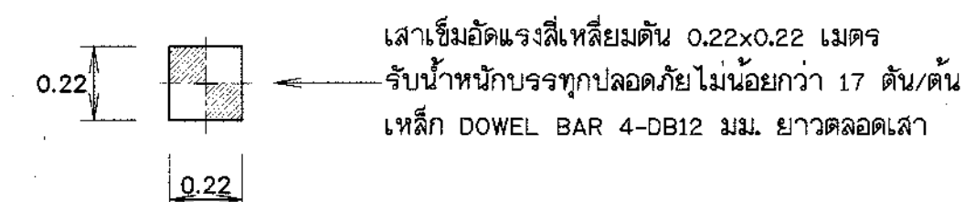
แบบขยายเสาริม P2 มาตราส่วน 1:20
