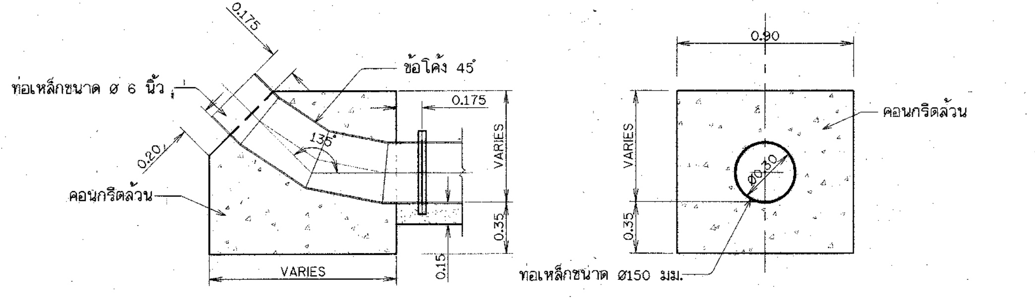
รูปตัด ก1 - ก1
