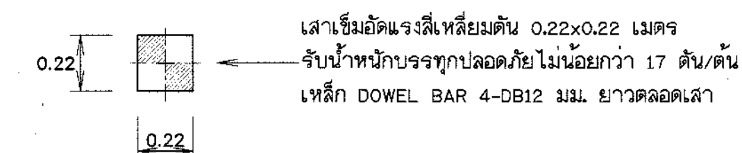
แบบขยายเสาริม P2 มาตราส่วน 1:20
