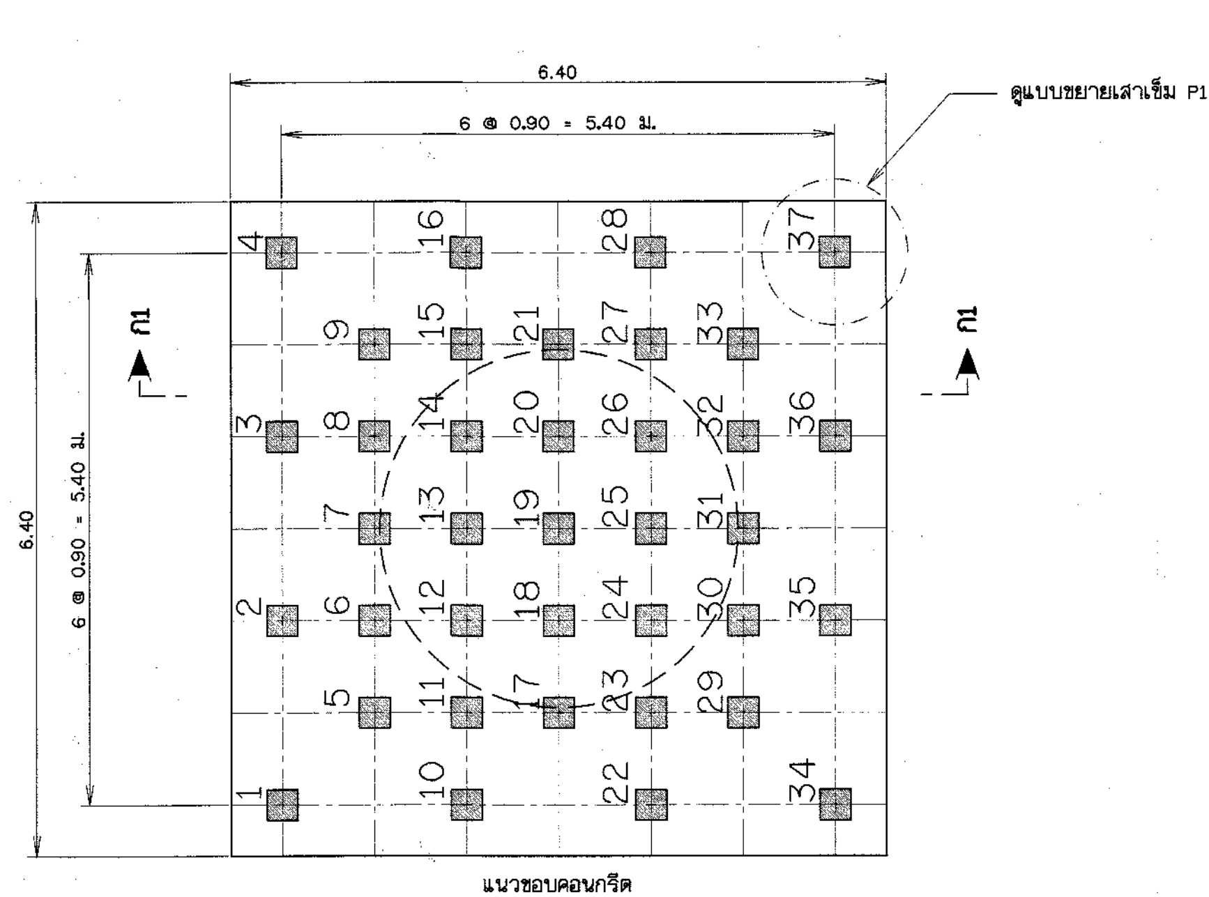
แบบขยายเสาริม P1 มาตราส่วน 1:50
