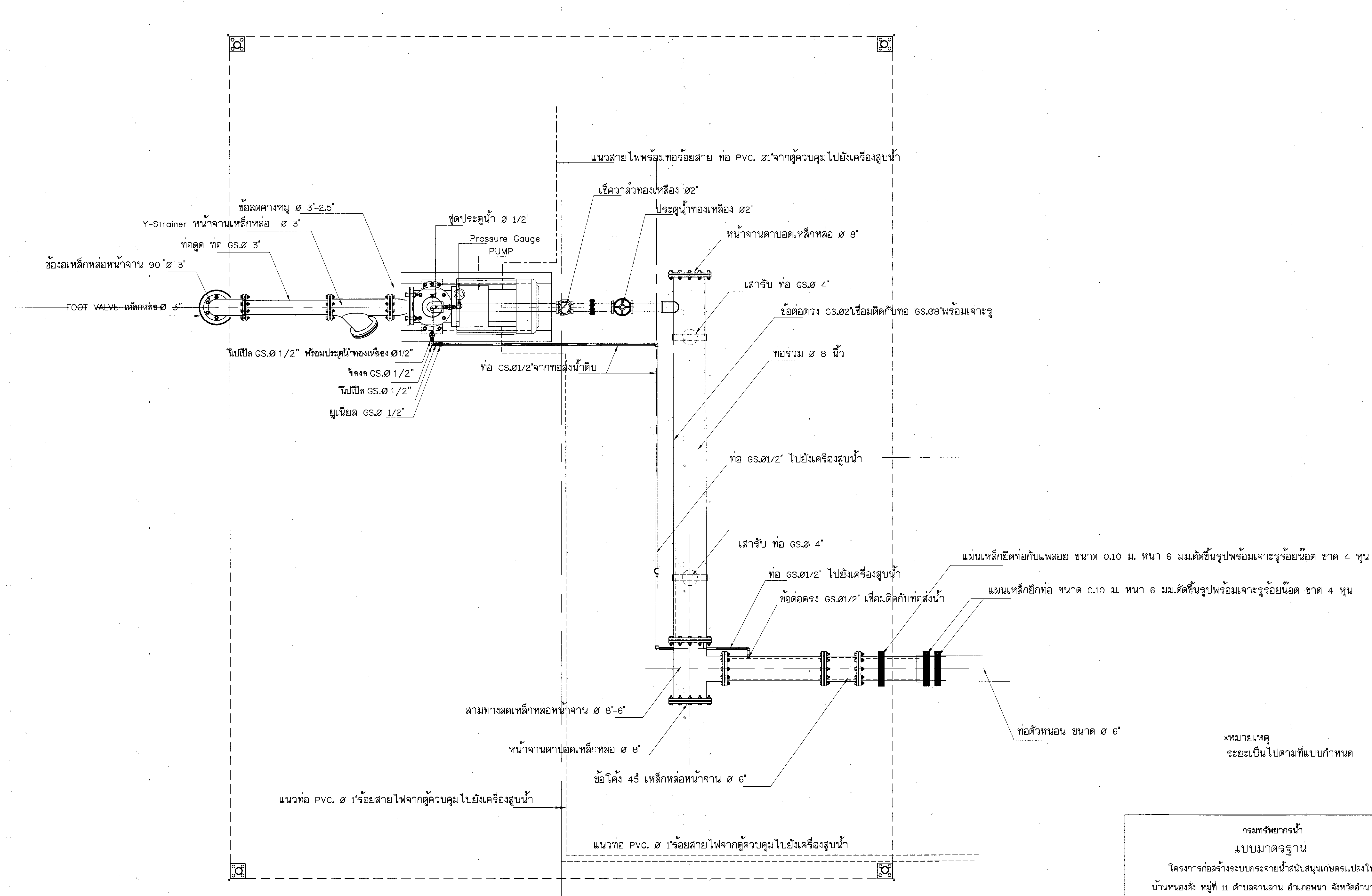
แผนขยายการติดตั้งเครื่องสูบน้ำ ไม่แสดงมาตราส่วน
