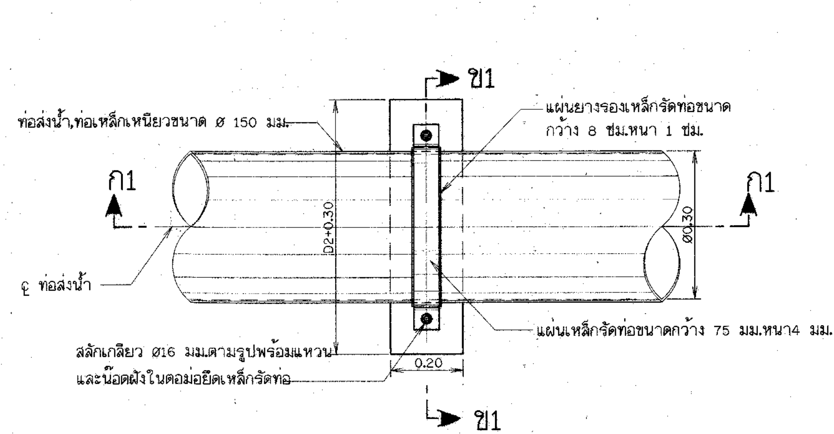
แปลนการยึดท่อ
