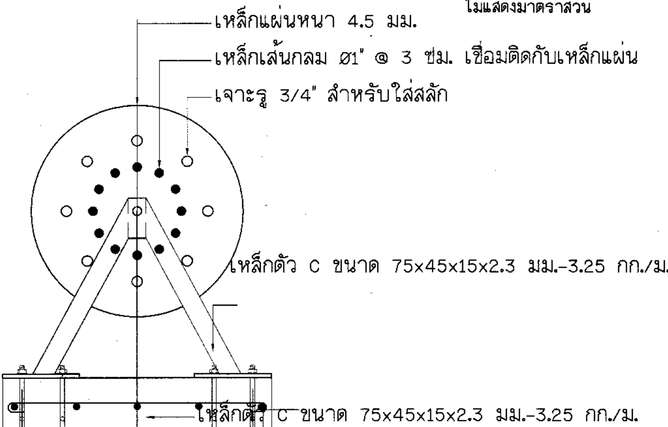
แบบขยาย "ด"
