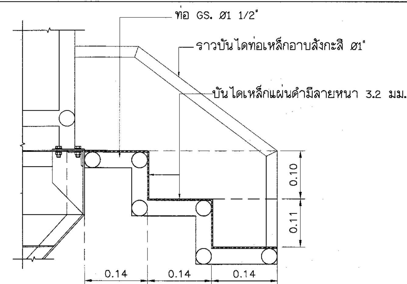
แบบขยาย "ด"
