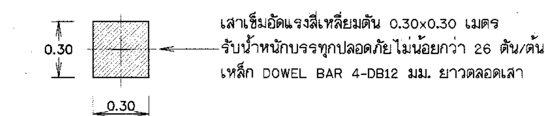
แบบขยายเสาริม P1 มาตราส่วน 1:20
