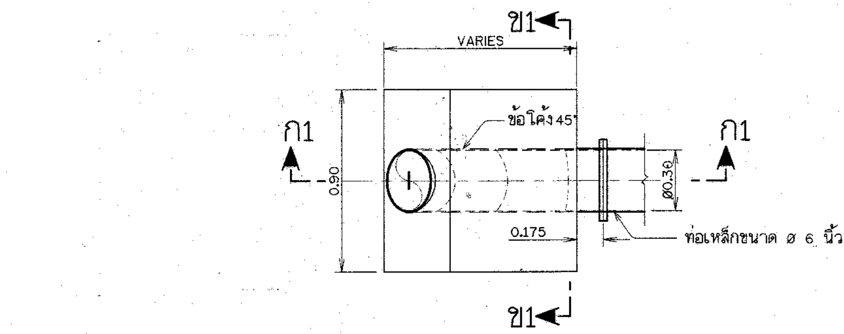
แปลน THRUST BLOCK
