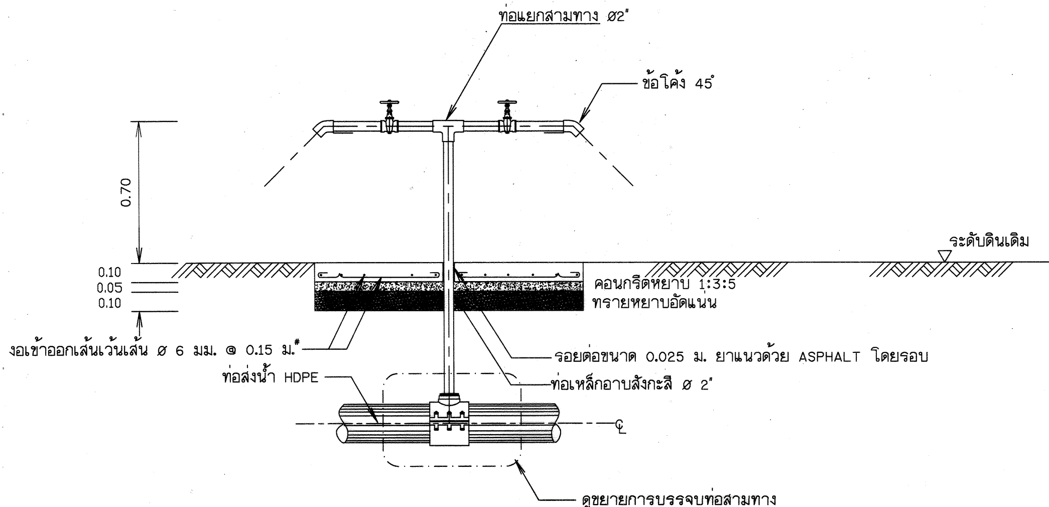
ขยายจุดที่ 1 การบรรจุท่อสามทาง HDPE กับท่อ HDPE
