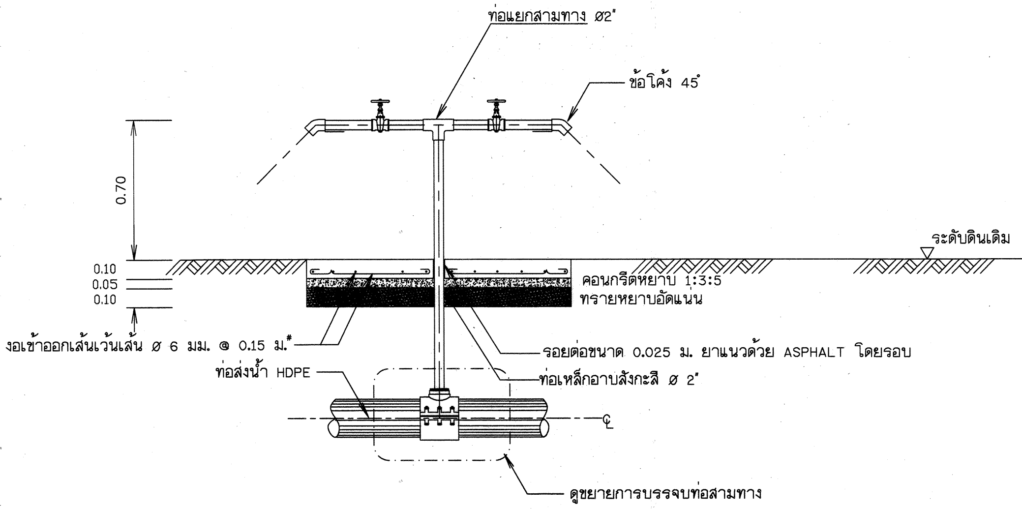
ขยายจุดที่ 1 การบรรจุท่อสามทาง HDPE กับท่อ HDPE ไม่แสดงมาตราส่วน
