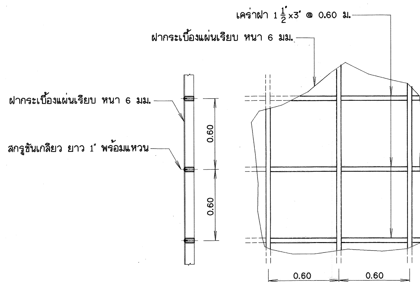
รูปขยายเค้า , ฝ้า มาตราส่วน 1:20
