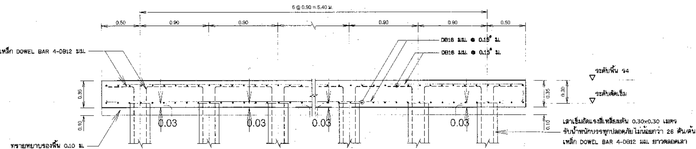
รูปตัด G1 - G1 มาตราส่วน 1:20
