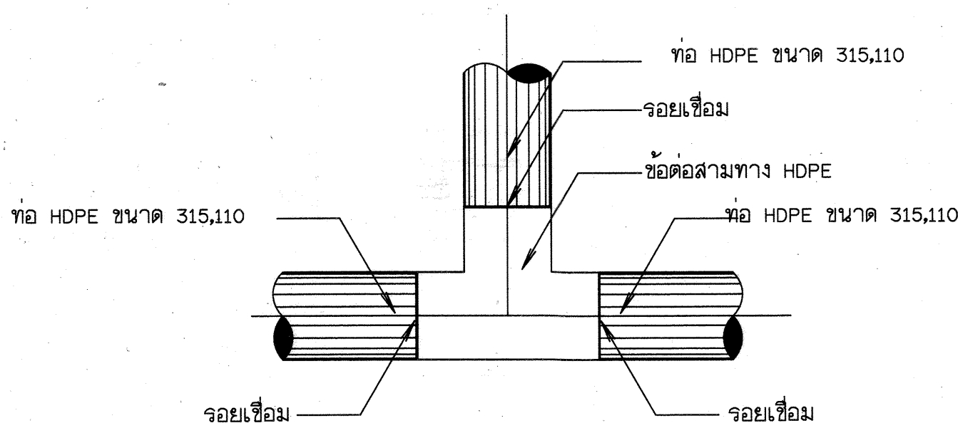
ขยายจุดที่ 1 การบรรจุท่อสามทาง HDPE กับท่อ HDPE ไม่แสดงมาตราส่วน
