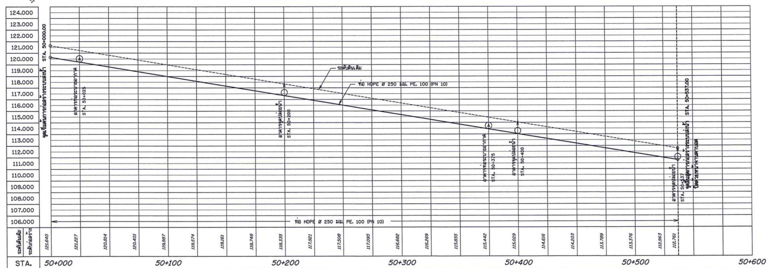
รูปตัดตามแนวยาว STA. 50+000 - 50+537
