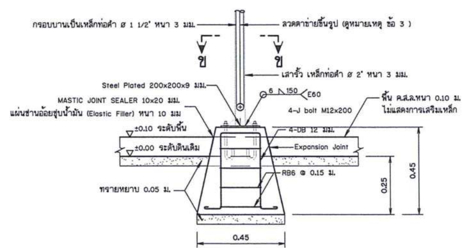
รูปขยายฐานรากโครงสร้างรับแผง F2 (ต่อม่อ คสล. หล่อสำเร็จรูปพร้อมติดตั้ง) ไม่แสดงมาตราส่วน
