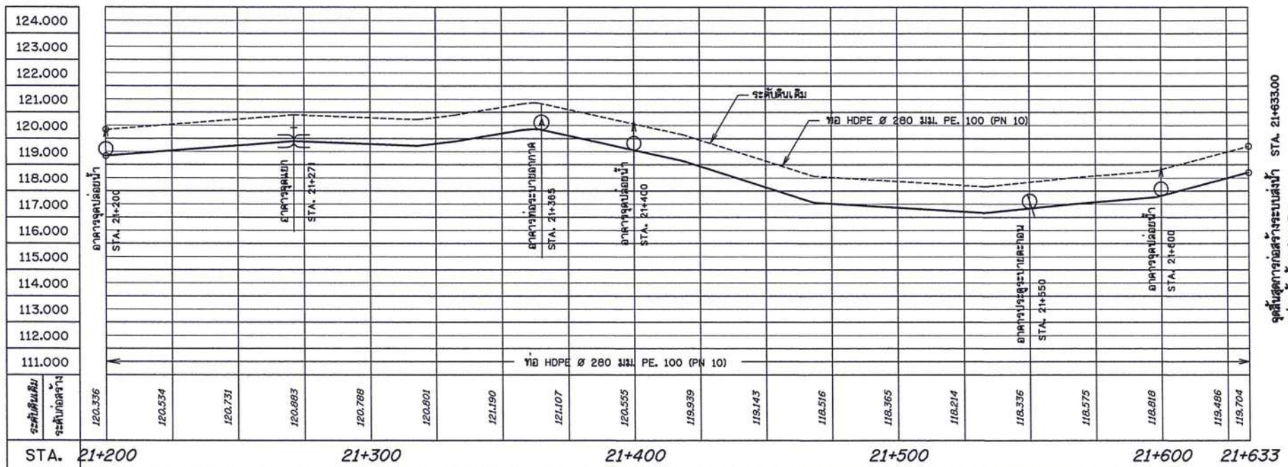
แปลนระบบส่งน้ำ STA. 21+200 - 21+633 มาตรฐาน 1:1,000
