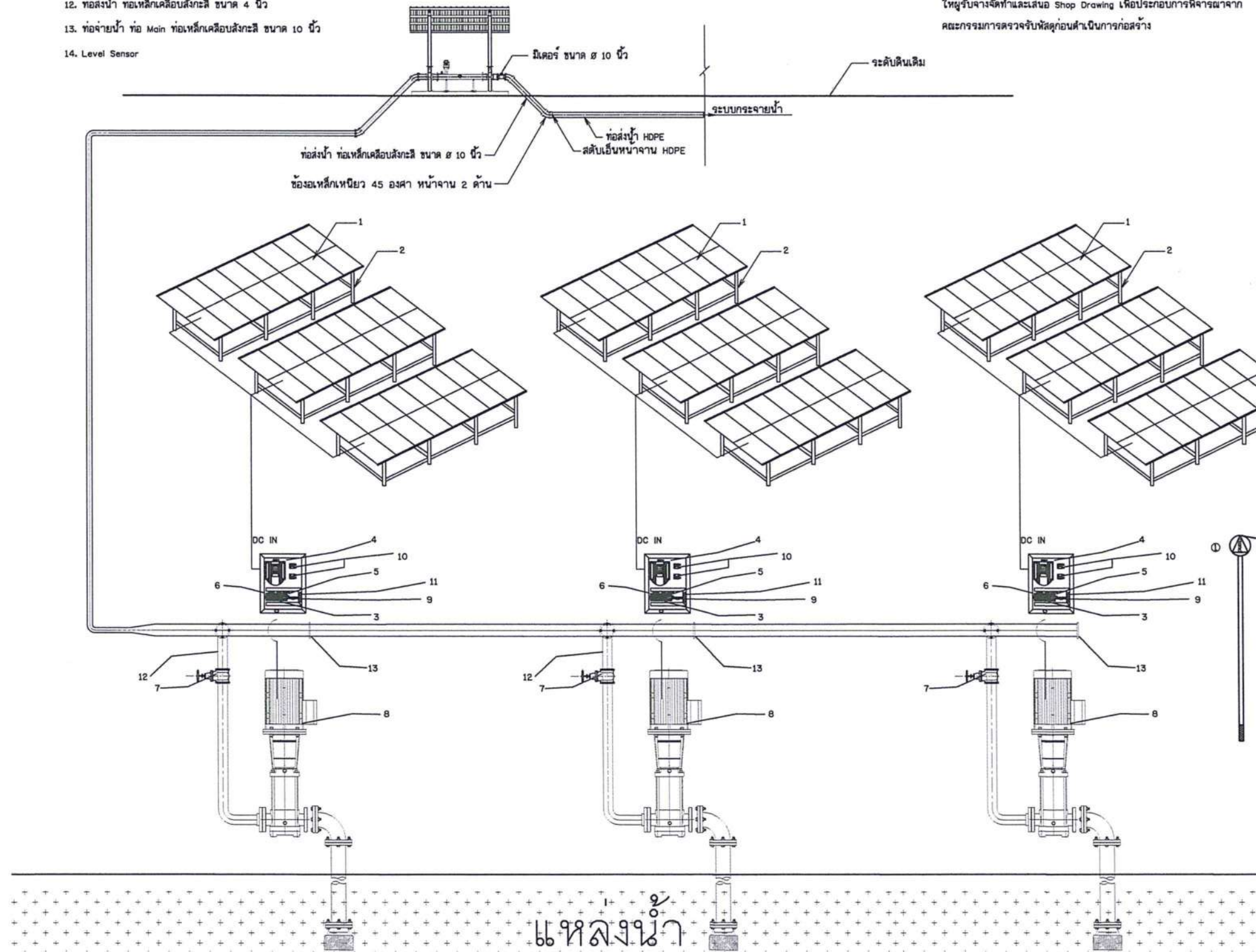
แบบระบบกระจายน้ำด้วยพลังงานแสงอาทิตย์
