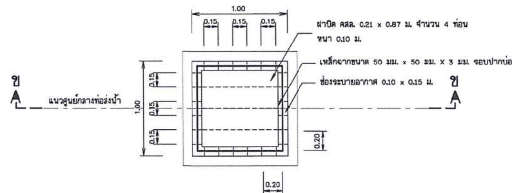
แปลนอาคารท่อระบายอากาศ
