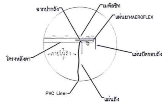
แบบขยาย 3-จุดยึดหลังคาบับแผ่นดัง Scale NTC.
