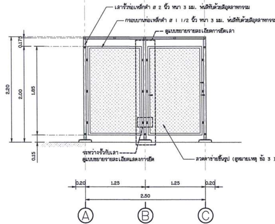
แบบขยายหัว 2 ไม่แสดงมาตราส่วน
