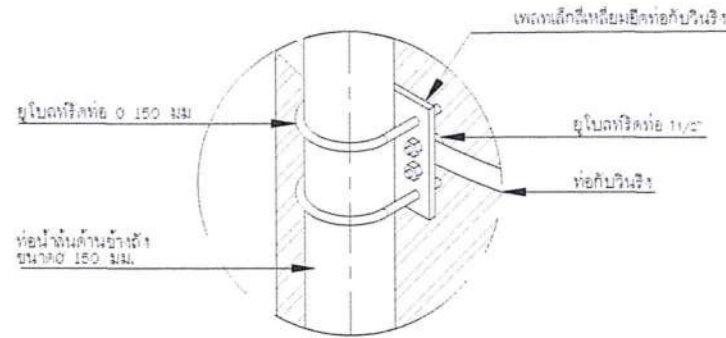
แบบขยาย 2-รูปแบบการประกอบแผ่นดัง Scale NTC.
