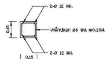
รูปตัด ก - ก ๙๑๙๙๑๐ 1:10
