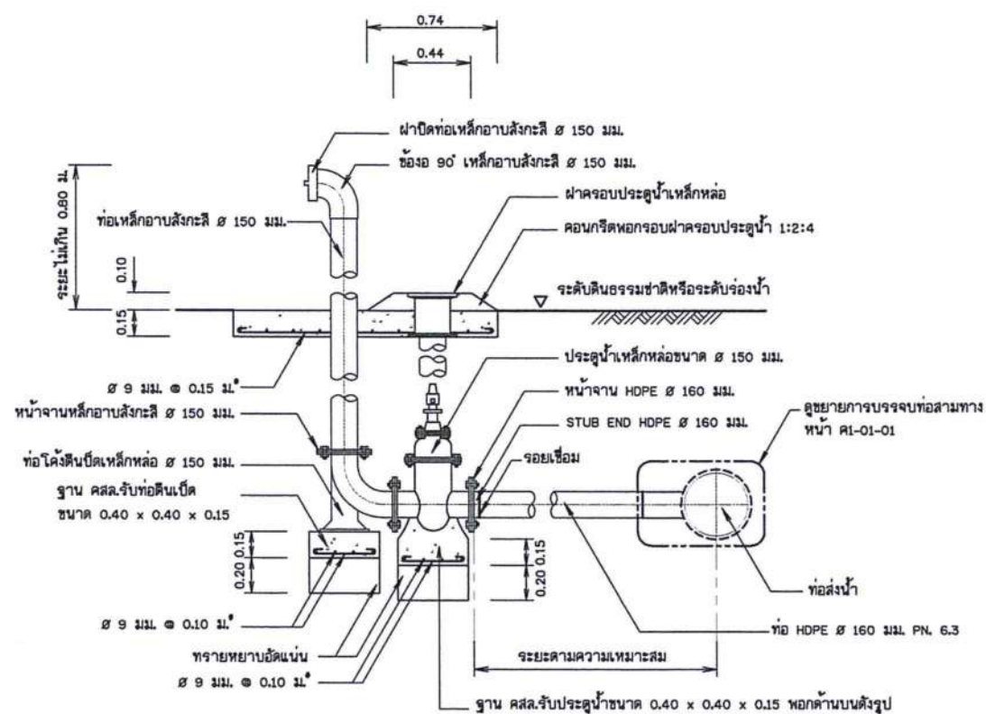
รูปตัด ก - ก แสดงการติดตั้งประติรูประบายตะกอน
