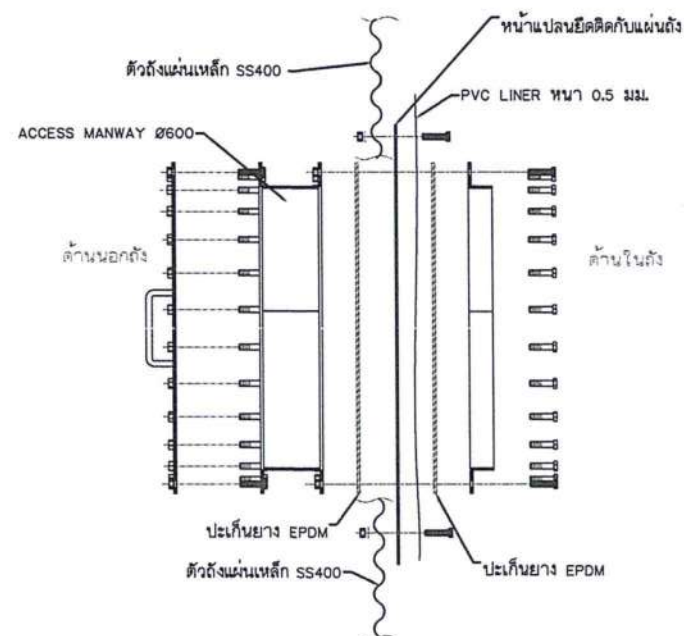
แบบขยายประตูตรวจสอบบ่ารุงรักษา Scale NTC.
