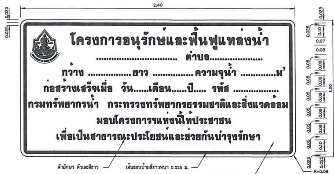
ป้ายโครงการ ๙๑๙๙๑๐ 1:10
