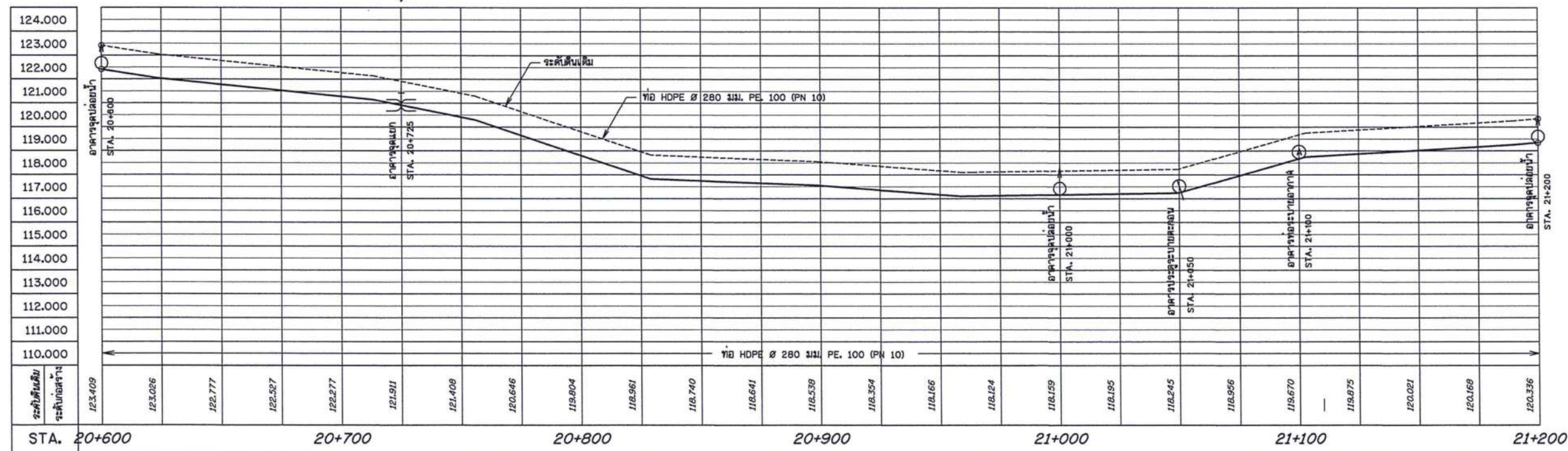
รูปตัดตามแนวยาว STA. 20+600 - 21+200
