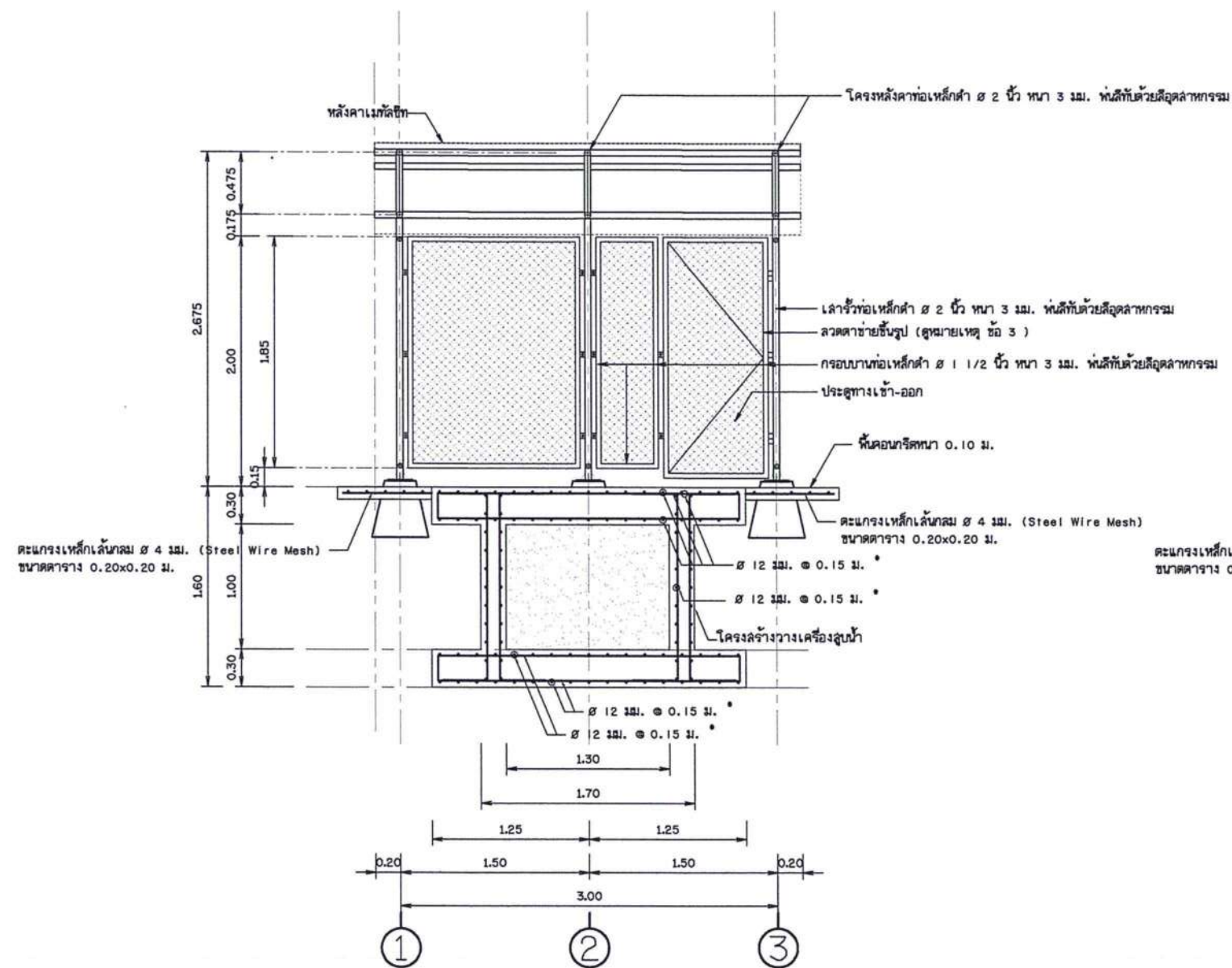
รูปตัด ก - ก ไม่แสดงขนาดจั่ววน
