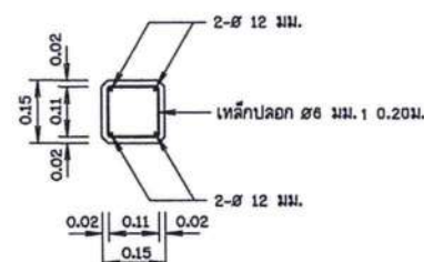
รูปตัด ข - ข ๙๑๙๙๑๐ 1:10
