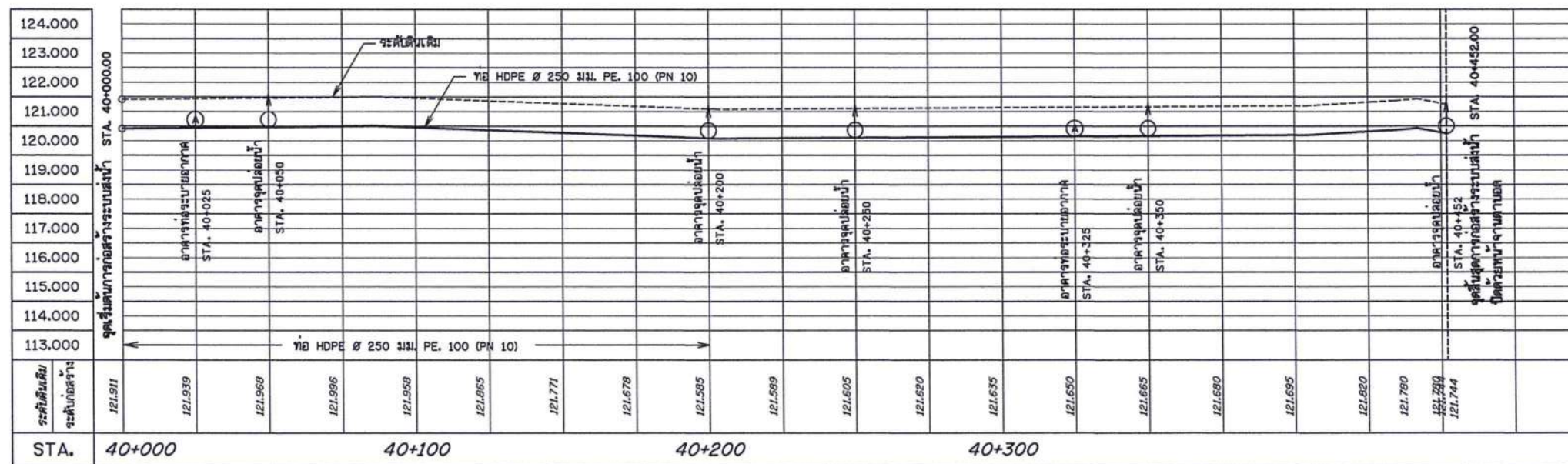
รูปตัดตามแนวยาว STA. 40+000 - 40+452
