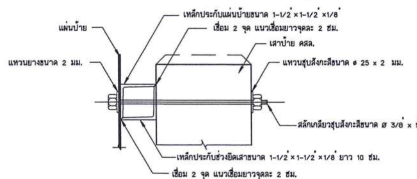
รูปตัดขยายการยึดแผ่นป้ายและเสา ๙๑๙๙๑๐ 1:20
