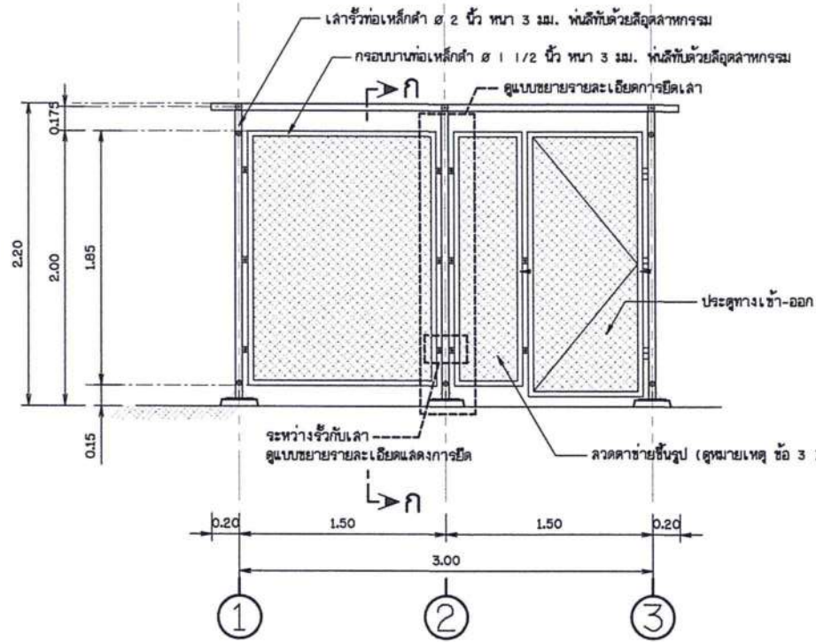
แบบขยายหัว 1 ไม่แสดงมาตราส่วน
