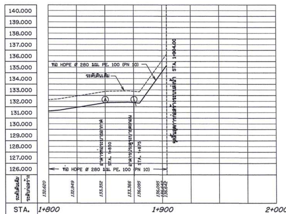
รูปตัดตามแนวยาว STA. 1+800 - 1+904
