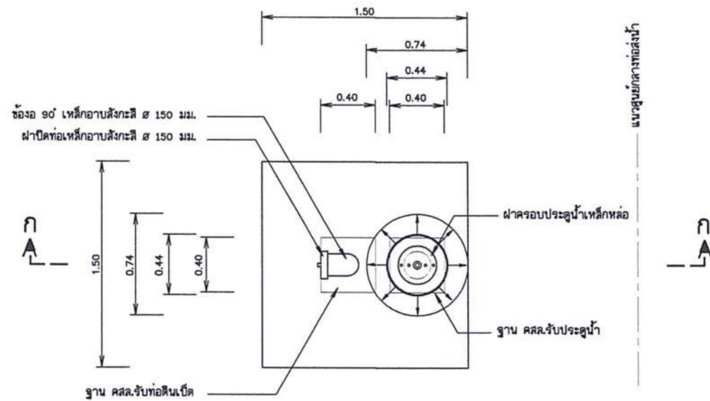
แปลนอาคารประติรูประบายตะกอน
