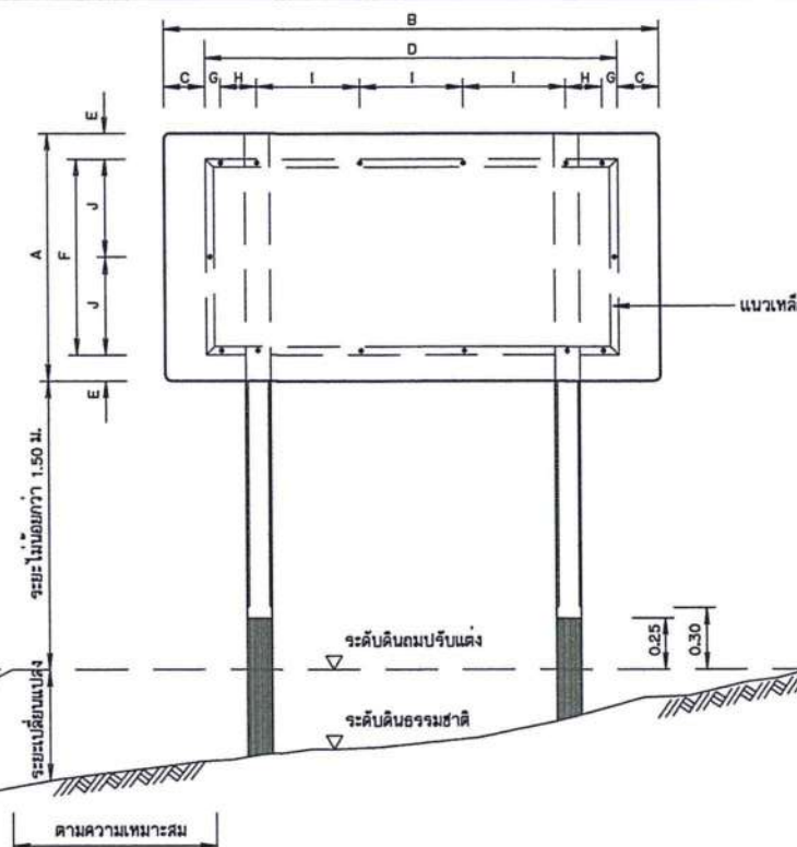
รูปแสดงการประกอบแผ่นป้าย ๙๑๙๙๑๐ 1:20
