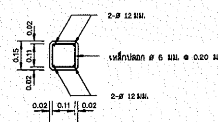
รูปตัด ข-ข ไม้เอกมาควบด้วย
