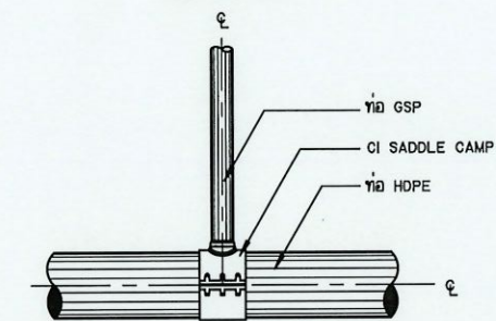
การบรรจุท่อสามทาง HDPE กับท่อ GSP แบบ CI SADDLE CLAMP (สำหรับอาคารจุดปล่อยน้ำ อาคารประจวบประจวบตะกอน อาคารท่อระบายอากาศ กรณีท่อส่งน้ำขนาดเส้นผ่านศูนย์กลางน้อยกว่าหรือเท่ากับ 315 มม.)
