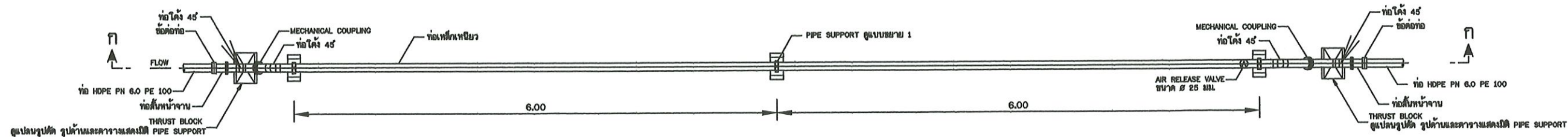
แปลนท่อข้ามคลอง มาตราส่วน 1:25
