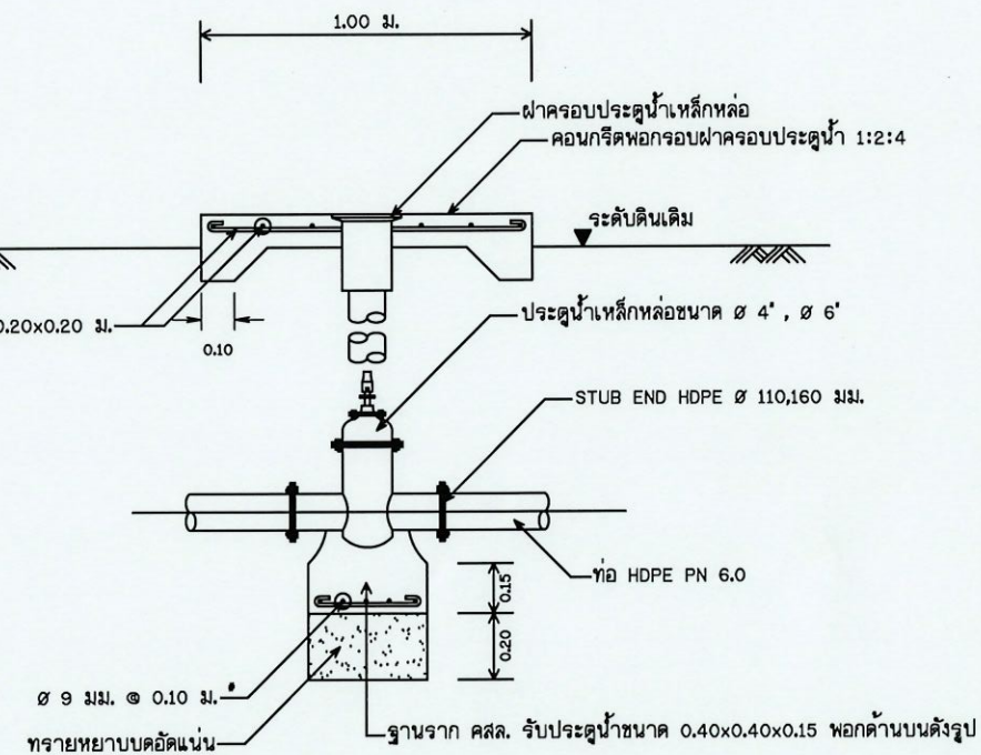
รูปตัด ค - ค แสดงการติดตั้งประตุน้ำใต้ดิน มาตราส่วน No Scale
