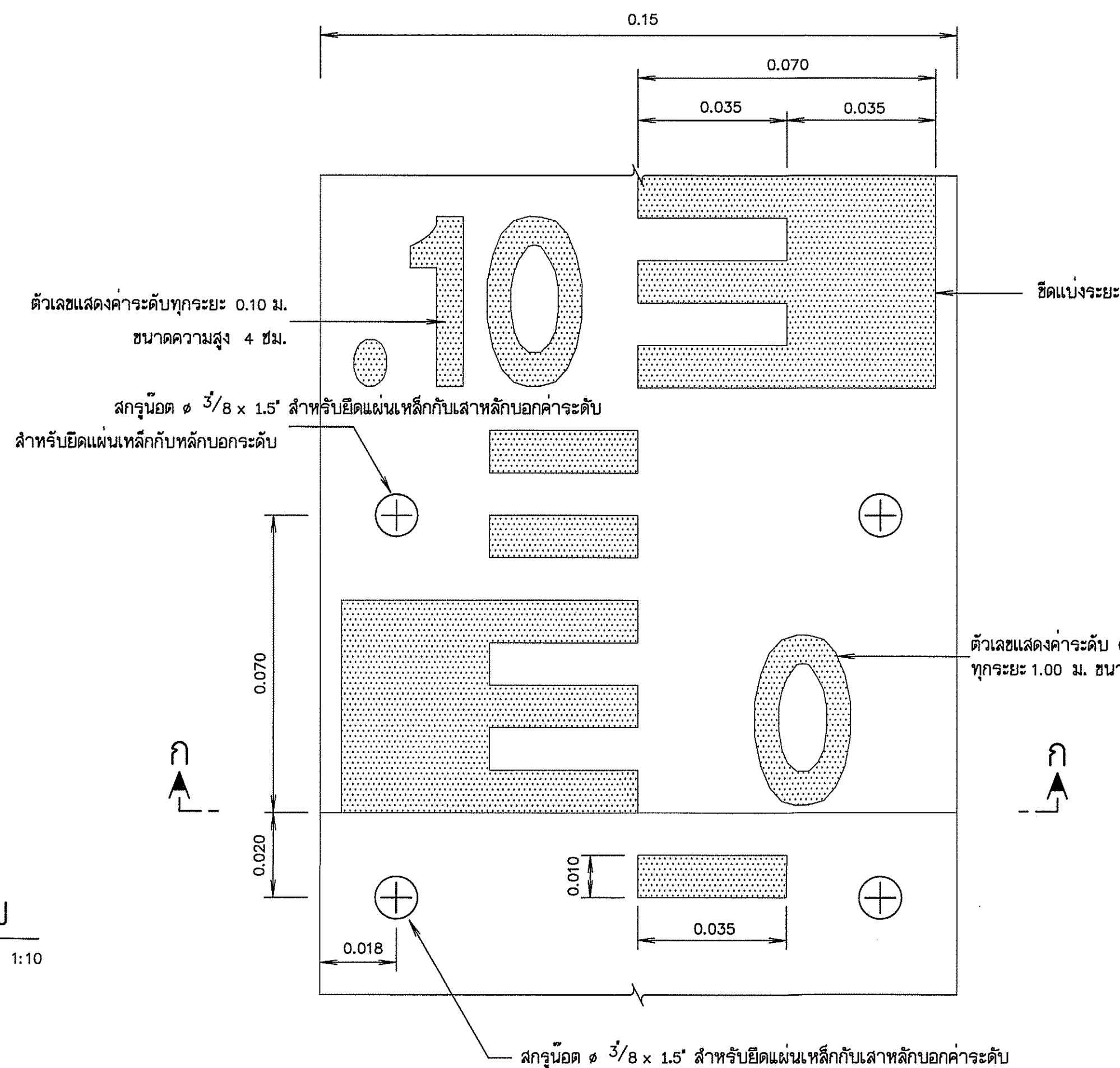
แผ่นเหล็กบอกระดับ
