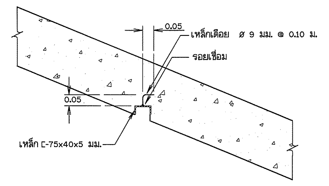
แบบขยาย 2 มาตราส่วน 1:10
