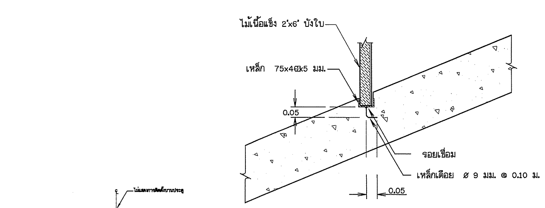
แบบขยาย 1 มาตราส่วน 1:10
