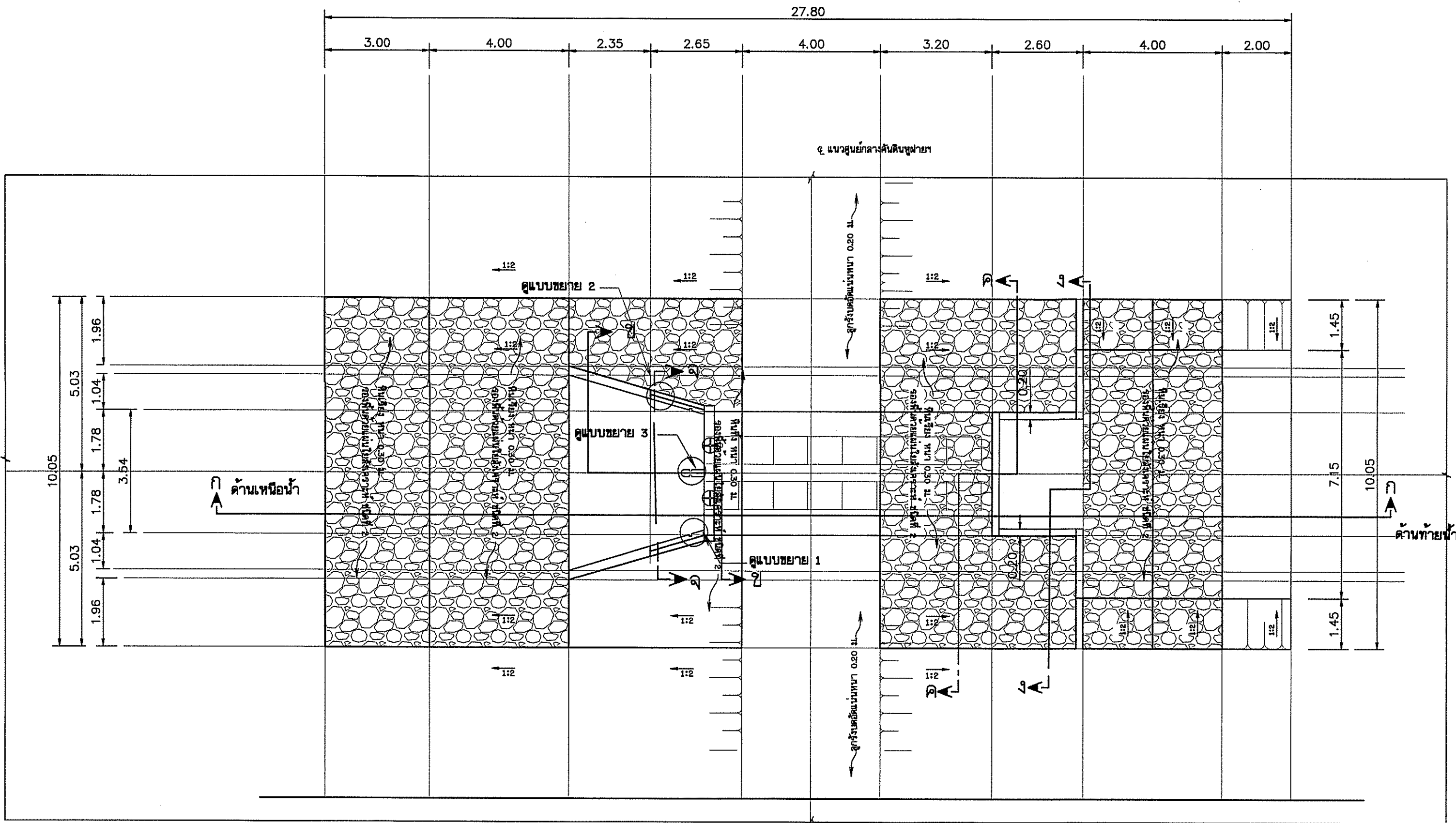
แปลนอาคารบังคับน้ำแบบทอกลม ท่อ 2 แถว (สำหรับฝายน้ำล้น)
