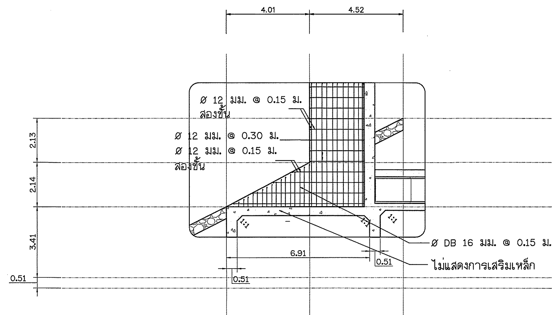
แสดงการเสริมเหล็กกำแพงด้านข้างอาคารเหนือน้ำ ไม่แสดงมาตราส่วน
