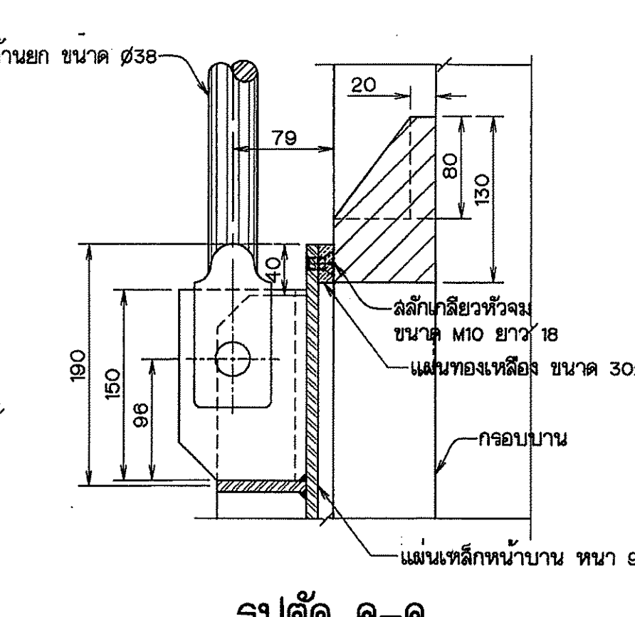
รูปตัด ค-ค
