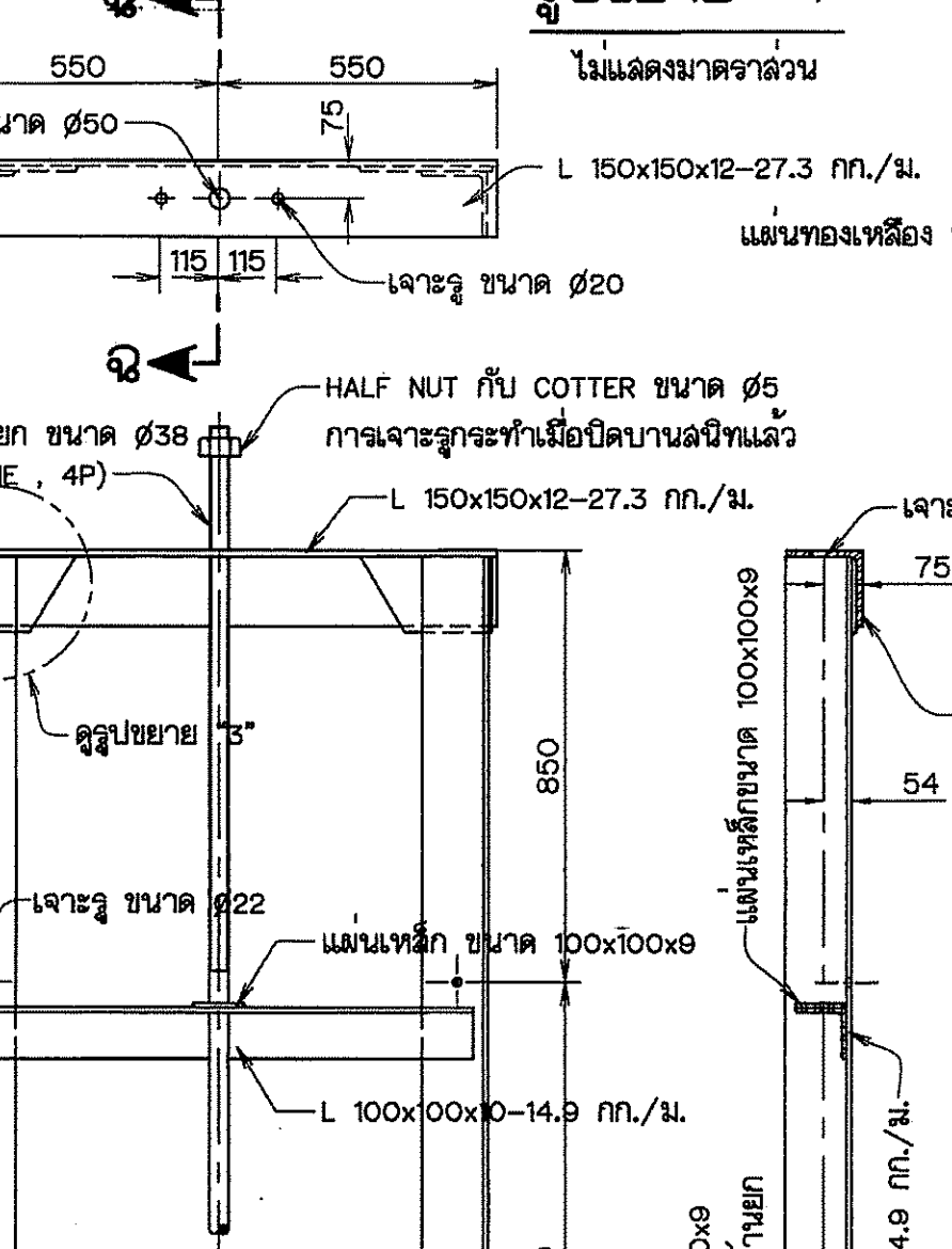
รูปขยาย "4"
