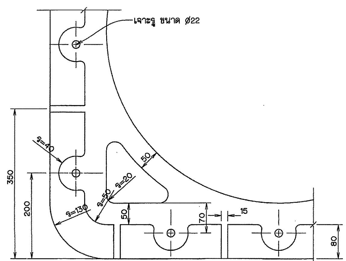
รูปขยาย "1"
