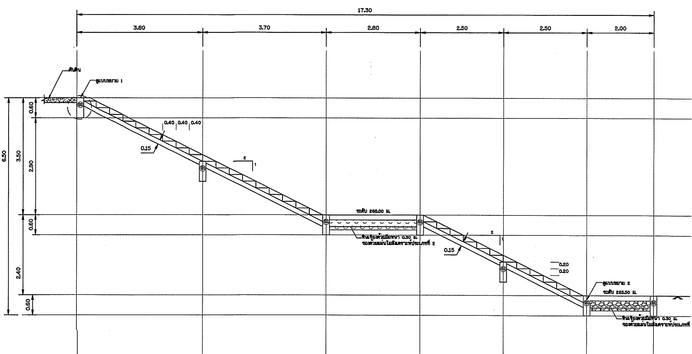
แนวตัด A-A มาตราส่วน 1 : 100
