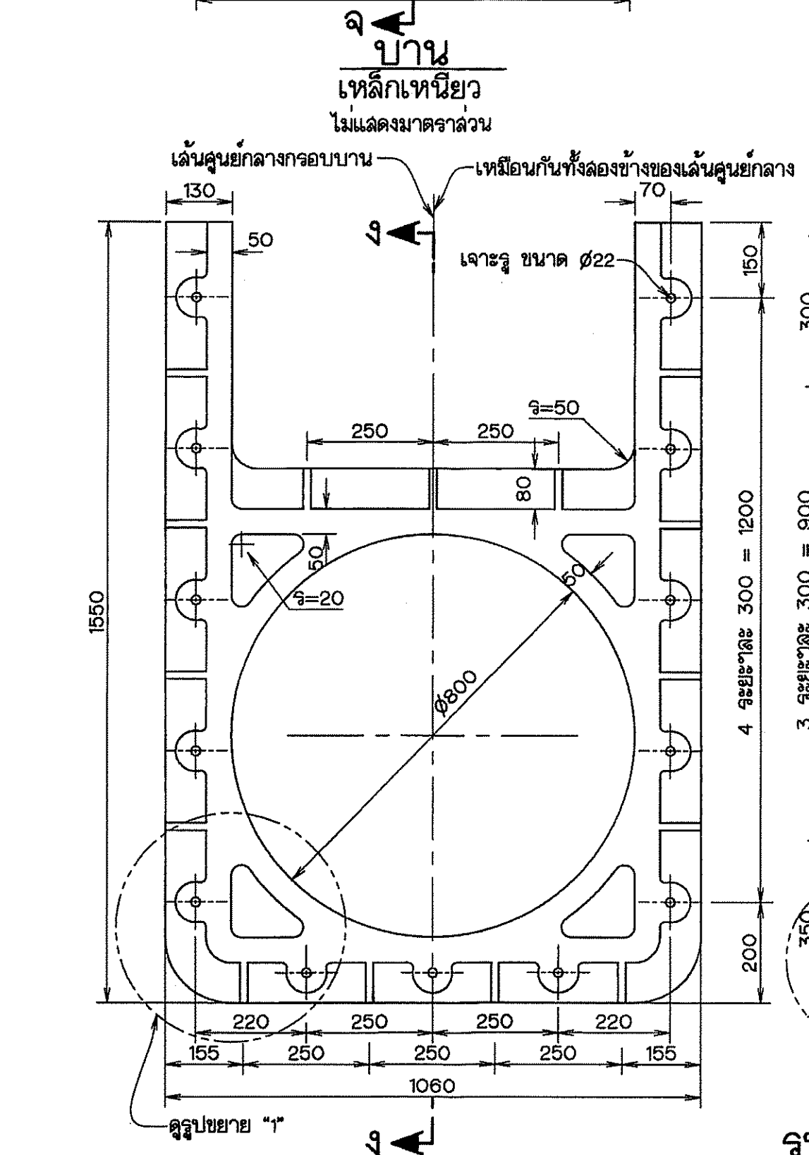
รูปขยาย "1"
