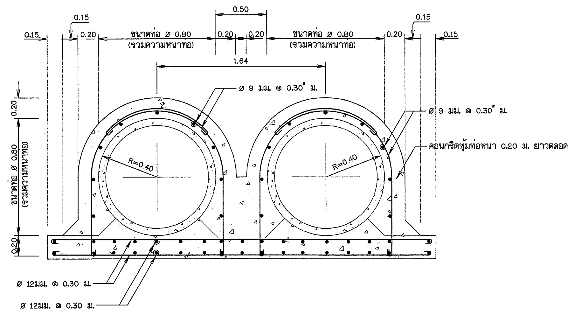
รูปตัด จ-จ มาตราส่วน 1:20
