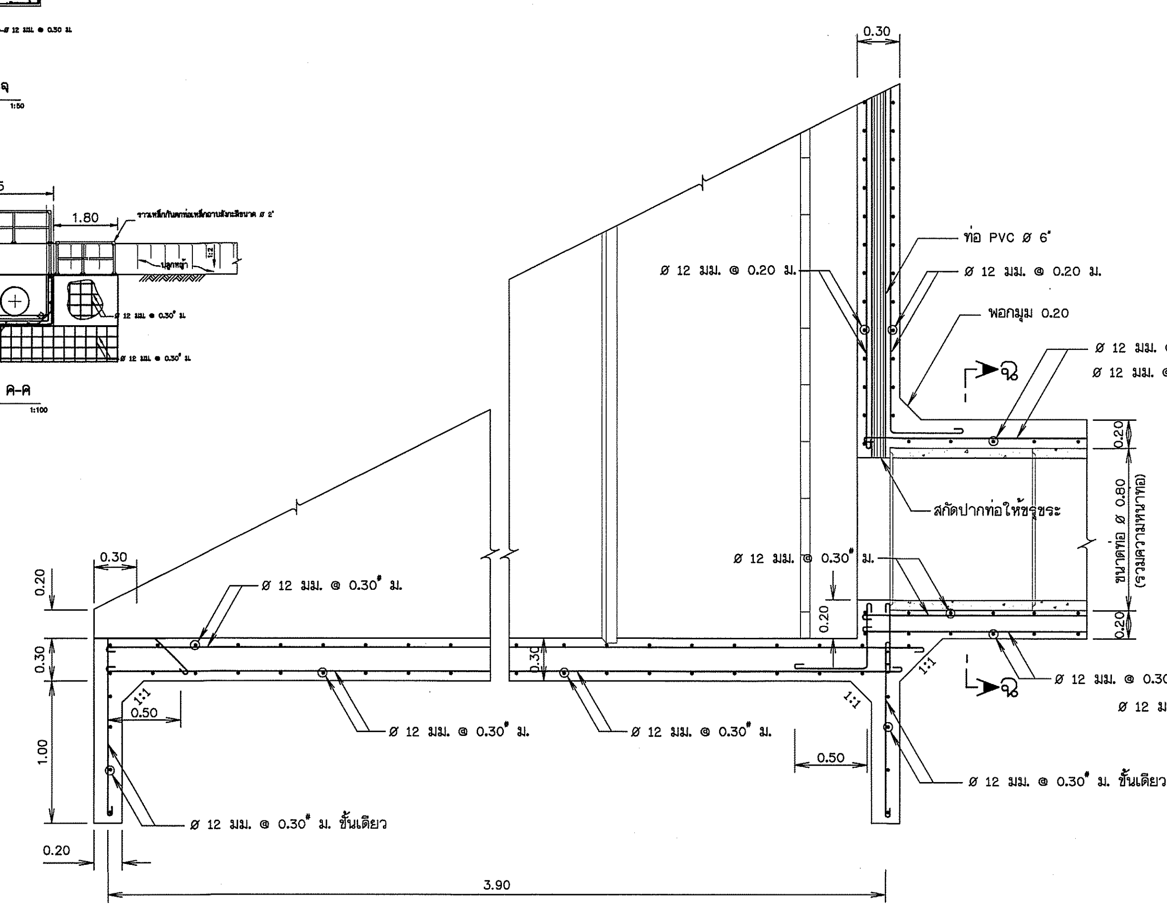
แบบขยาย 4 มาตราส่วน 1:25
