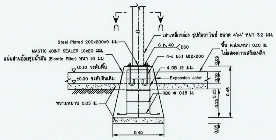
รูปขยายฐานรากโครงสร้างรับแผ่น F1 (ต่อม่อ ค.ส.ล. ห่อสำหรับประกอบติดตั้ง) ไม่แสดงมาตราส่วน
