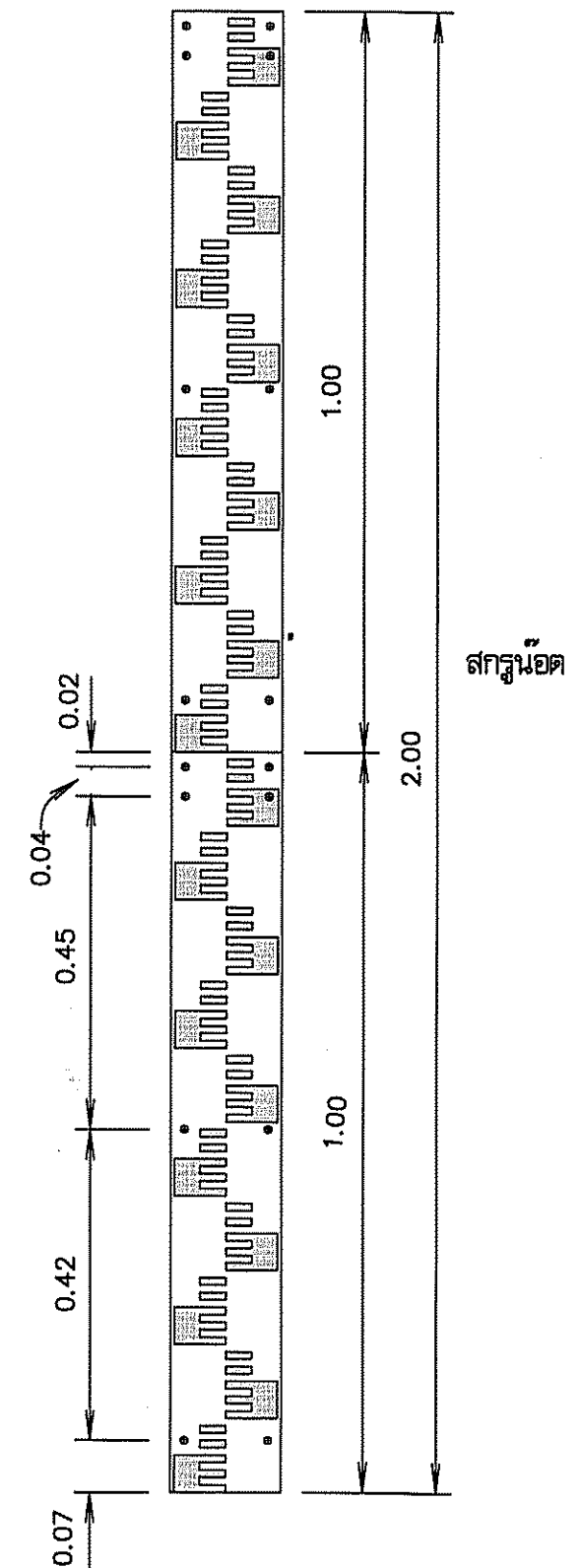
แผ่นหลักบอกค่าระดับ มาตราส่วน 1:10
