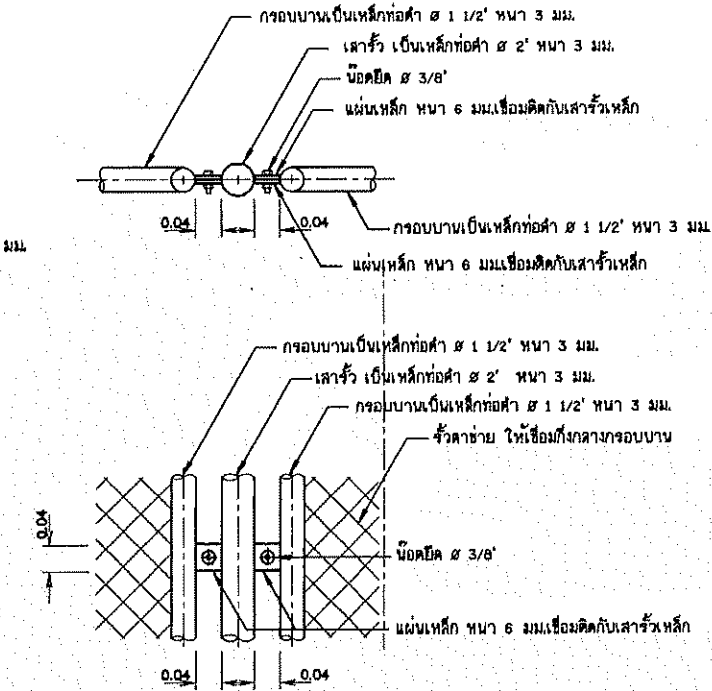
แบบขยายรายละเอียดแสดงการยึดระหว่างหัวกับเสา ไม่แสดงขนาดจั่ว
