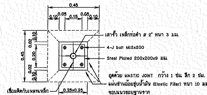
รูปตัด ข-ข ไม่แสดงขนาดจั่ว
