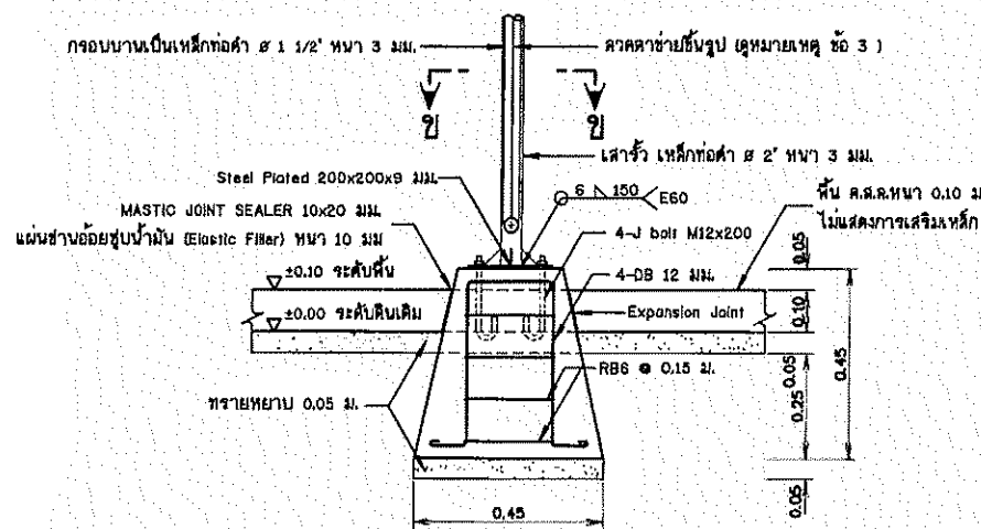
รูปขยายฐานจากโครงสร้างรับแผง F1 (คอมม. ค.ล.ค. หน้า 0.10 ม. หรือรูปอื่นใดที่ ไม่แสดงขนาดจั่ว)
