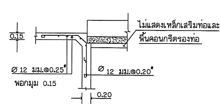
ขยาย ④ ไม่แสดงขนาดบางส่วน
