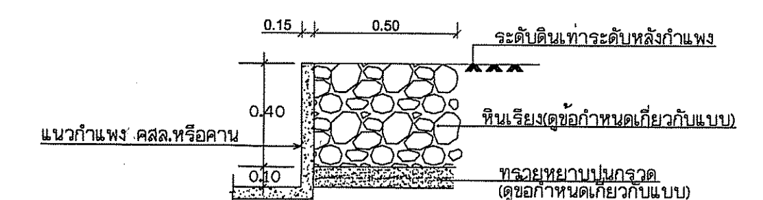
ขยายหินเรียง 1 ไม่แสดงขนาดบางส่วน
