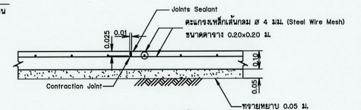
แบบขยายรอยต่อพื้น (Contraction Joint) ไม่แสดงมาตราชั่ว
