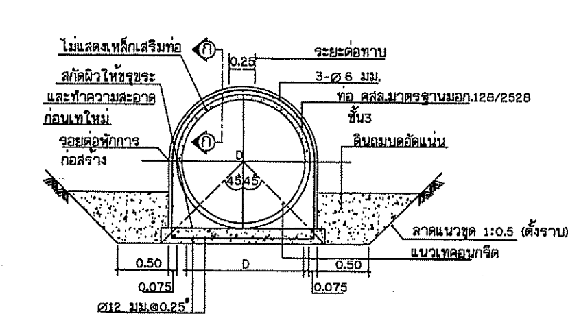
รูปตัดการวางท่อ คสล. ไม่แสดงขนาดบางส่วน
