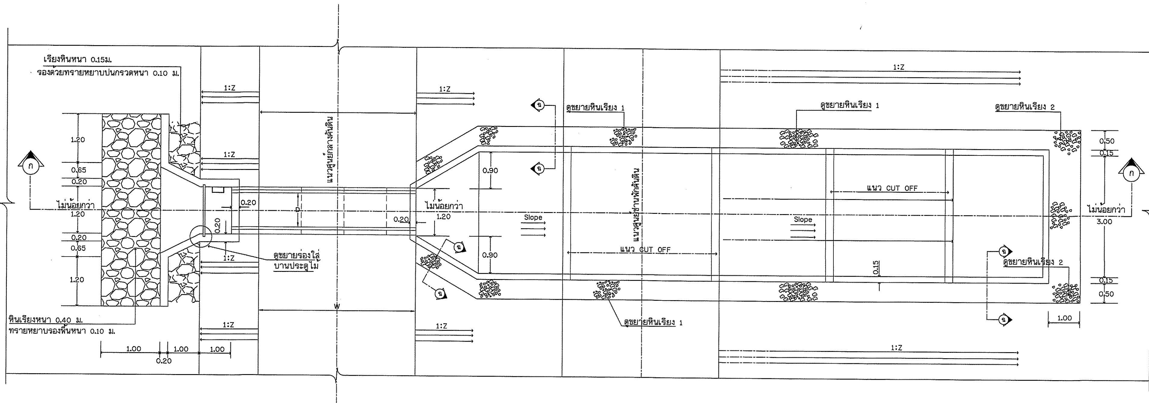
แปลนอาคารทางน้ำเข้า ไม่แสดงขนาดบางส่วน
