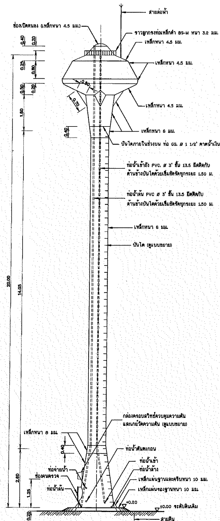
รูปด้านข้างของถังสูง แบบถังเหล็กรูปทรงแชมเปญ ไม่แสดงขนาดจากส่วน
