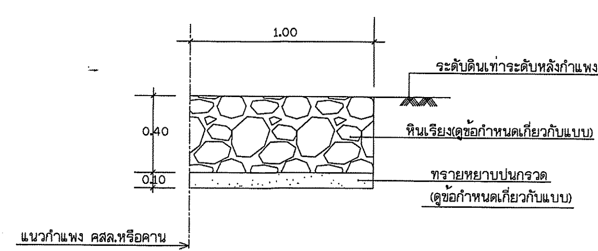
ขยาย ④ ไม่แสดงขนาดบางส่วน
