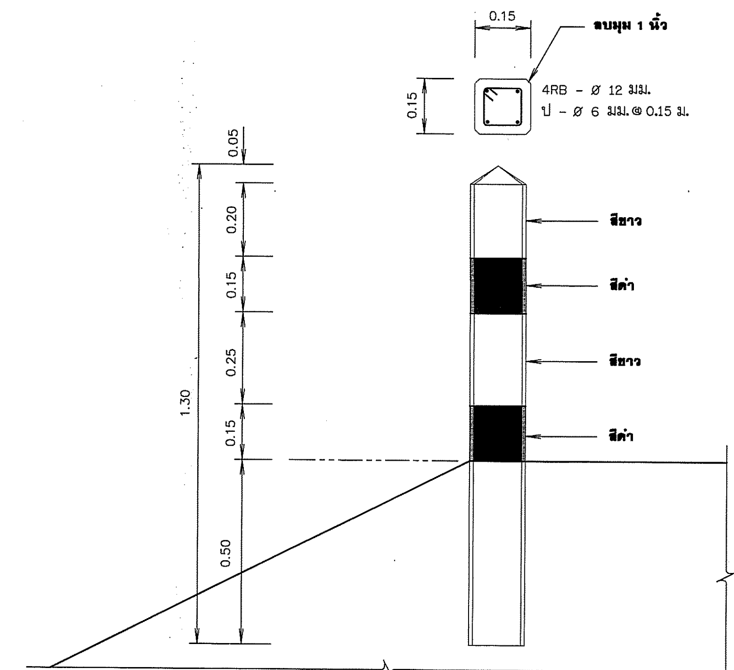
แบบขยายหลักริมคันดิน
