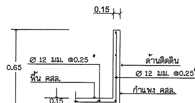
รูปตัด ก-ก (ความหนาพื้น 0.15 ม.) ไม่แสดงขนาดบางส่วน
