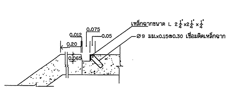
ขยายร่องไสบานประตูไม้ ไม่แสดงขนาดบางส่วน
