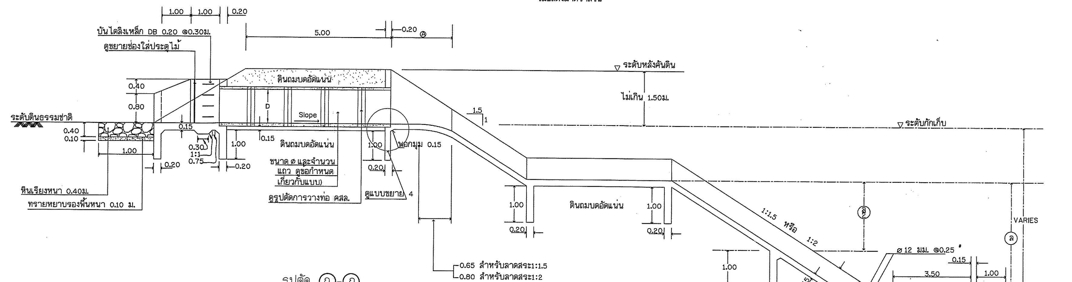
รูปตัด ก-ก ไม่แสดงขนาดบางส่วน
