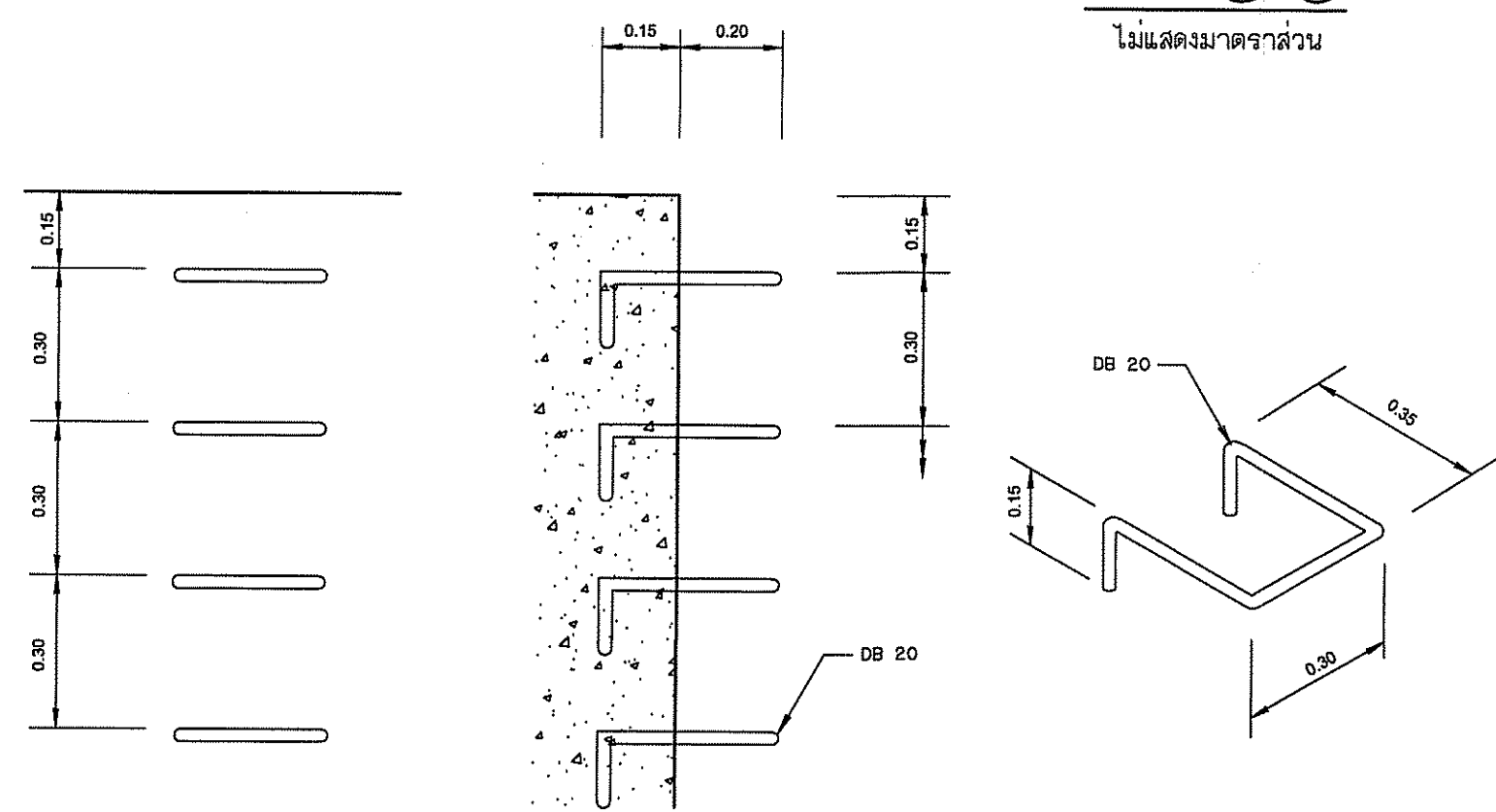
รูปขยายบันไดลิง ไม่แสดงขนาดบางส่วน
