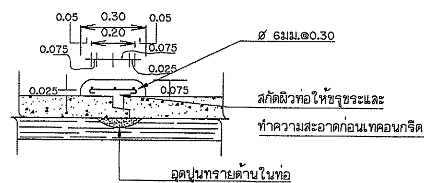
รูปตัด ก-ก ไม่แสดงขนาดบางส่วน
