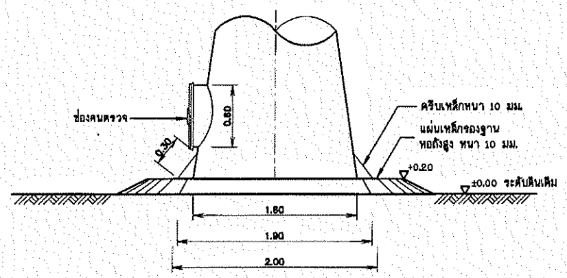
แบบขยายแมนโฮลล่างหอดึงสูง ไม่แสดงขนาดบางส่วน
