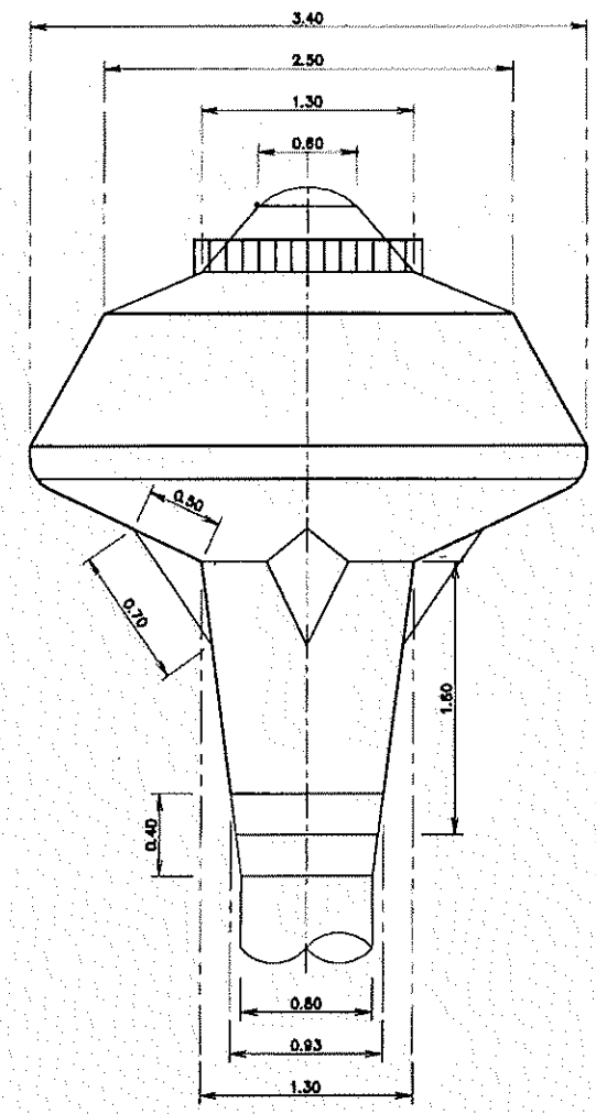
แบบขยายแมนโฮลบนหอดึงสูง ไม่แสดงขนาดบางส่วน
