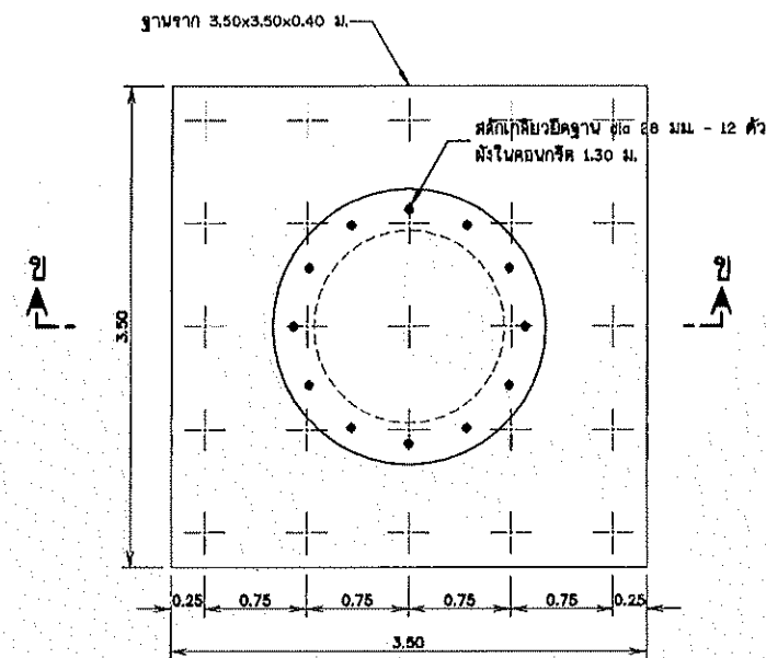
แปลน ฐานรากให้อ่างสูง (แบบเสาเข็ม)
