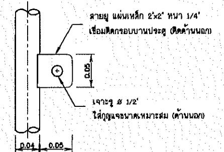
แบบขยายสายมู่ ไม่แสดงขนาดจั่ว
