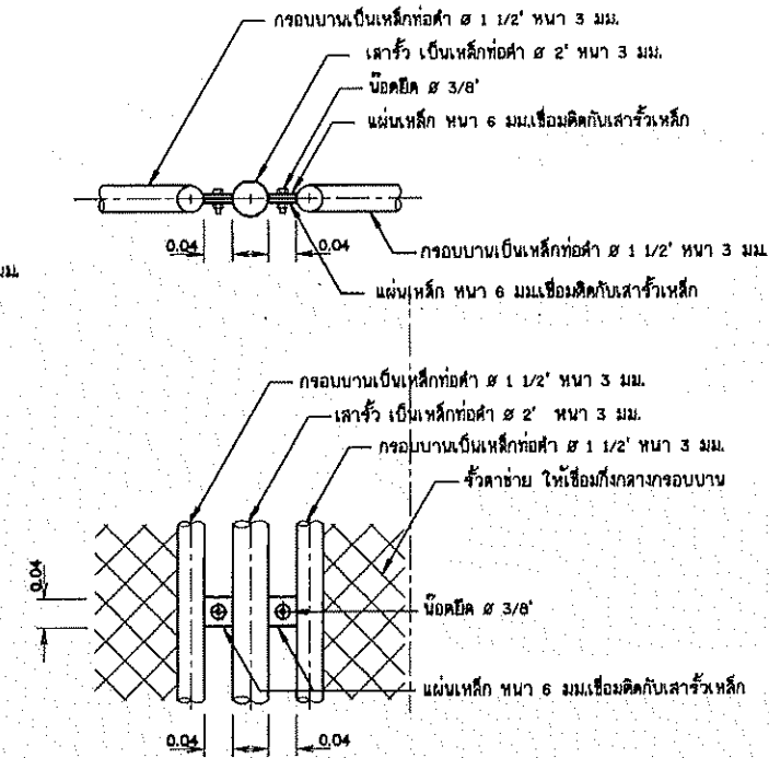
แบบขยายรายละเอียดแสดงการยึดระหว่างหัวกับเสา ไม่แสดงขนาดจั่ว
