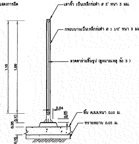
รูปตัด ก-ก ไม่แสดงขนาดจั่ว
