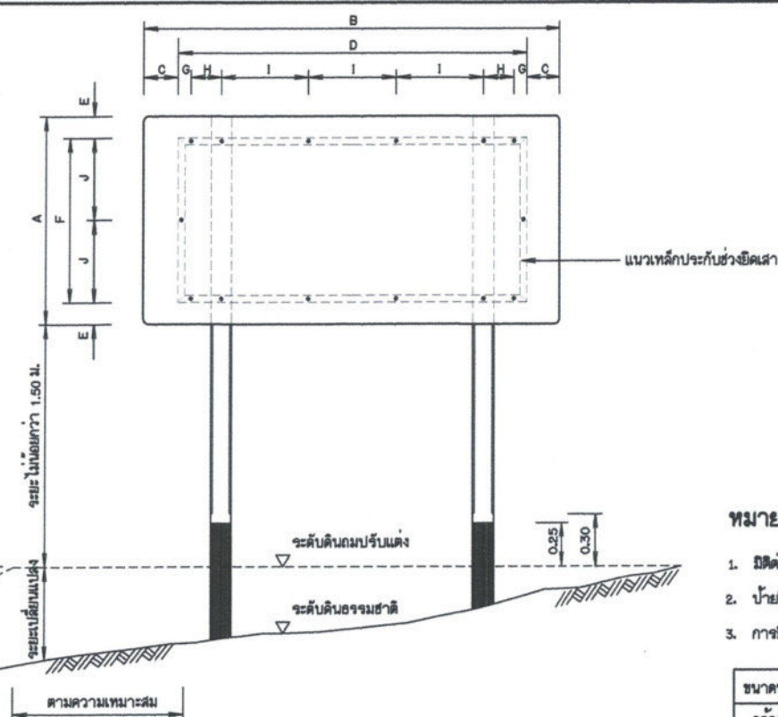
รูปแสดงการประกอบแผ่นป้าย
