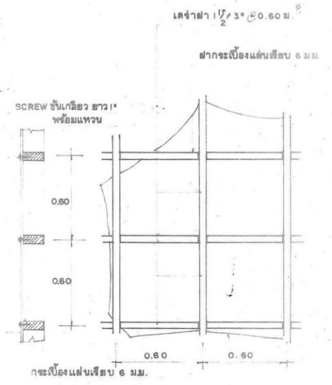
รูปขยายโครงฝ้า 1820
