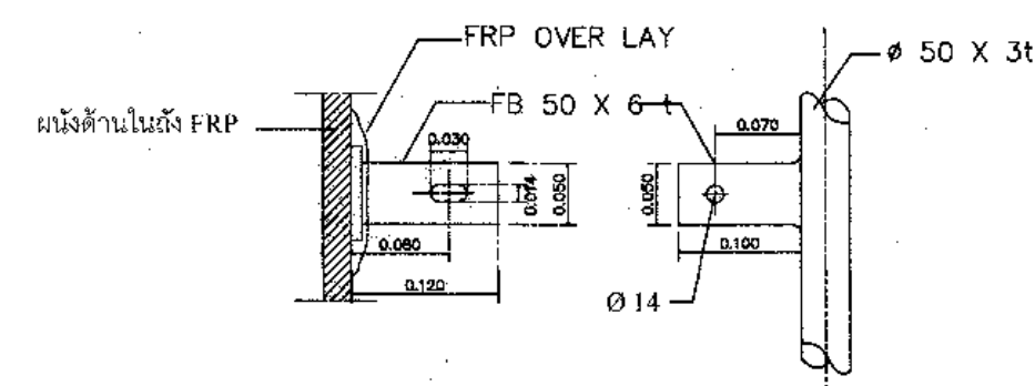
DETAIL A (ขี้ดราวก้นตึก)
