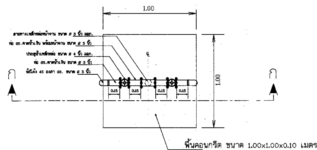
แปลน มาตราส่วน 1:20
