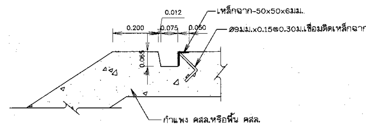
ขยายร่องใส่บานประตูไม้ มาตราส่วน 1:10
