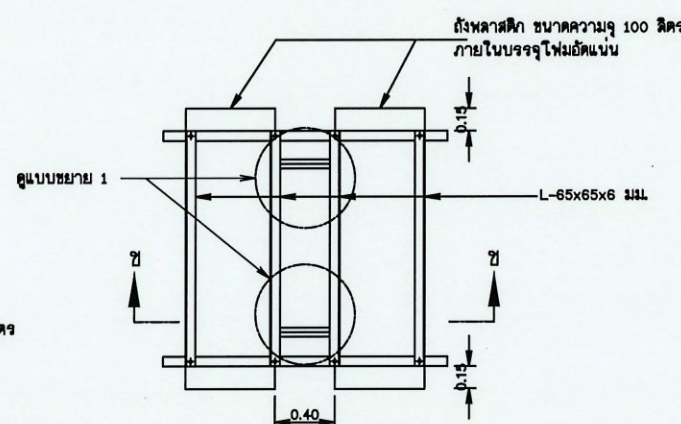
ท่อน้ำรับตัวอย่างตัวหนอน มาตราส่วน No scale
