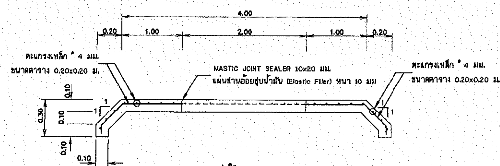
รูปตัด ค-ค
