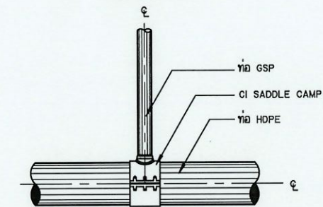
การบรรจุท่อสามทาง HDPE กับท่อ GSP แบบ CI SADDLE CLAMP (สำหรับอาคารจุดปล่อยน้ำ อาคารประจักษ์ประภาศกอน อาคารท่อระบายอากาศ กรณีท่อส่งน้ำขนาดเส้นผ่าศูนย์กลางน้อยกว่าหรือเท่ากับ 315 มม.)
