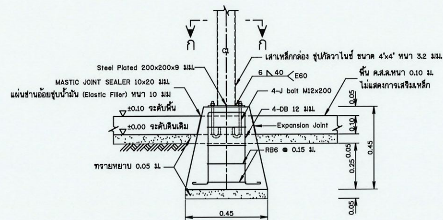
รูปขยายฐานรากโครงสร้างรับแผง F1 (ต่อม. คสล. ท่อสำหรับจุ่มพร้อมติดตั้ง) ไม่แสดงมาตราส่วน
