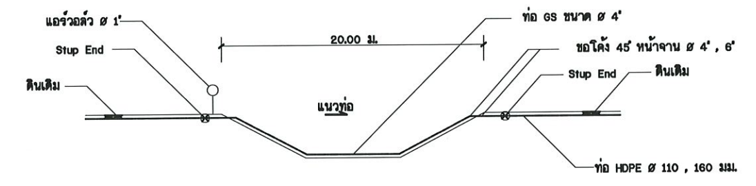
แบบขยายการวางท่อทางน้ำข้าม Wet Crossing มาตราส่วน No Scale
