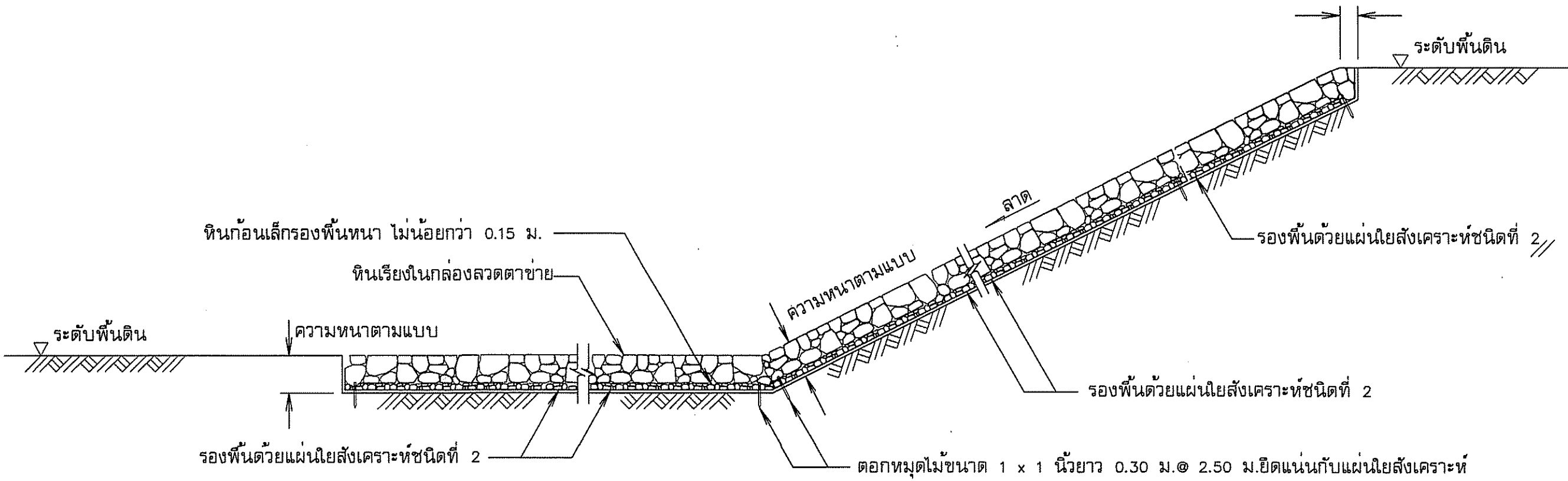
รูปตัดแสดงการเรียงหิน
