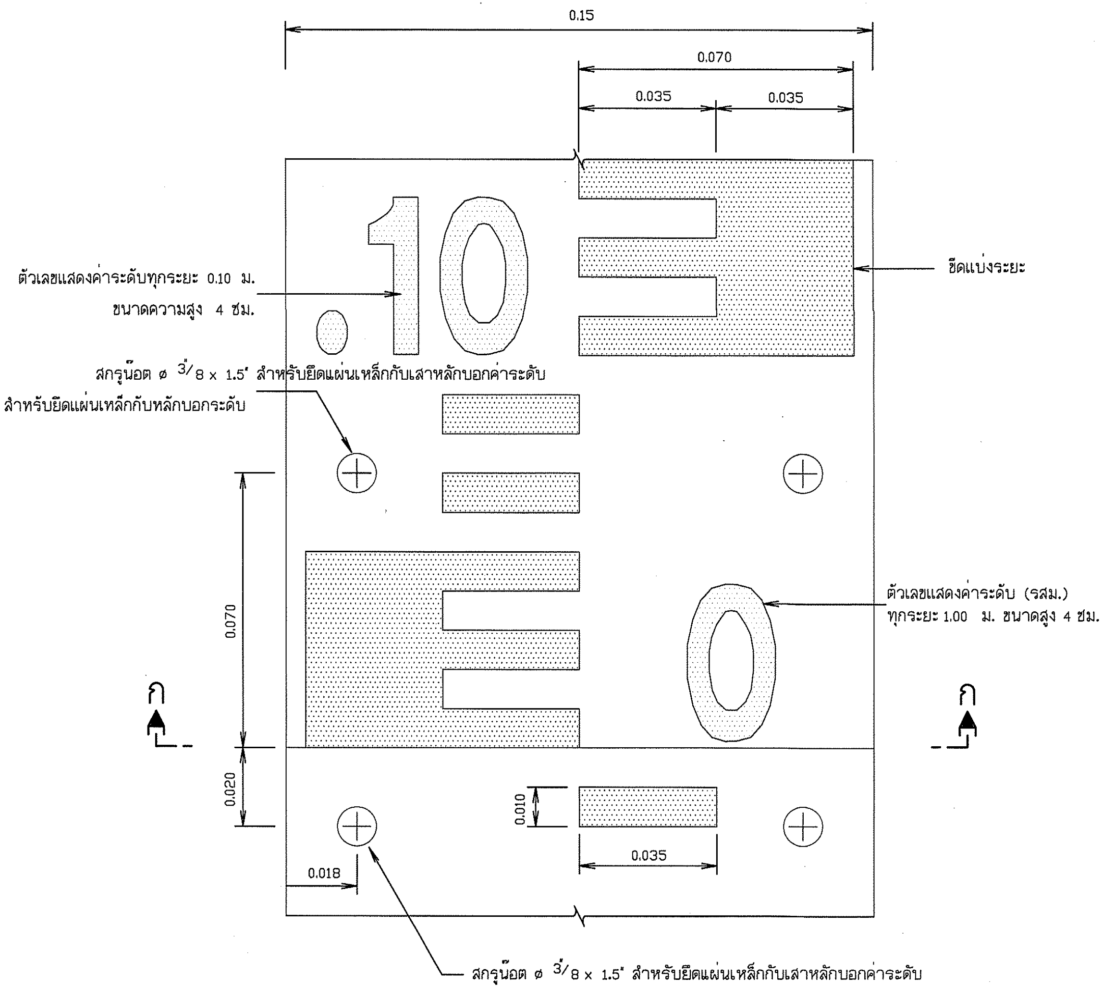
ขยายแผ่นหลักบอกค่าระดับ
