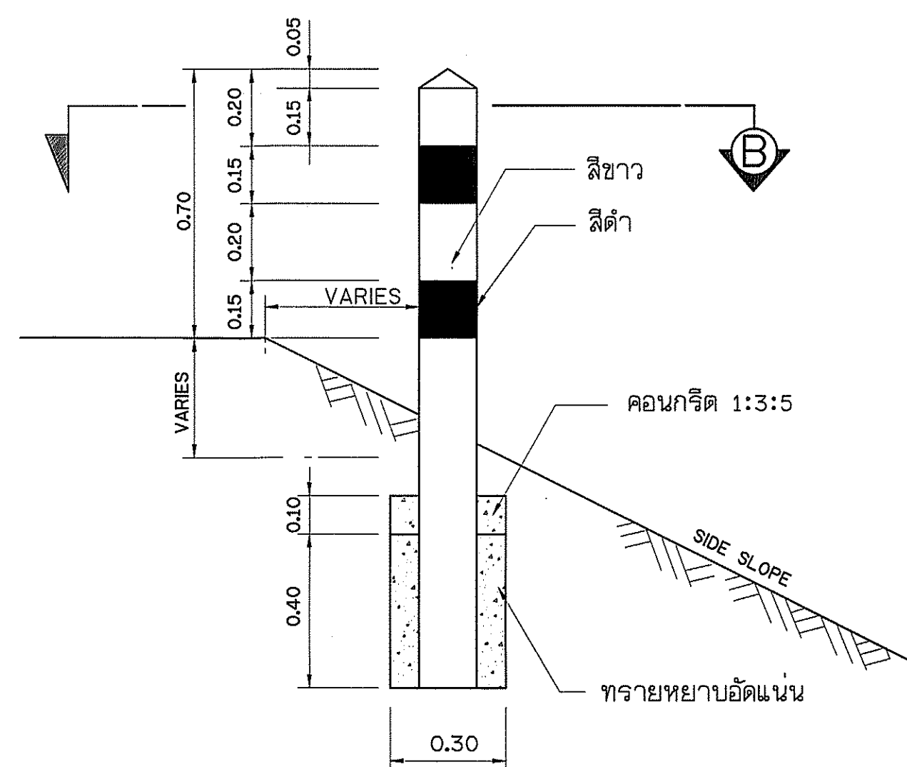
รูปขยาย ① SCALE NTS
