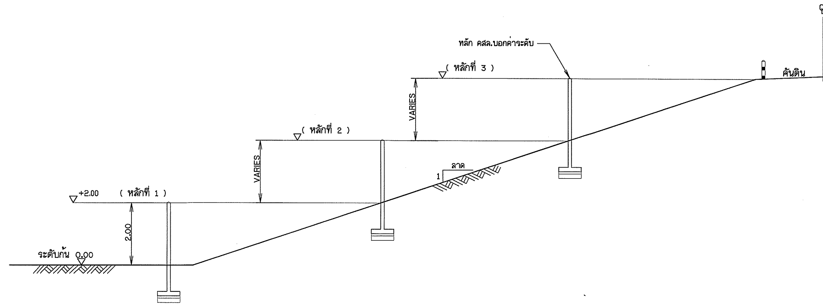
อุปดัดทั่วไปแสดงตำแหน่งหลักบอกระดับน้ำ ไม่แสดงมาตราส่วน
