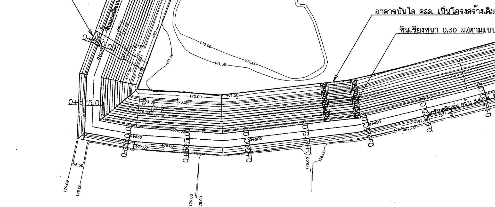
รูปแปลนโครงการ มาตรฐาน 1: 750
