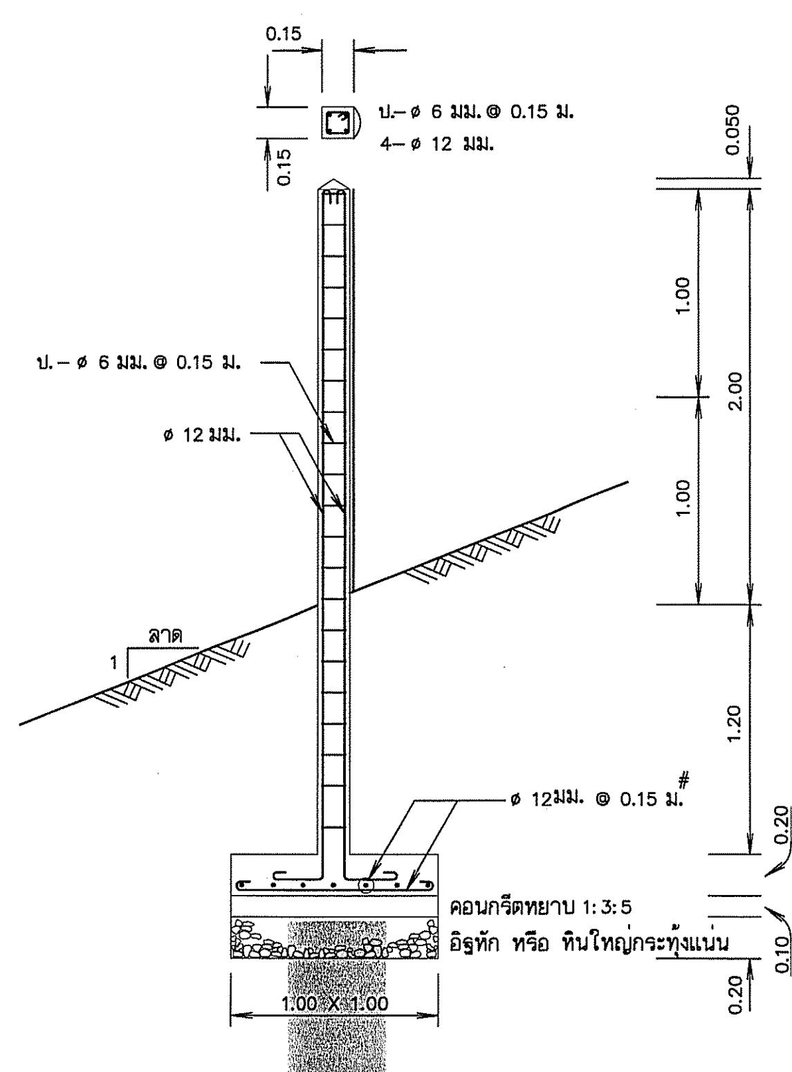
ขยายหลัก คสล.บอการค้าระดับ
