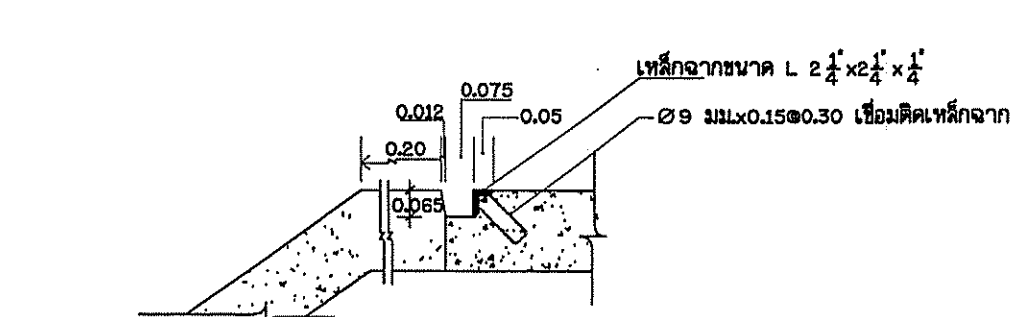
ขยายร่องใส่บานประตูไม้ ไม่แสดงมาตราส่วน
