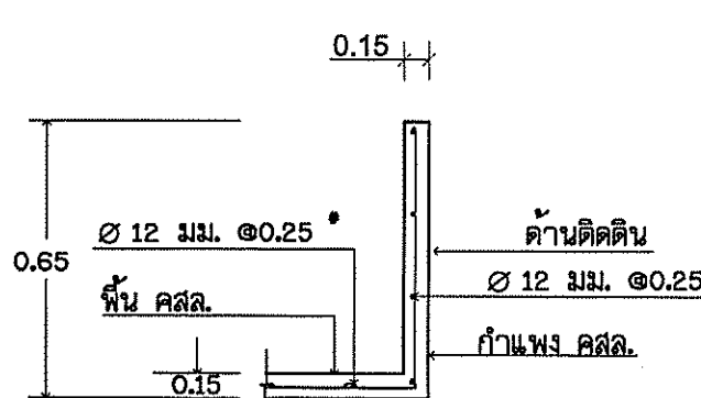
รูปตัด ๘-๘ (ความหนาพื้น 0.15 ม.) ไม่แสดงมาตราส่วน
