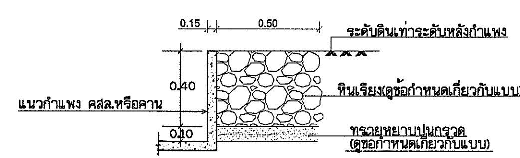
ขยายหินเรียง 1 ไม่แสดงมาตราส่วน
