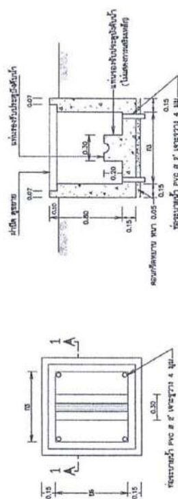
แปลนบ่อประตบบังคั้นน้ำ
