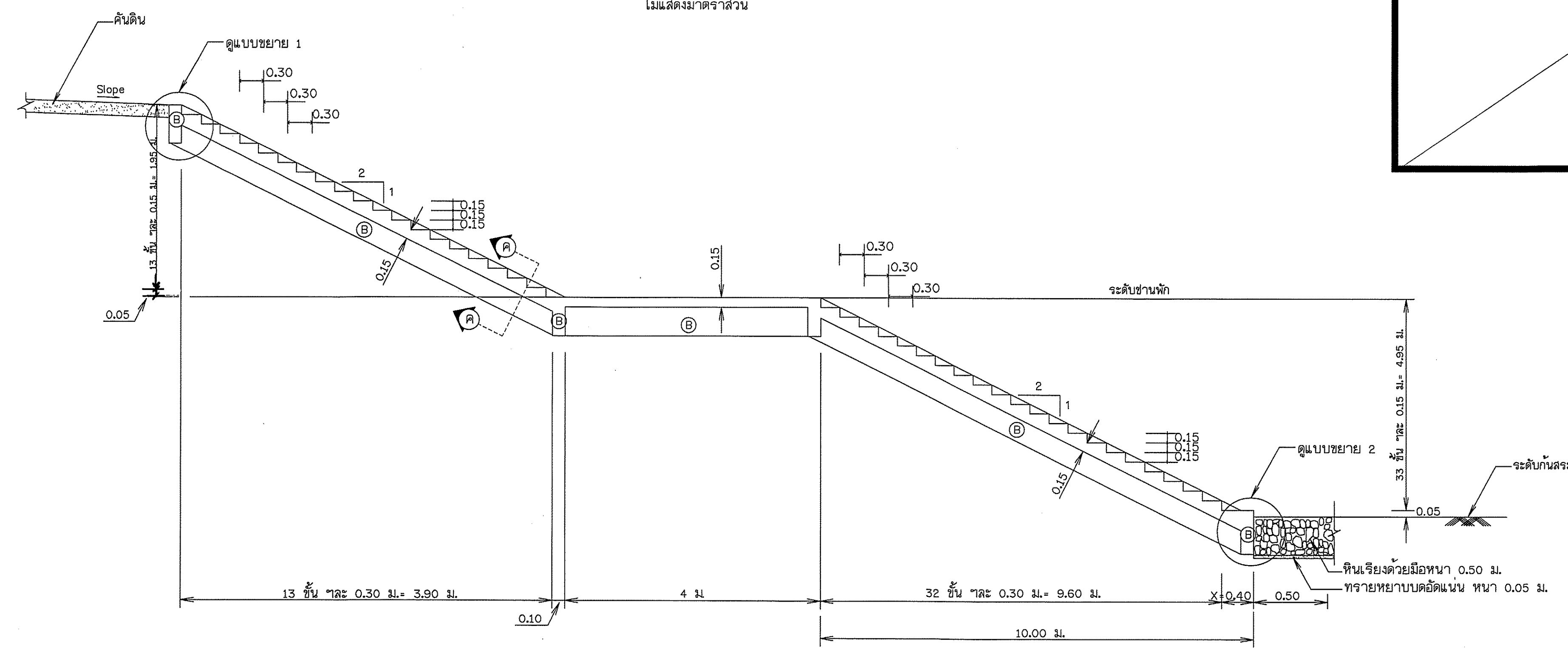
แปลนบ้านโด คสล. แบบมีชานพัก ไม่แสดงขนาดราส่วน
