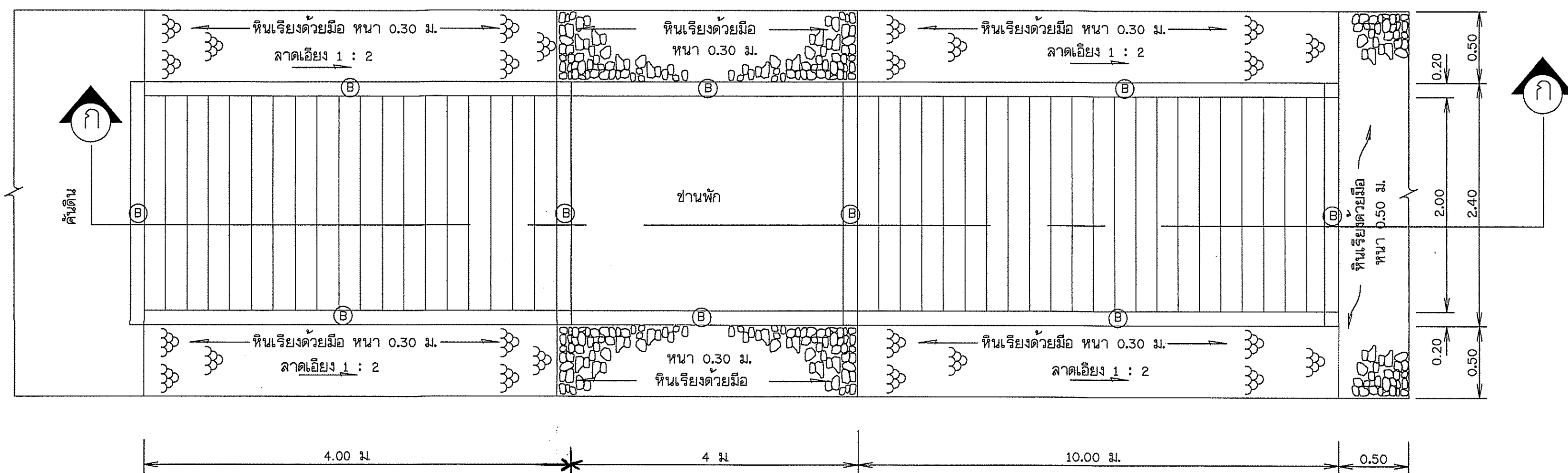
แปลนบ้านโด คสล. แบบมีชานพัก ไม่แสดงขนาดราส่วน
