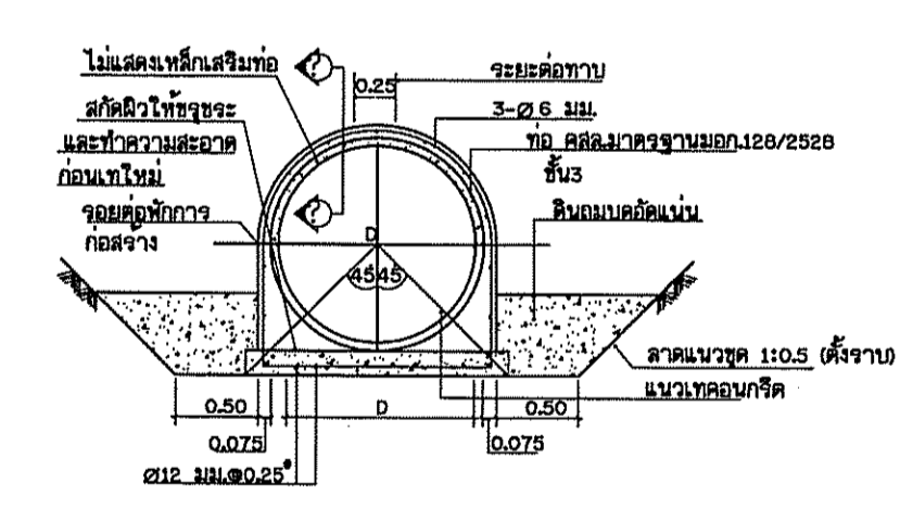
รูปตัดการวางท่อ คลล. ไม่แสดงมาตราส่วน
