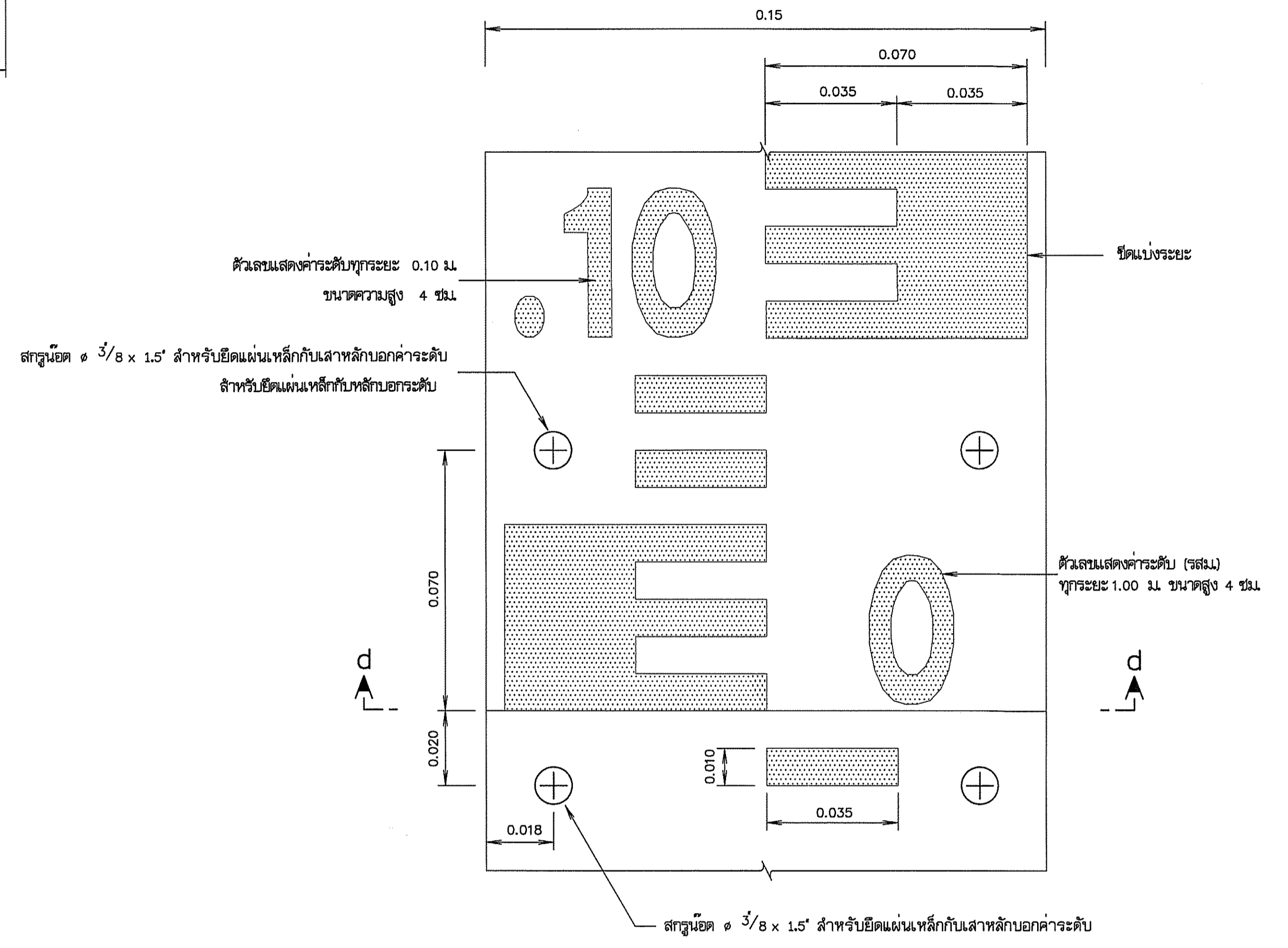
ขยายแผ่นเหล็กบ่อค่าระดับ มาตรฐาน 1:1
