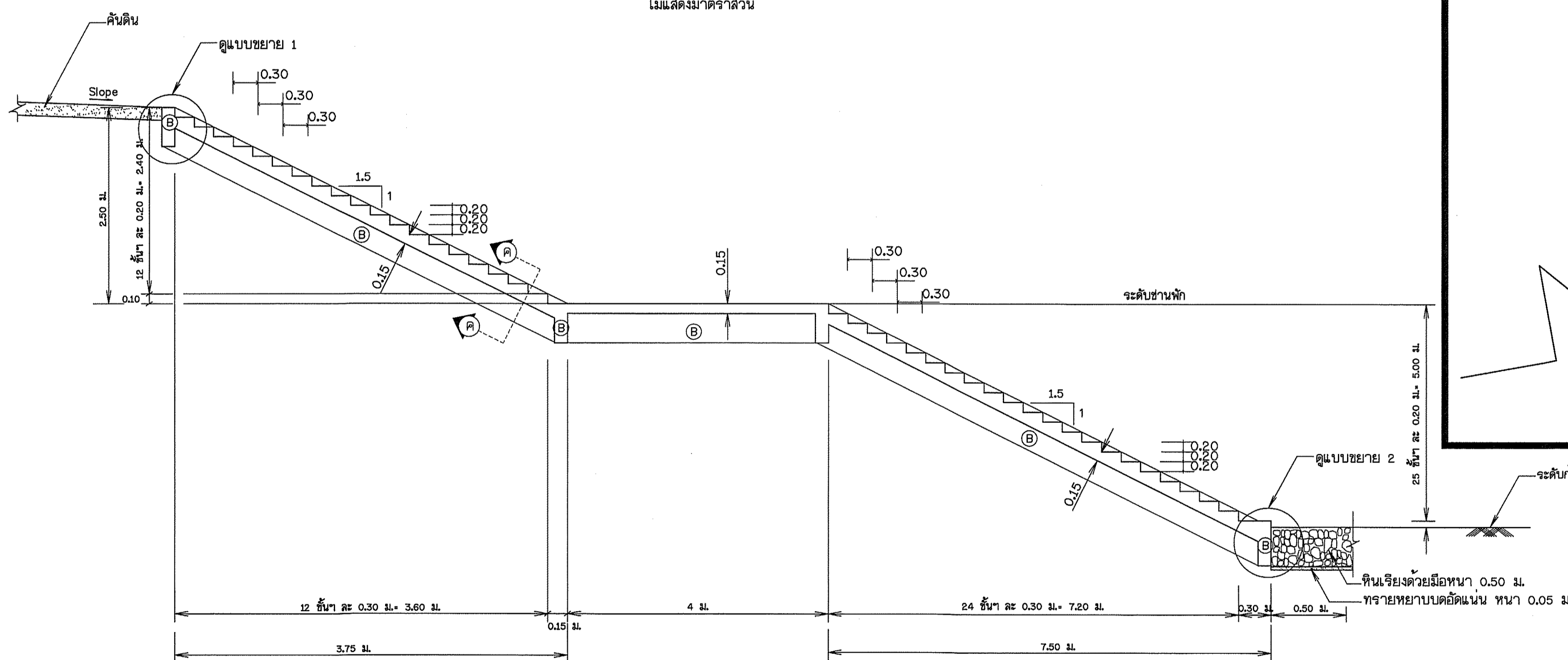
รูปตัด ก - ก
