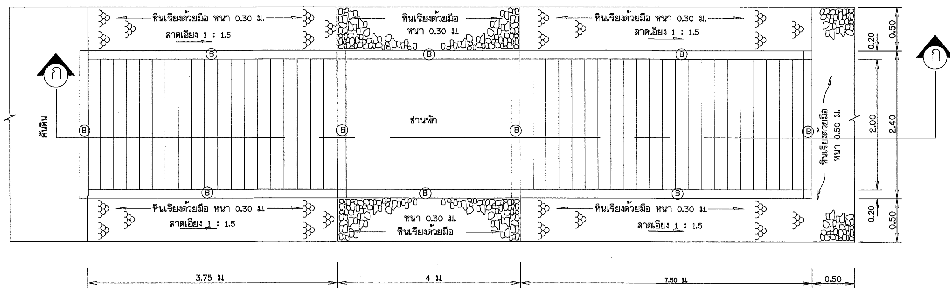
แปลนบ้านโด คสล. แบบมีชานพัก
