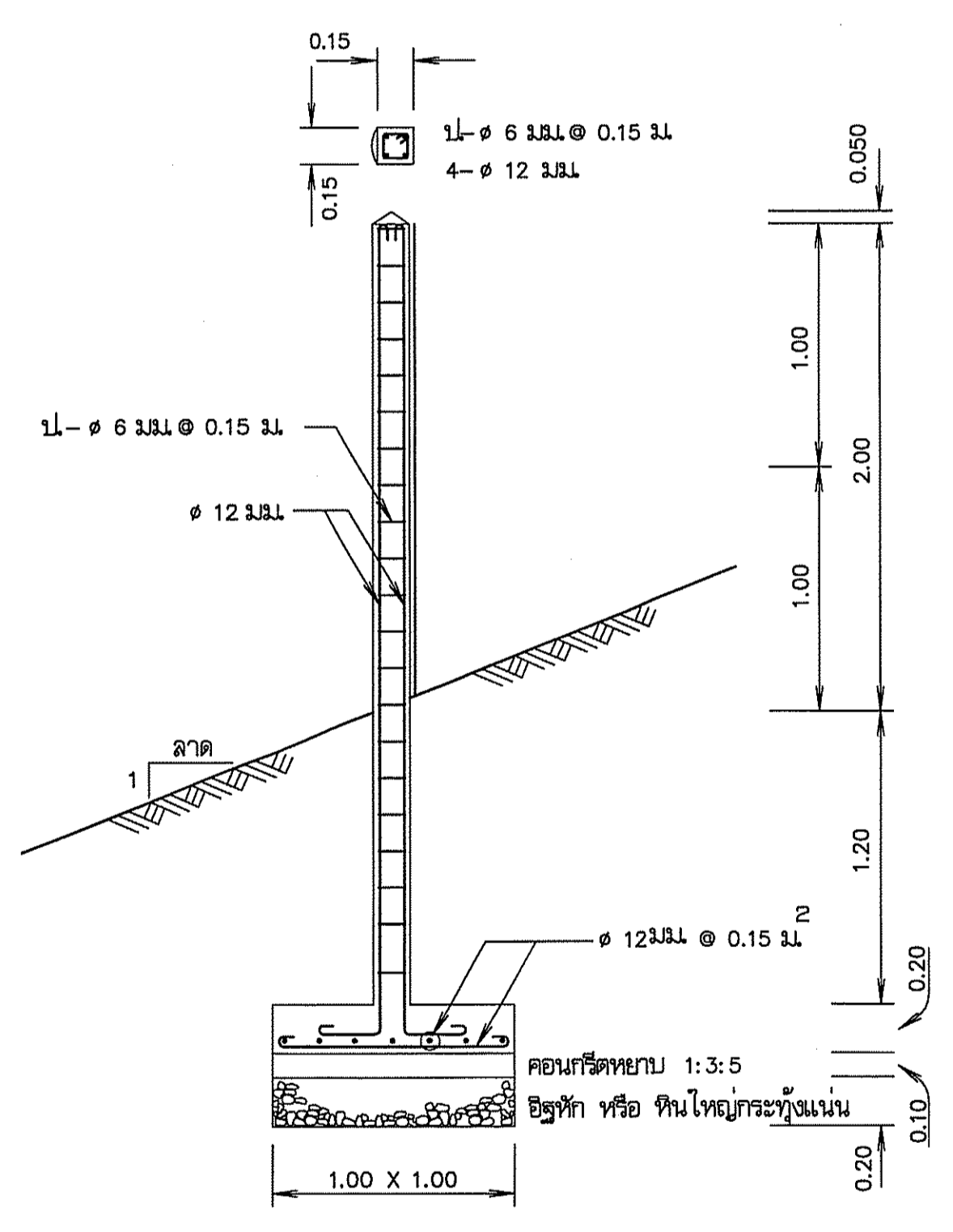
ขยายหลัก คสล.บ่อค่าระดับ มาตรฐาน 1:25
