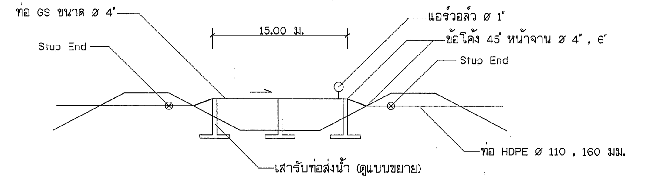
แบบขยายการวางท่อข้ามคลอง มาตรฐาน No Scale
