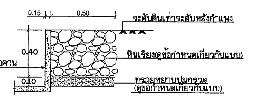
ขยายหินเรียง 1 ไม่แสดงมาตราส่วน
