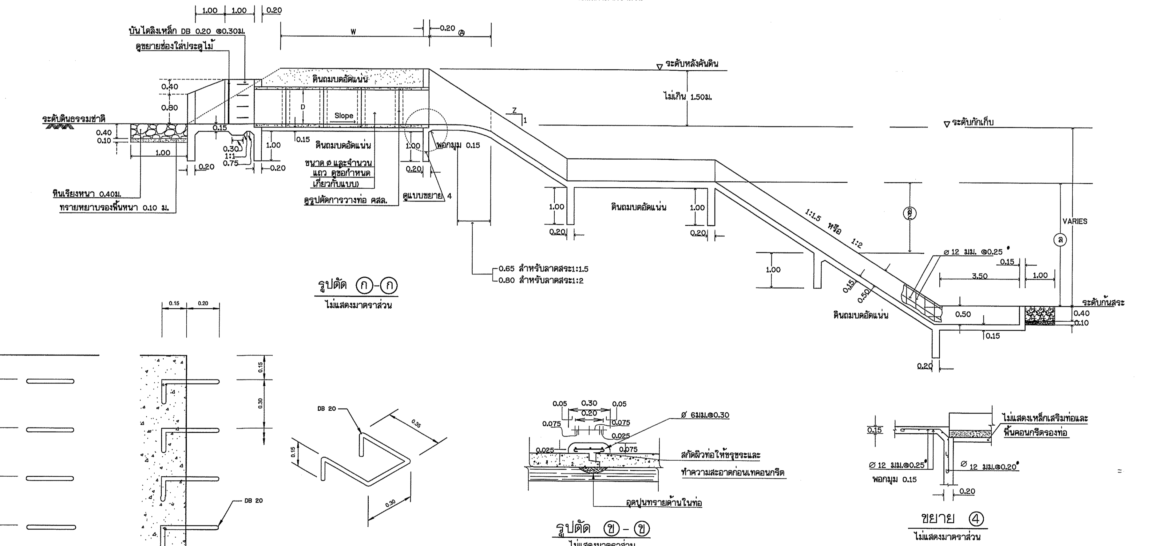
รูปขยายบันไดลิง ไม่แสดงมาตราส่วน
