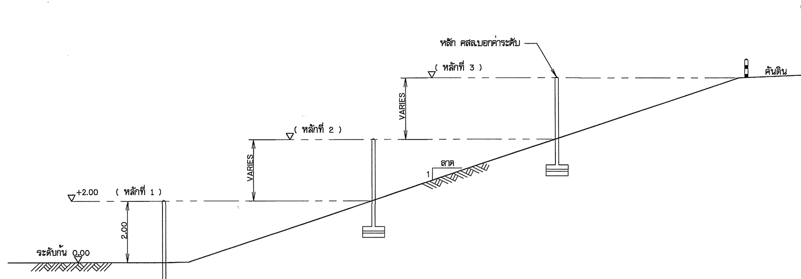
รูปตัดทั่วไปแสดงตำแหน่งหลักบ่อค่าระดับน้ำ ไม่แสดงขนาดส่วน
