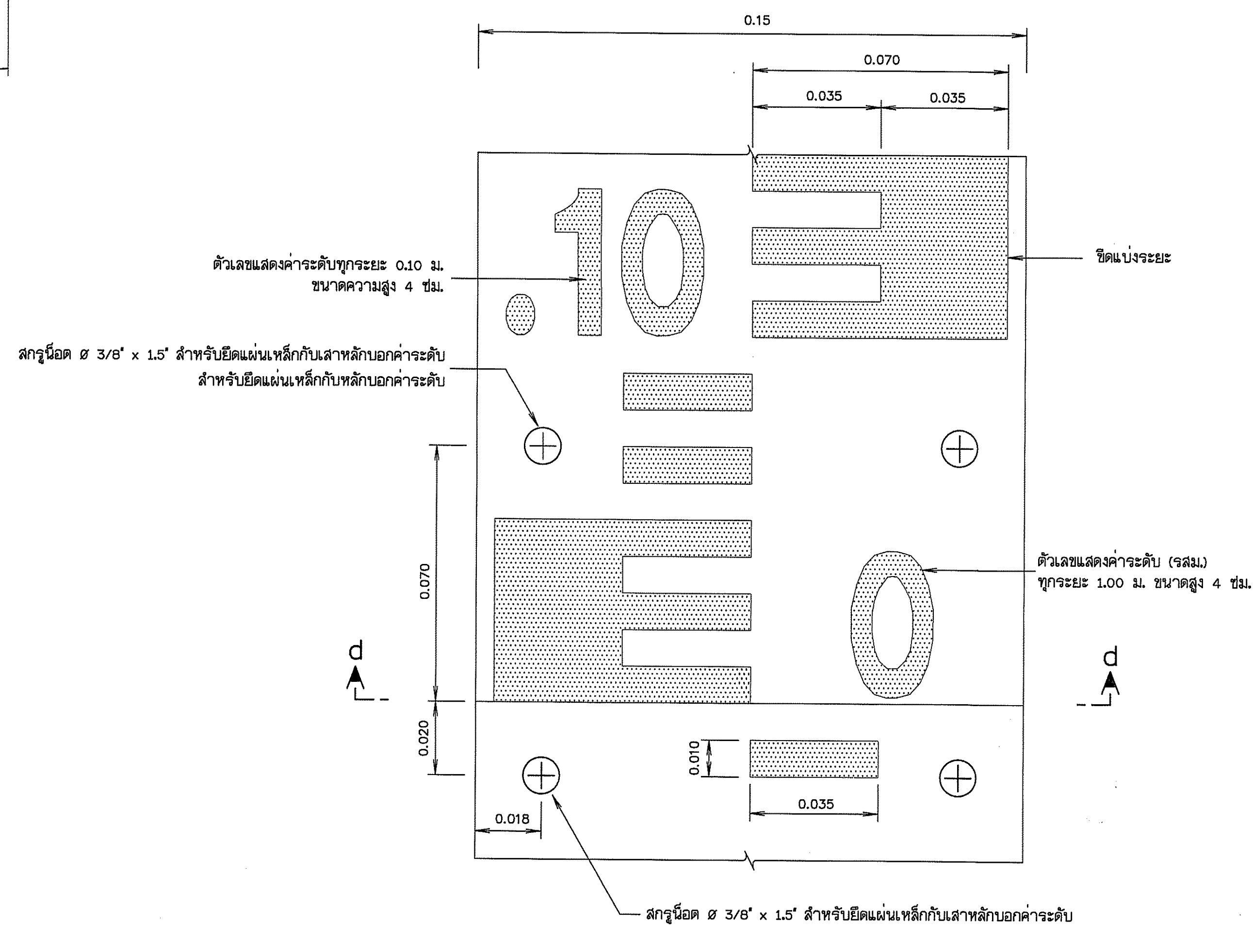
ขยายแผ่นเหล็กบอกระดับน้ำ มาตราส่วน 1:1
