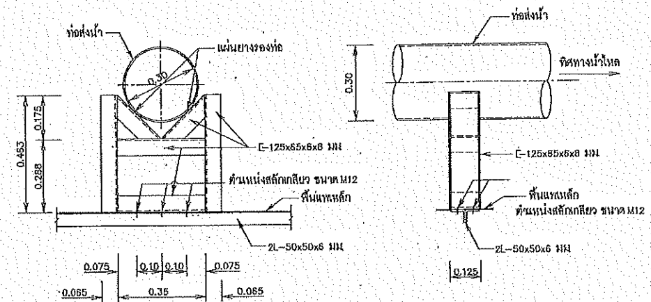
รูปขยาย SUPPORT "B" ไม่แสดงขนาดวาล์ว
