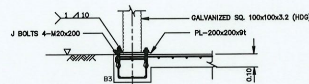
รูปตัด ก1 - ก1
