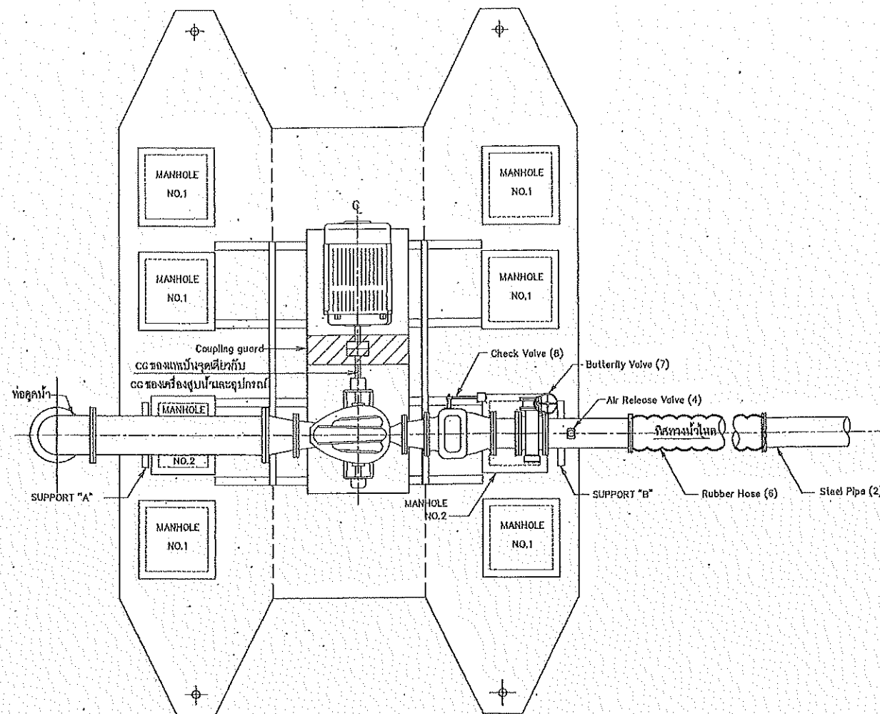
แปลนแสดงการติดตั้งเครื่องสูบน้ำ ไม่แสดงขนาดวาล์ว
