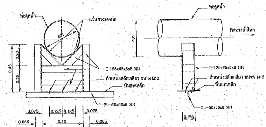
รูปขยาย SUPPORT "A" ไม่แสดงขนาดวาล์ว
