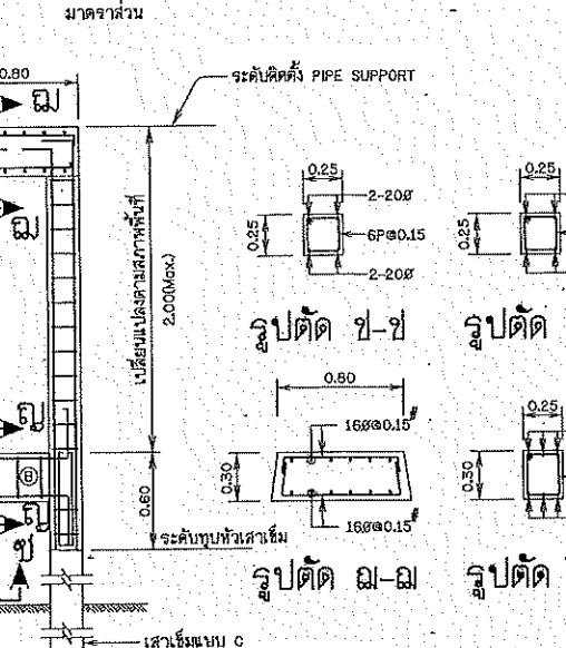
คอมม่อรับท่อแบบที่ 3, 4
