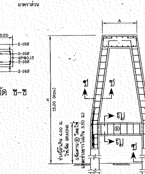
การเสริมเหล็ก คอมม่อแบบที่ 2
