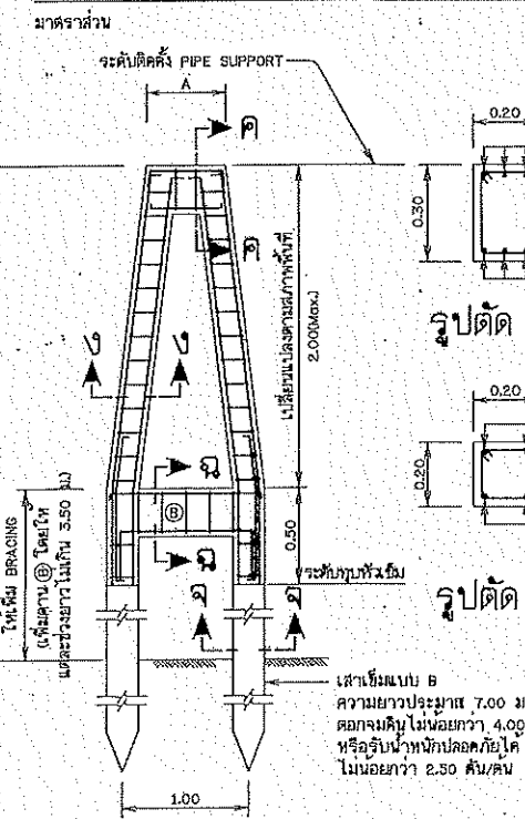
การเสริมเหล็ก คอมม่อแบบที่ 2
