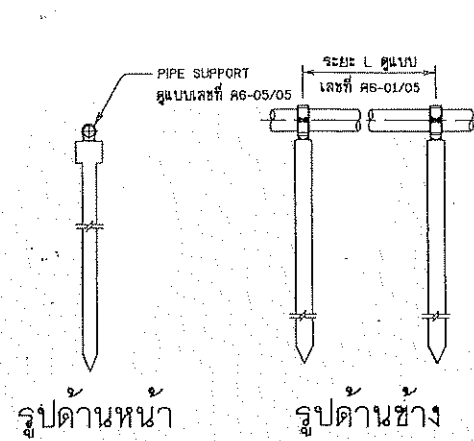
คอมม่อรับท่อแบบที่ 1
