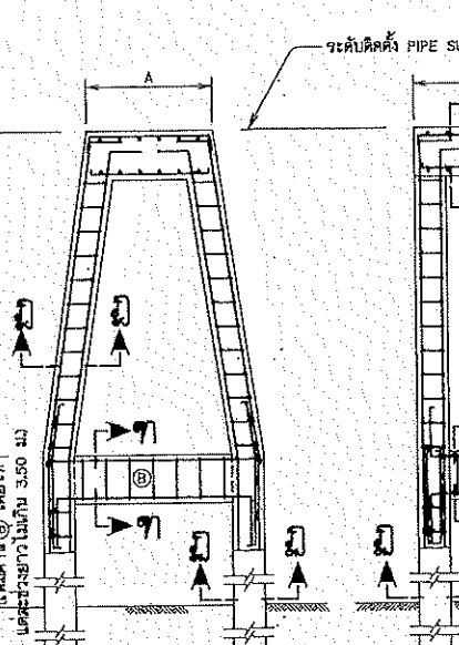
การเสริมเหล็ก คอมม่อแบบที่ 3
