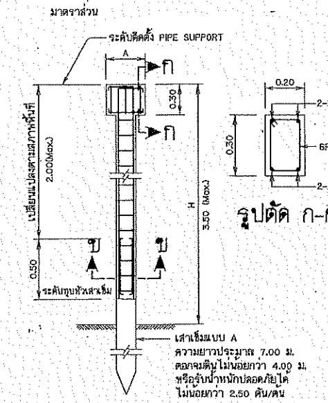
การเสริมเหล็ก คอมม่อแบบที่ 1
