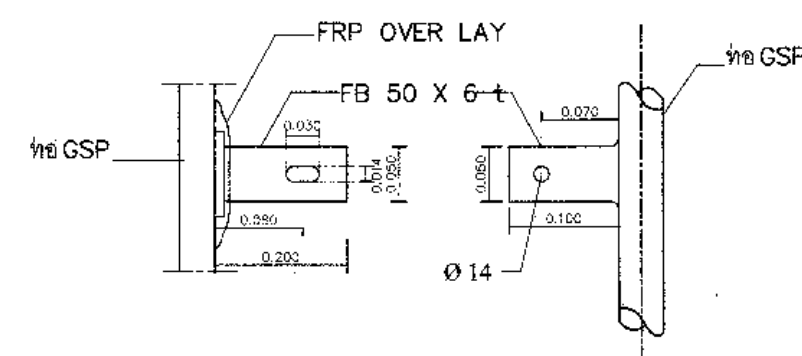
DETAIL C (ขี้นคั่นโค)
