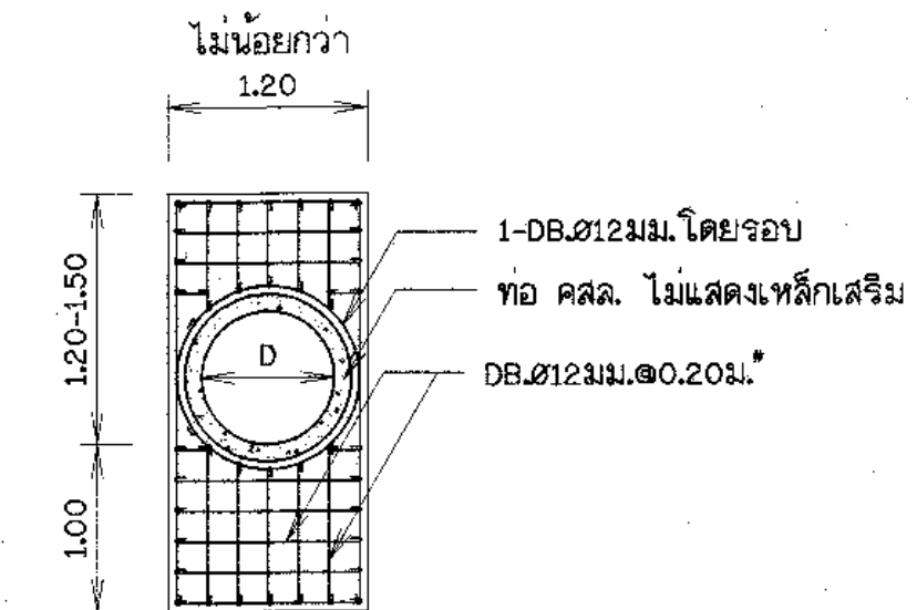
ขยายการเสริมเหล็กกำแพงปากท่อและท่าย่อ มาตรฐาน 1:50
