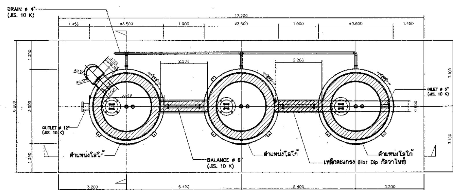
PLAN SCALE: 1:100
