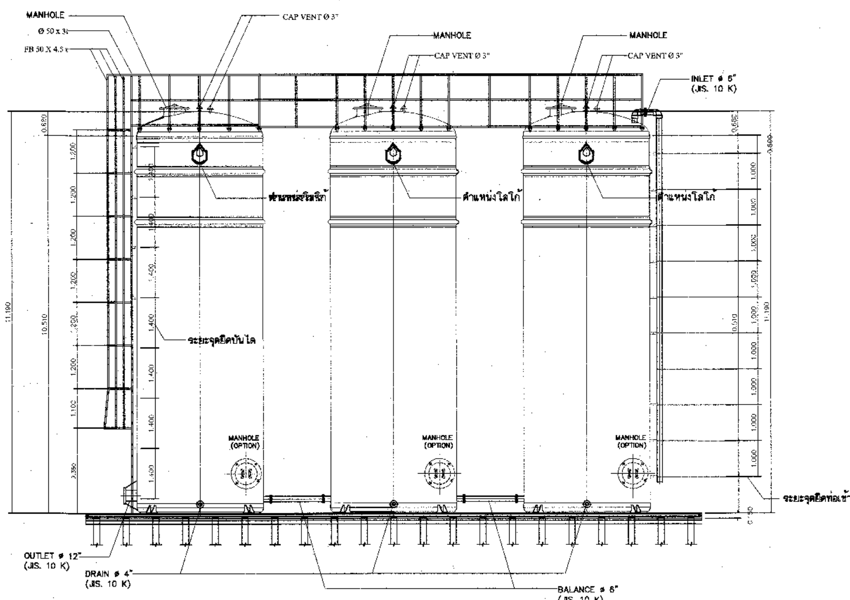
SECTION SCALE: 1:100
