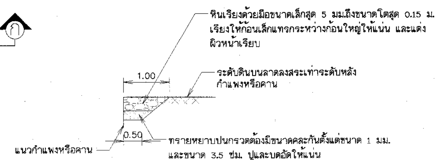
ขยายขึ้นเรียง 1
