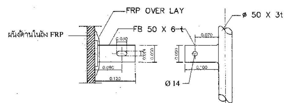
DETAIL A (ขี้นคั่นโค)
