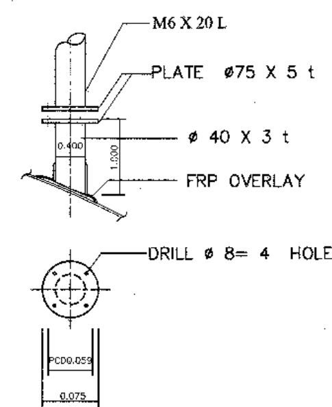
DETAIL B (ขี้นครวกันคก)
