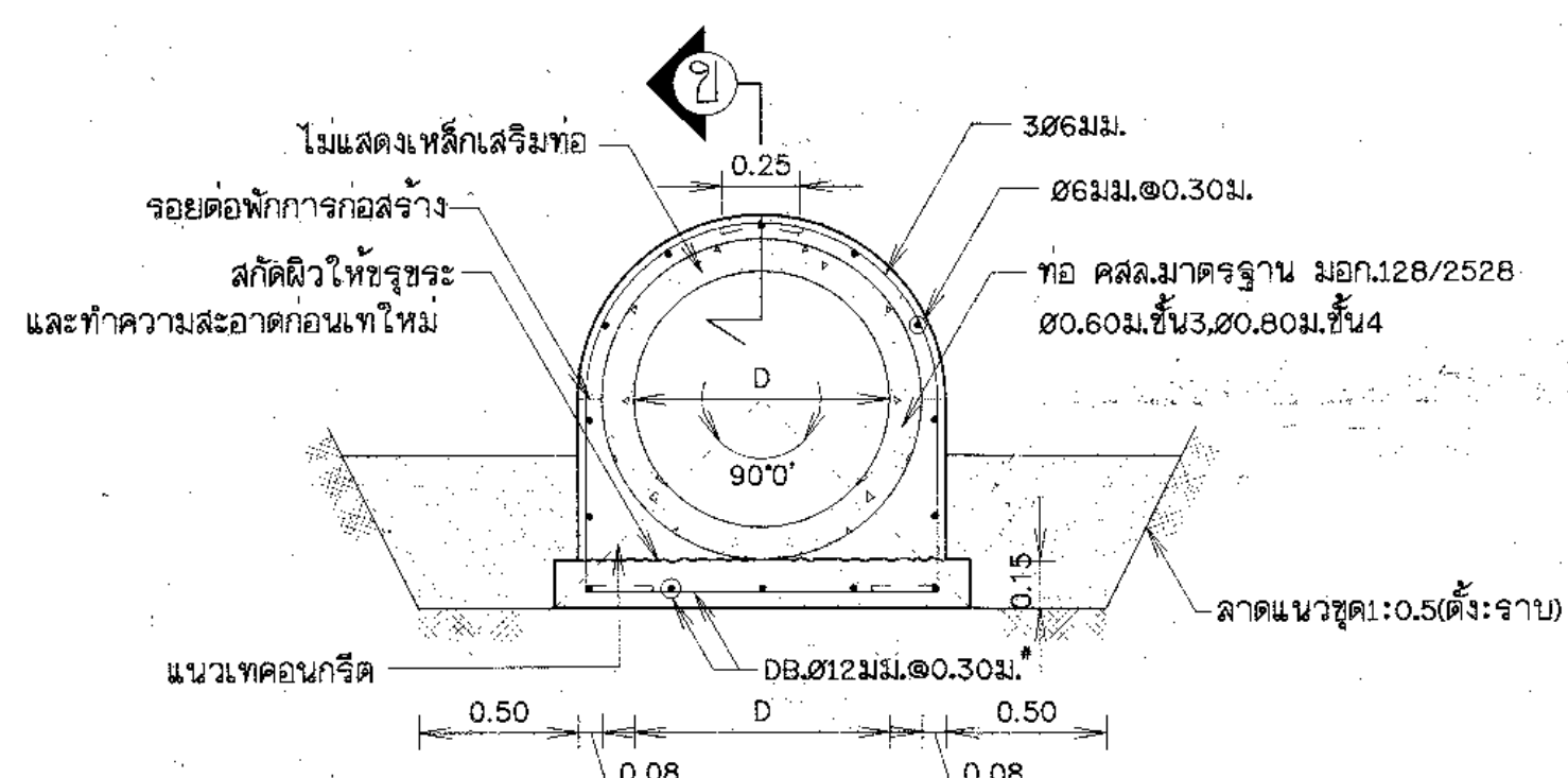
รูปตัดการวางท่อ คสล. มาตราส่วน 1:25
