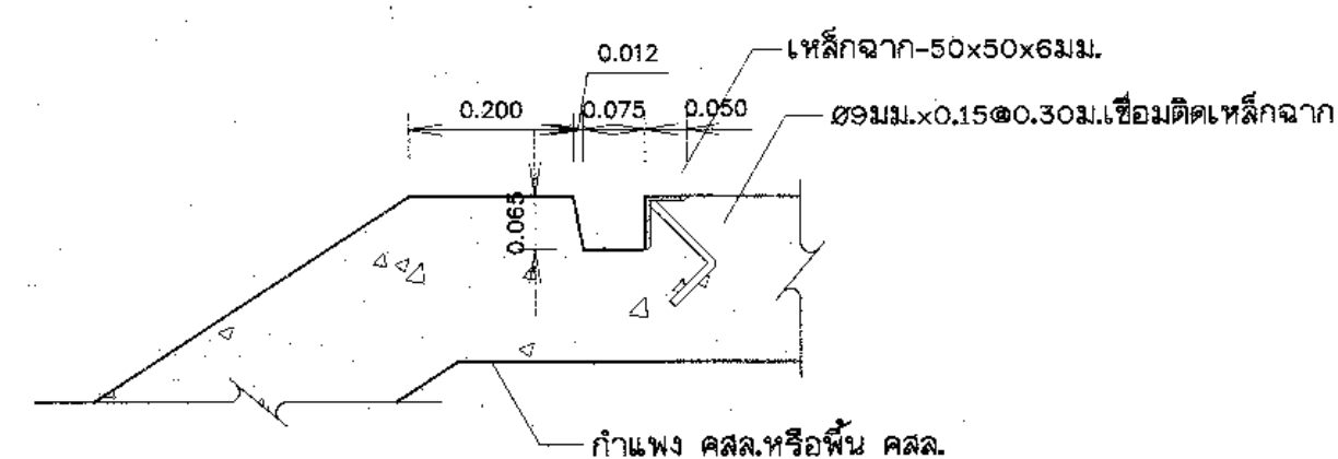
ขยายร่องไผ่บานประตูไม้
