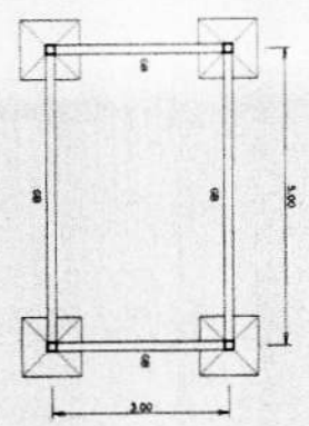
แปลนฐานราก คานคอดิน 1:150
