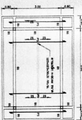
แปลนคาน พื้นหลังคา 1:150
